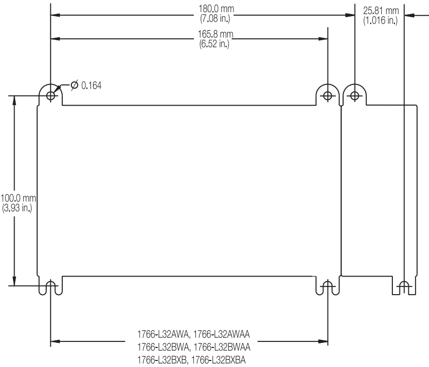
MicroLogix 1400 系统安装尺寸
