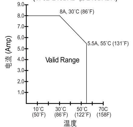
场效应晶体管 每公共端电流 (1762-L40BXB 和 L40BXBR)
