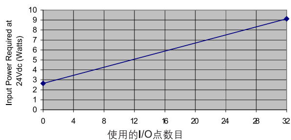
1761-L32BBB 典型功率要求
