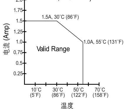
场效应晶体管 每点电流 (1762-L24BXB, L40BXB, L24BXBR, L40BXBR)
