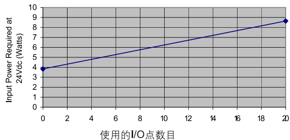
1761-L20BWB-5A典型功率要求
