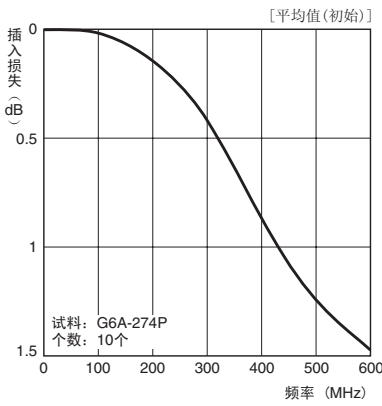
高频特性（插入损失） *1、*2
