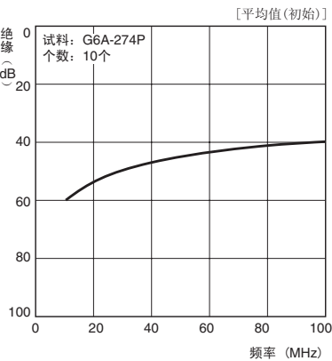
高频特性（绝缘） *1、*2
