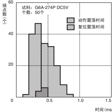
动作・复位/置位・重置震荡时间的分布 *1 G6A-274P
