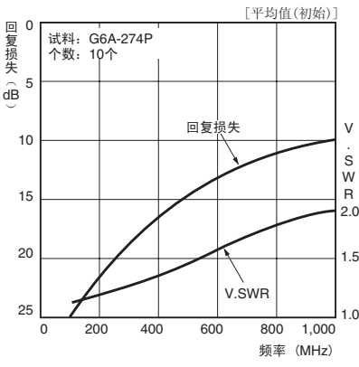
高频特性（回复损失、V.SWR） *1、*2
