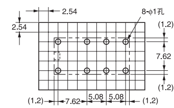
印刷基板加工尺寸 (BOTTOM VIEW) 尺寸公差±0.1mm。
