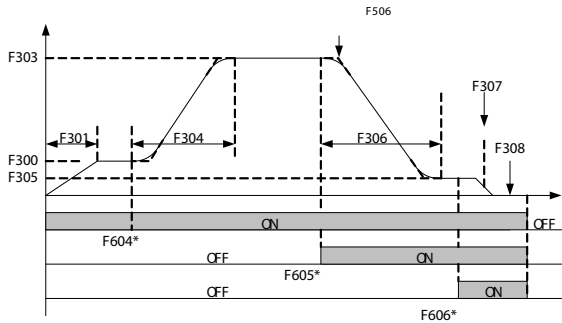
图6-4 距离控制开门曲线示意图
