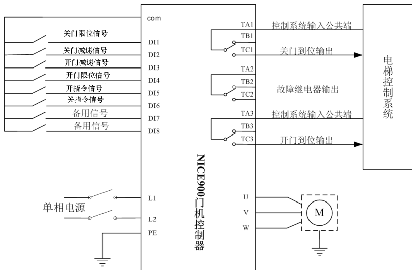
图7-4 速度控制系统典型应用接线图
