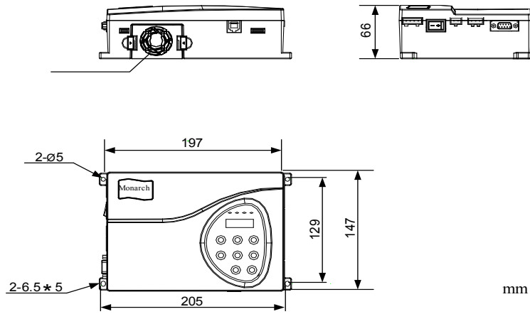
图2-3 产品外型
