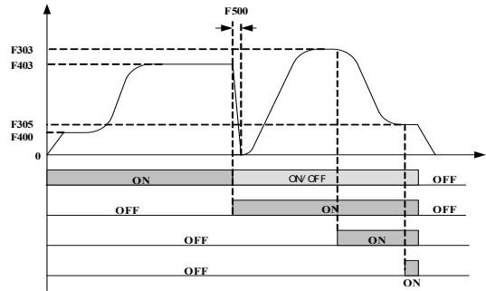
图7-8 距离控制方式遇阻运行曲线图
