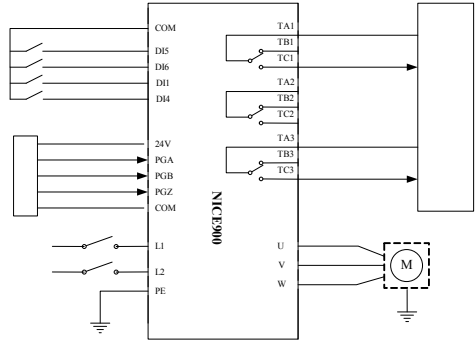
图7-6 距离控制方式（脉冲+限位开关）应用接线方式
