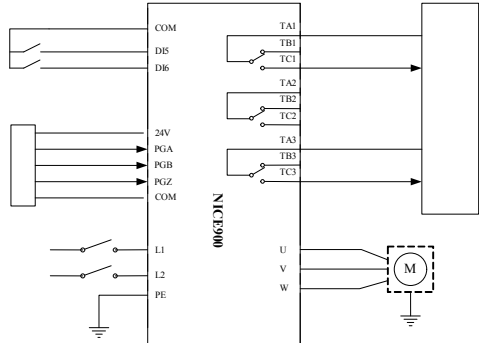
图7-7 距离控制方式（全脉冲）应用接线方式
