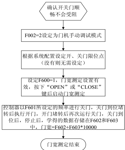
图7-3 门宽自学习
