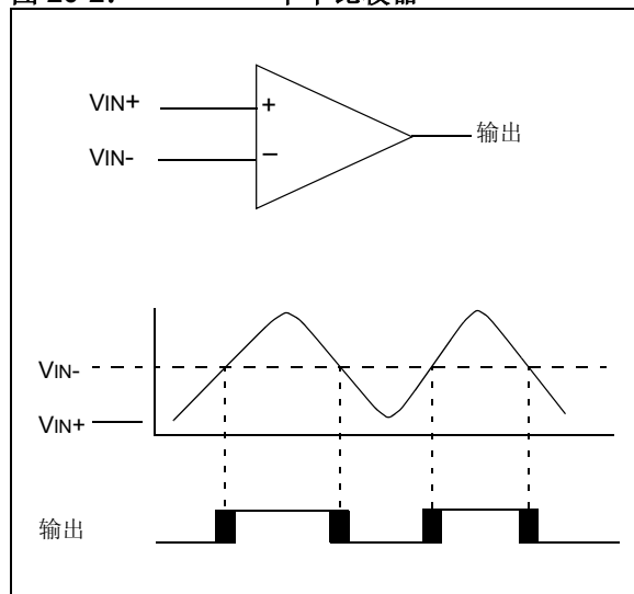
图 20-2: 单个比较器
