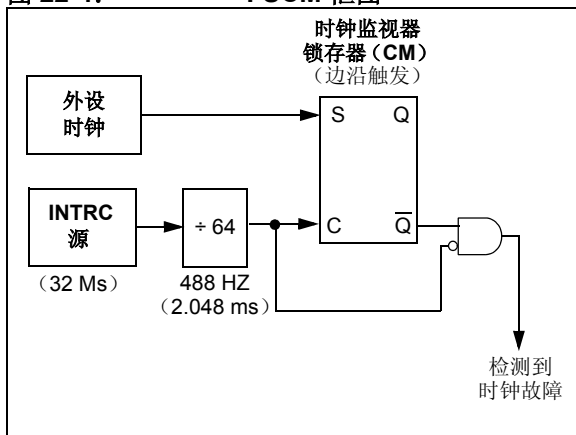
图 22-4: FSCM 框图
