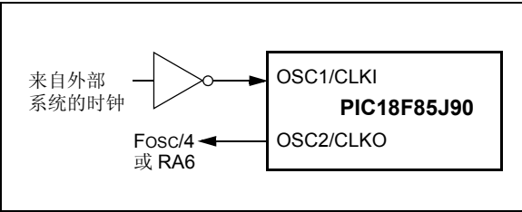
图 2-3: 外部时钟输入工作原理 (EC 配置)
