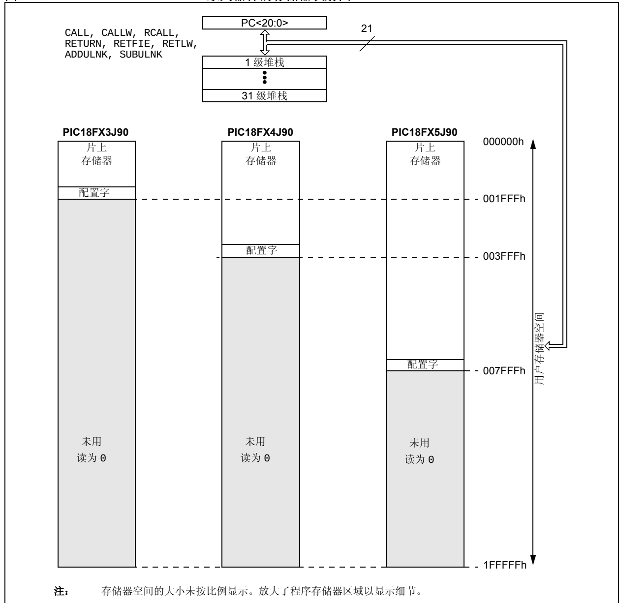
图 5-1: PIC18F85J90 系列器件的存储器映射图
