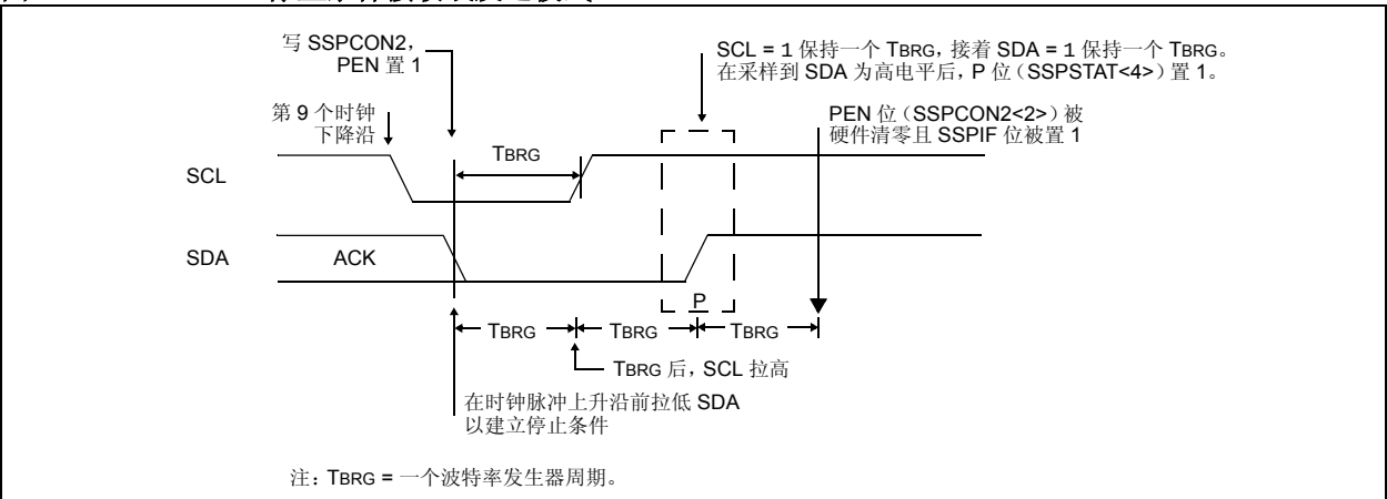
图 16-26: 停止条件接收或发送模式
