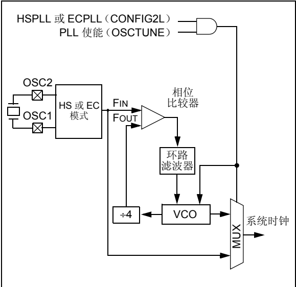
图 2-5: PLL 框图
