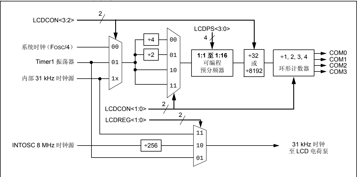
图 15-2: LCD 时钟的产生
