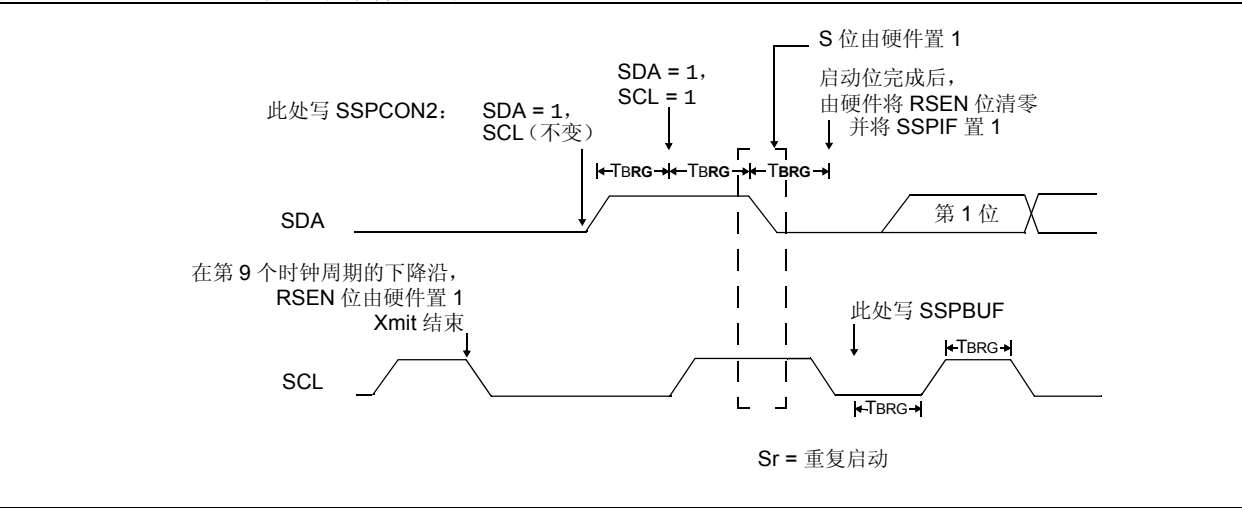
图 16-22: 重复启动条件波形图
