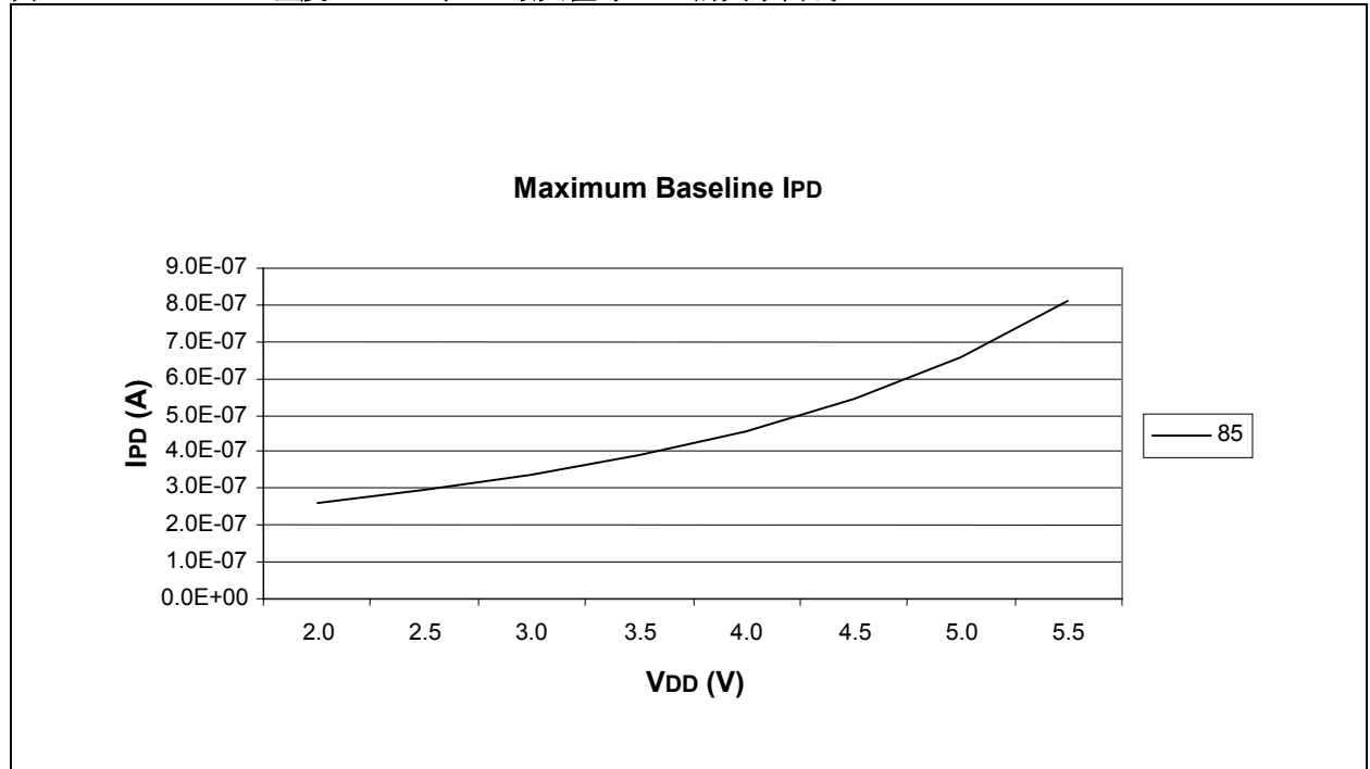
图 13-5: 温度 +85°C 时 IPD 最大值与 VDD 的关系曲线
