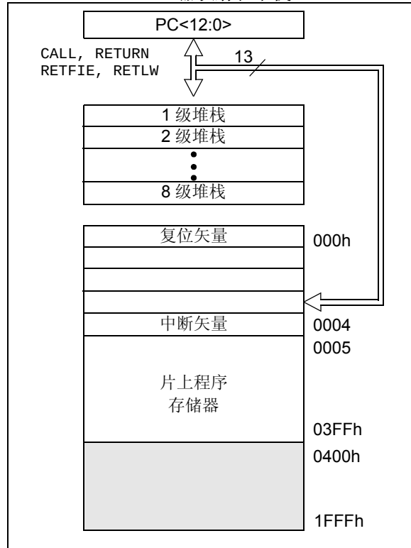
图 2-1: PIC12F629/675 的程序存储器映射和堆栈
