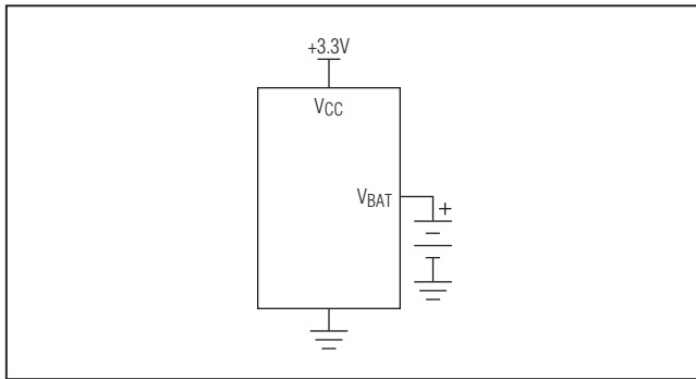
图6. 双电源
