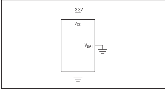
图4. 单电源(V CC )
