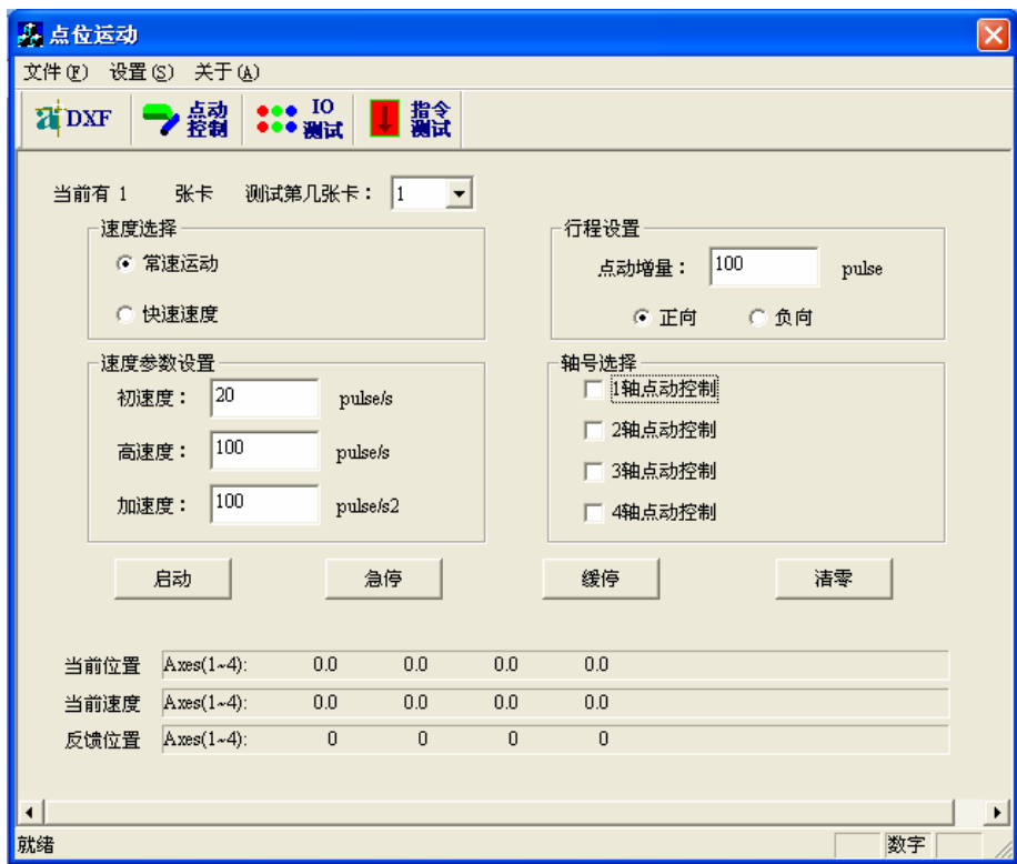
图 4-4 点动控制模块
