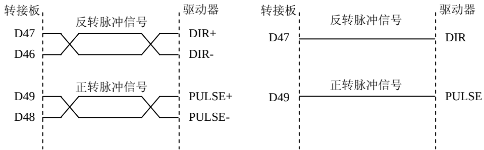
(a) 双脉冲双端方式
