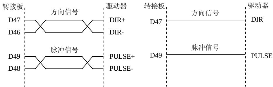
(a) 脉冲/方向双端方式
