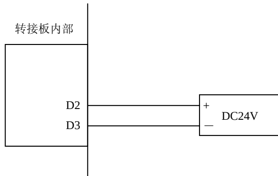
图 3-5 转接板与外部电源连接示意图
