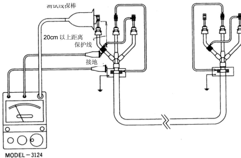
图 2 使用保护线
