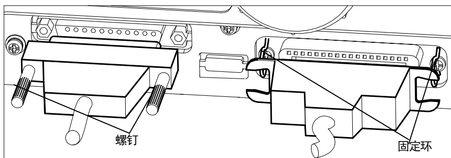
串口(选件)
