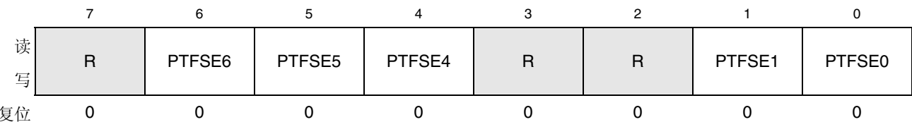
图 6-36. F 口输出斜率控制使能寄存器（PTFSE）
