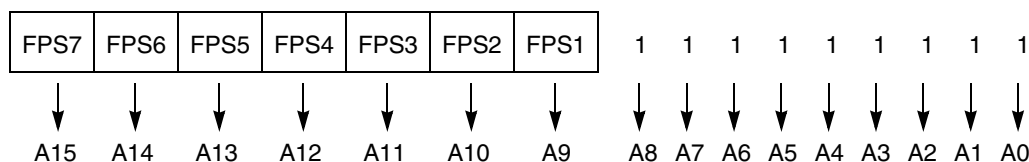
图 4-4. 块保护机制
