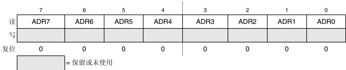
图 14-6. 数据低结果寄存器 (ADCRL)
