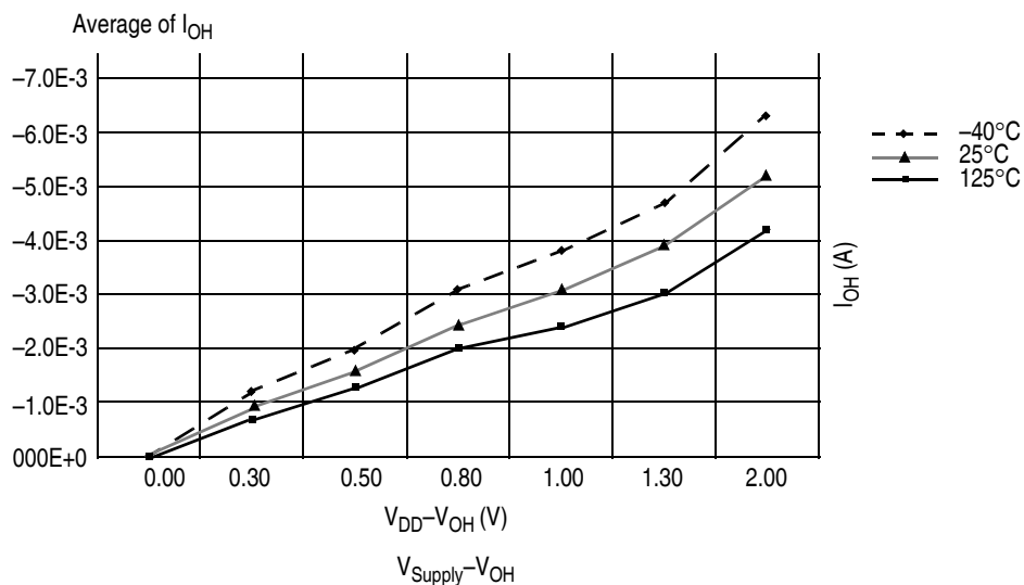
图 A-3. V_{DD} = 5\text{ V} 时, I_{OH} (低驱动) 和 V_{DD}-V_{OH} 的典型值
