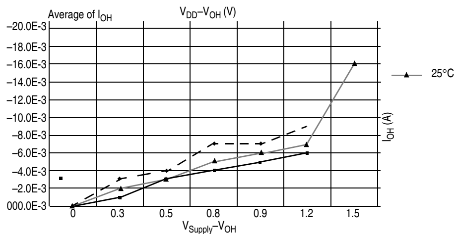
图 A-2. V_{DD} = 3\text{ V} 时, I_{OH} (低驱动) 和 V_{DD}-V_{OH} 的典型值
