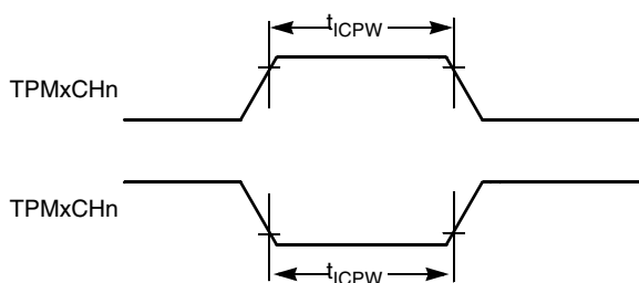
图 A-15. 定时器输入捕获脉冲
