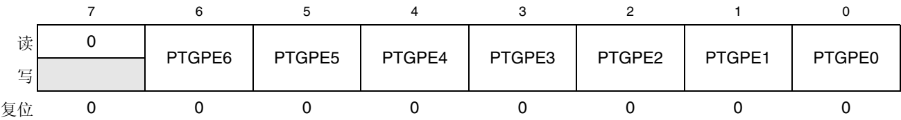
图 6-40. G 口内部上拉电阻使能（PTGPE）
