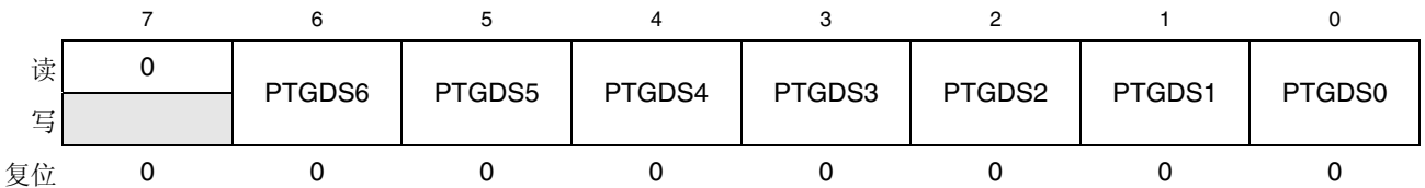
图 6-42. G 口输出驱动强度寄存器（PTGDS）
