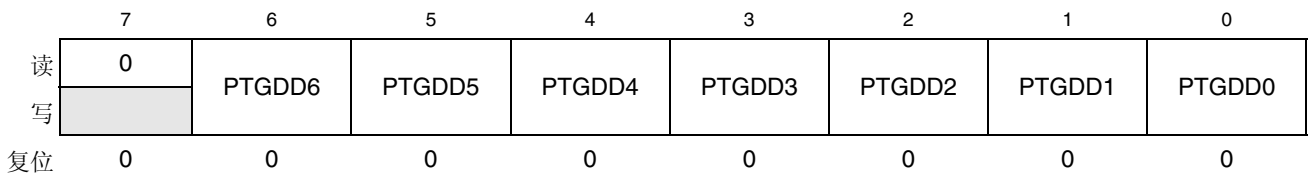
图 6-39. G 口数据方向寄存器（PTGDD）
