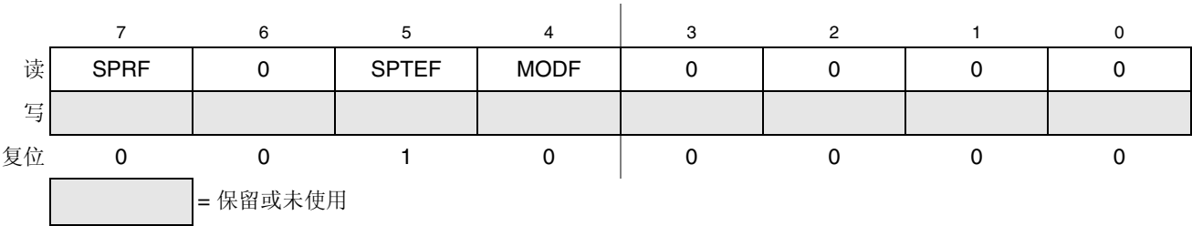
图 12-8. SPI 状态寄存器 (SPIS)
