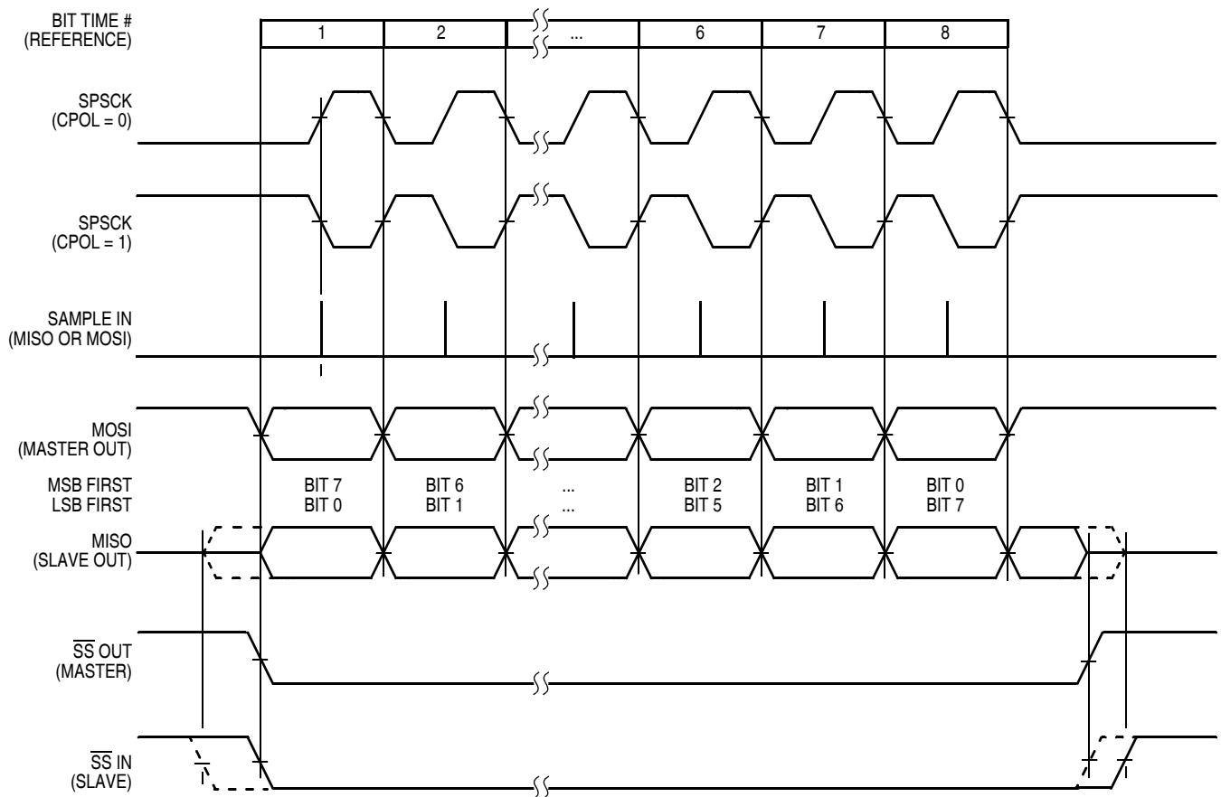
图 12-11. SPI 时钟格式 (CPHA=0)
