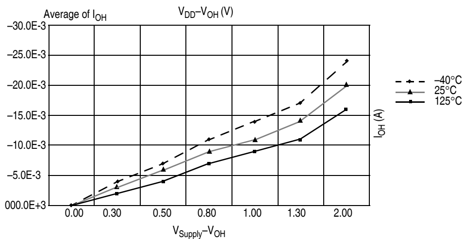
图 A-4. V_{DD} = 3\text{ V} 时, I_{OH} (低驱动) 和 V_{DD}-V_{OH} 的典型值
