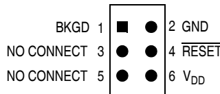
图 15-1. 工具接口
