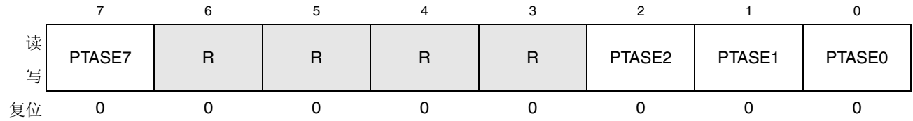
图 6-12. A 口输出斜率控制使能寄存器（PTASE）
