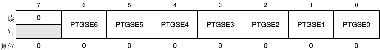
图 6-41. G 口输出斜率控制使能寄存器（PTGSE）
