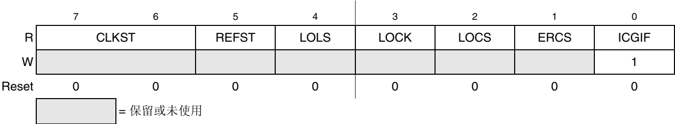
图 9-8. ICG 状态寄存器 1（ICGS1）
