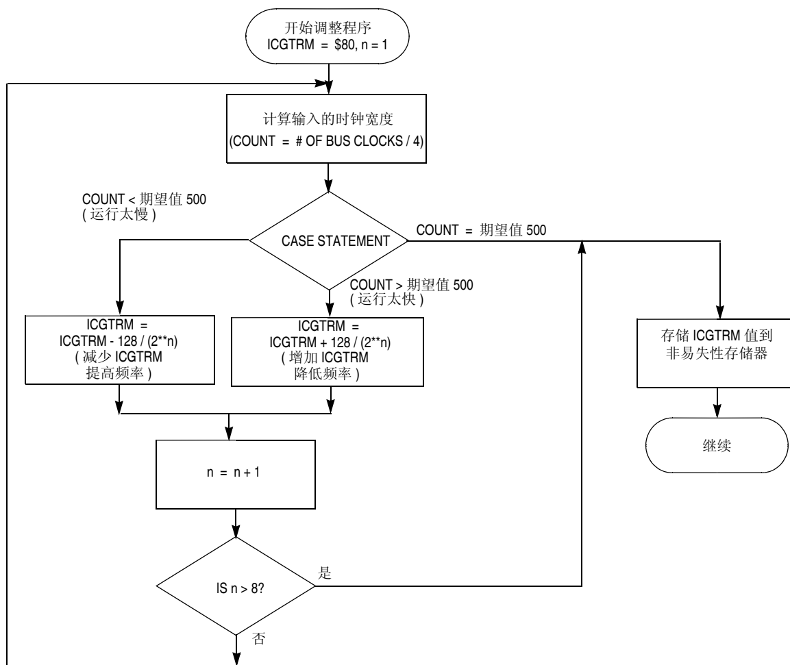
图 9-17. 调整程序
