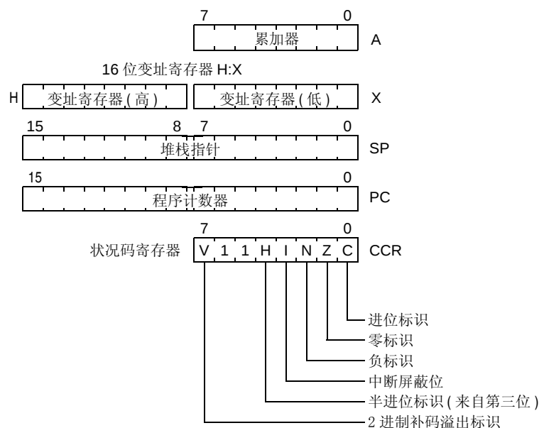
图 7-1. CPU 寄存器
