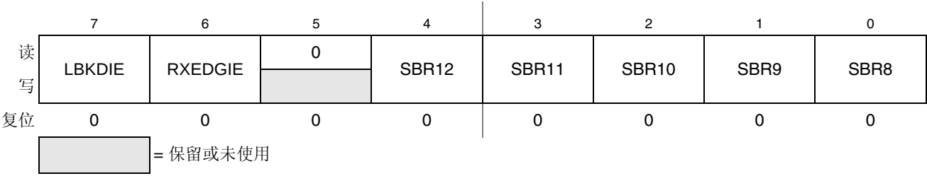
图 11-4. SCI 波特率寄存器（SCIxBDH）
