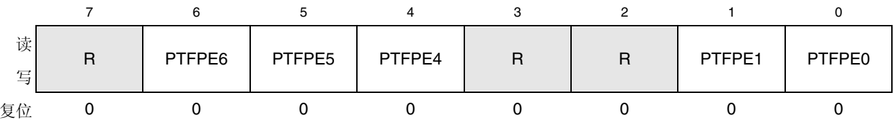
图 6-35. F 口内部上拉电阻使能（PTFPE）
