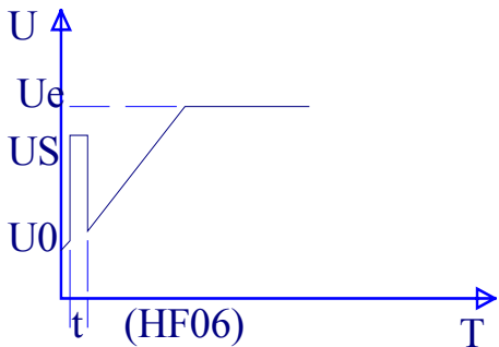
突跳起动特性曲线 图（3）
