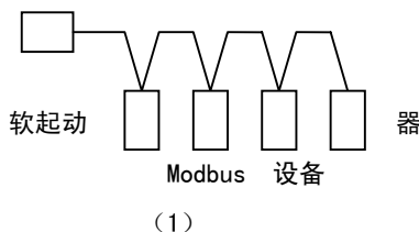
正确接法
