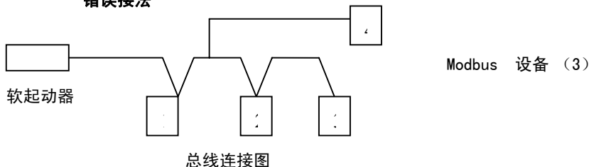
错误接法
