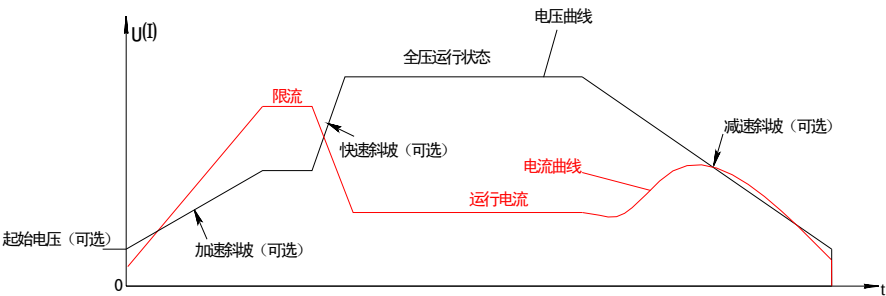
软起/软停电压（电流）特性曲线
