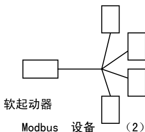
错误接法
