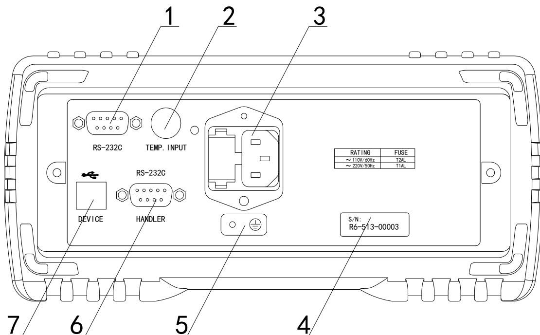
图 2-2 后面板说明
