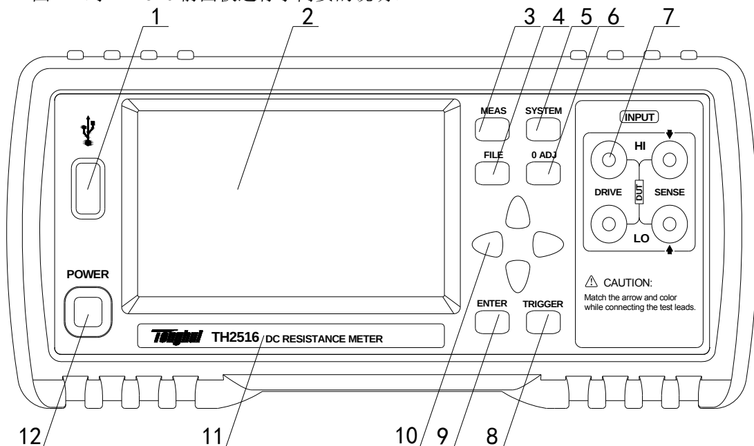
图 2-1 前面板说明
