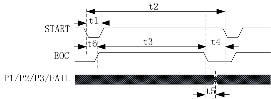
时序图
