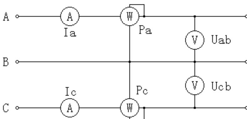
图十九 三相三线制测量原理图
