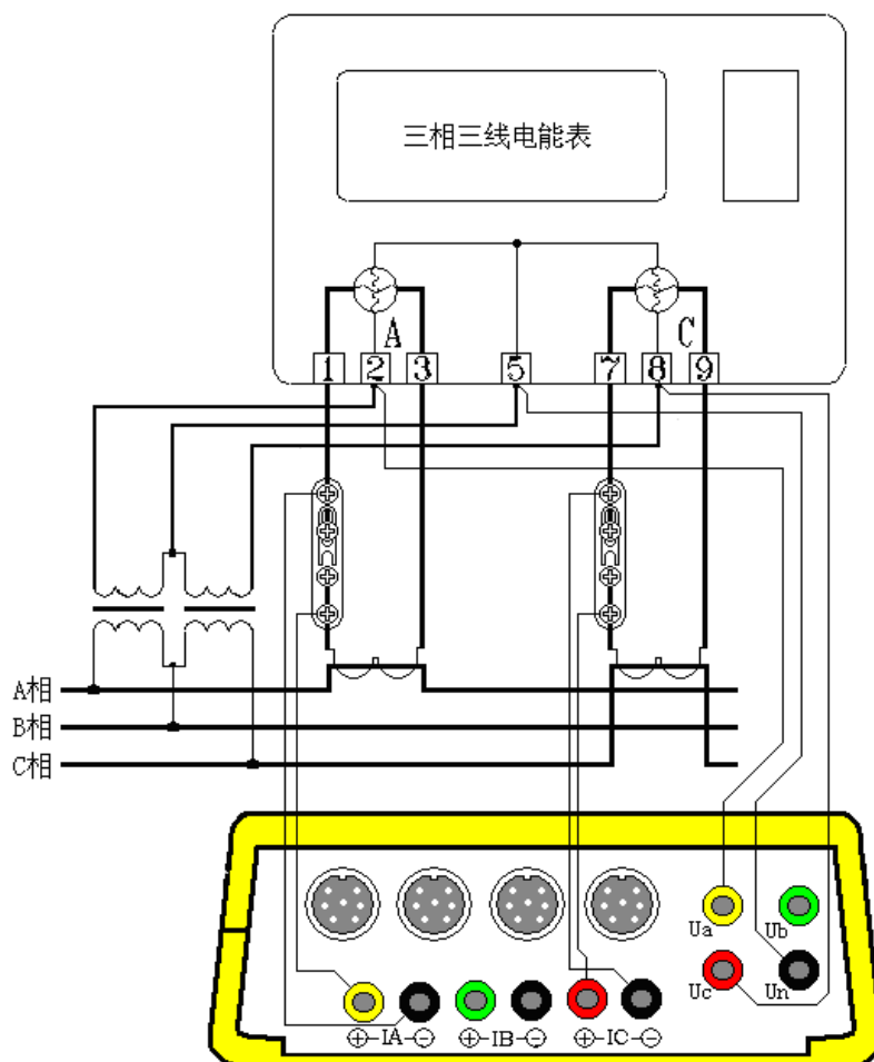
三相三线高压表计经内部CT接入接线
