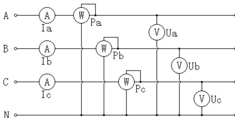
图二十 三相四线制测量原理图
