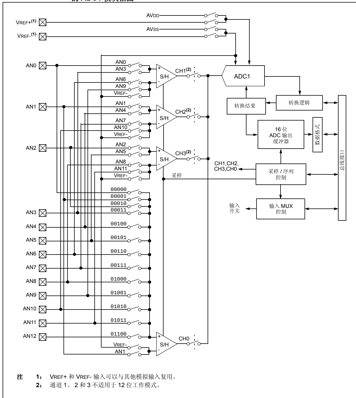
图 20-1: dsPIC33FJ32GP304、dsPIC33FJ64GP204/804 和 dsPIC33FJ128GP204/804 器件的 ADC1 模块框图
