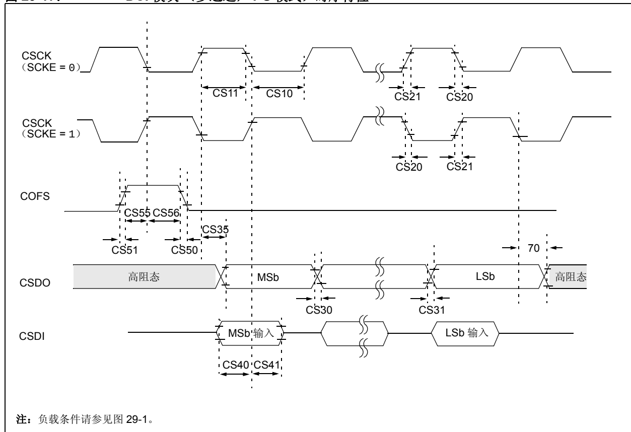
图 29-17: DCI 模块 (多通道, I 2 S 模式) 时序特性
