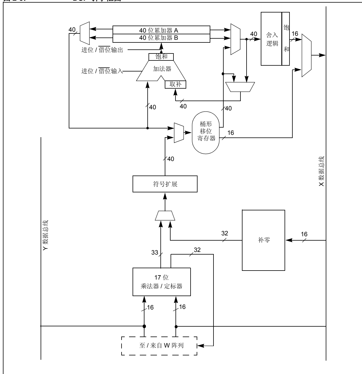
图 2-3: DSP 引擎框图
