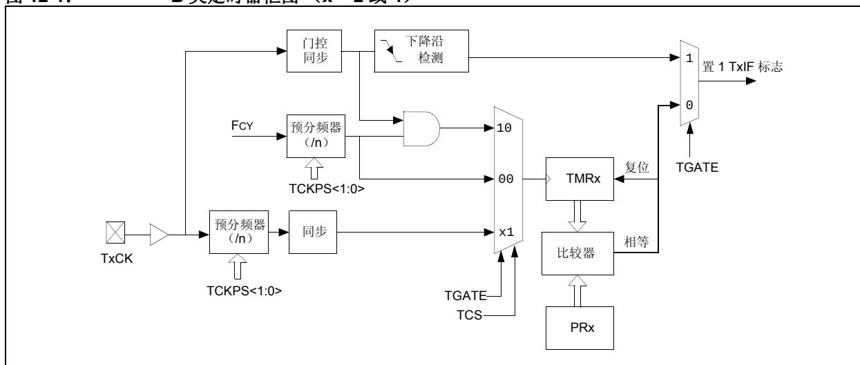
图 12-1: B 类定时器框图 (x = 2 或 4)
