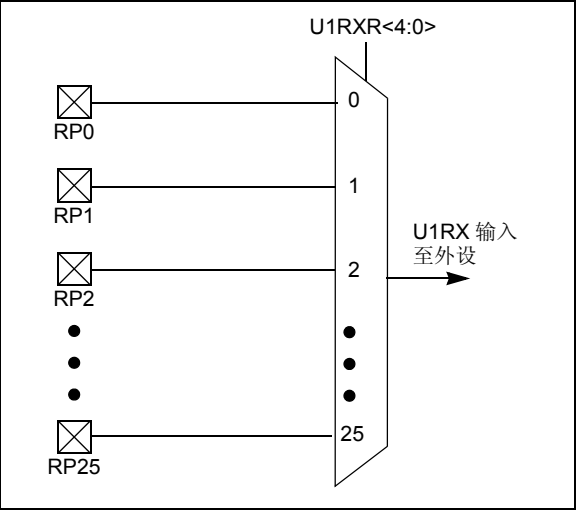
图 10-2: U1RX 的可重映射多路开关 (MUX) 输入
