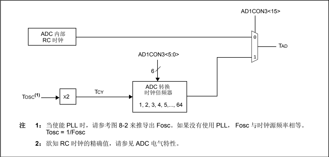
图 20-3: ADC 转换时钟周期框图
