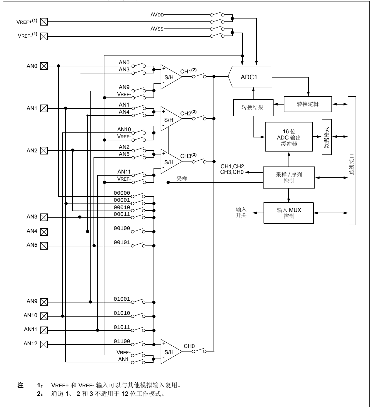
图 20-2: dsPIC33FJ32GP302、dsPIC33FJ64GP202/802 和 dsPIC33FJ128GP202/802 器件的 ADC1 模块框图
