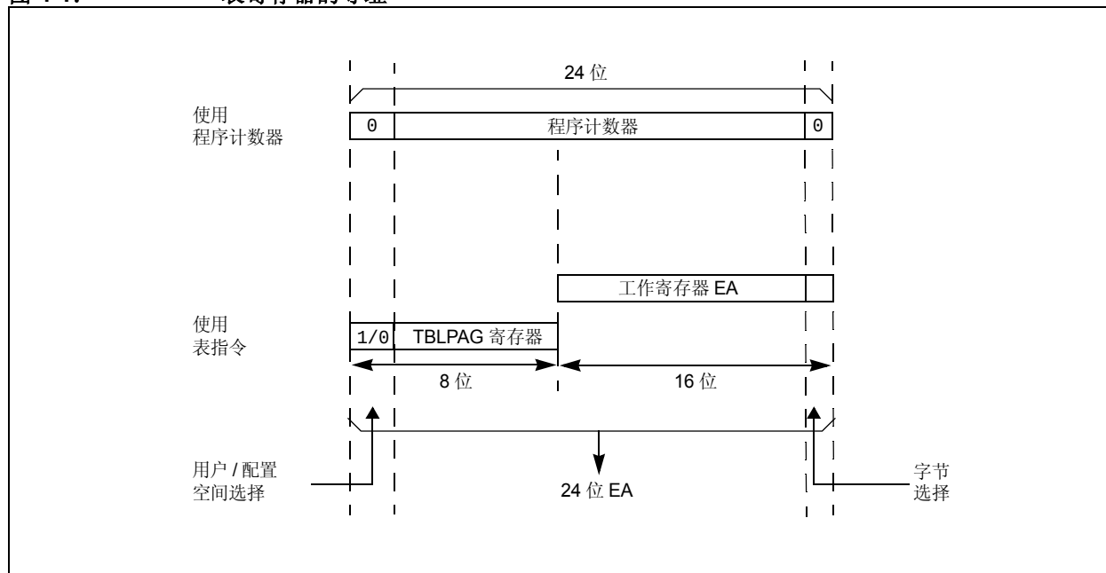
图 4-1： 表寄存器的寻址
