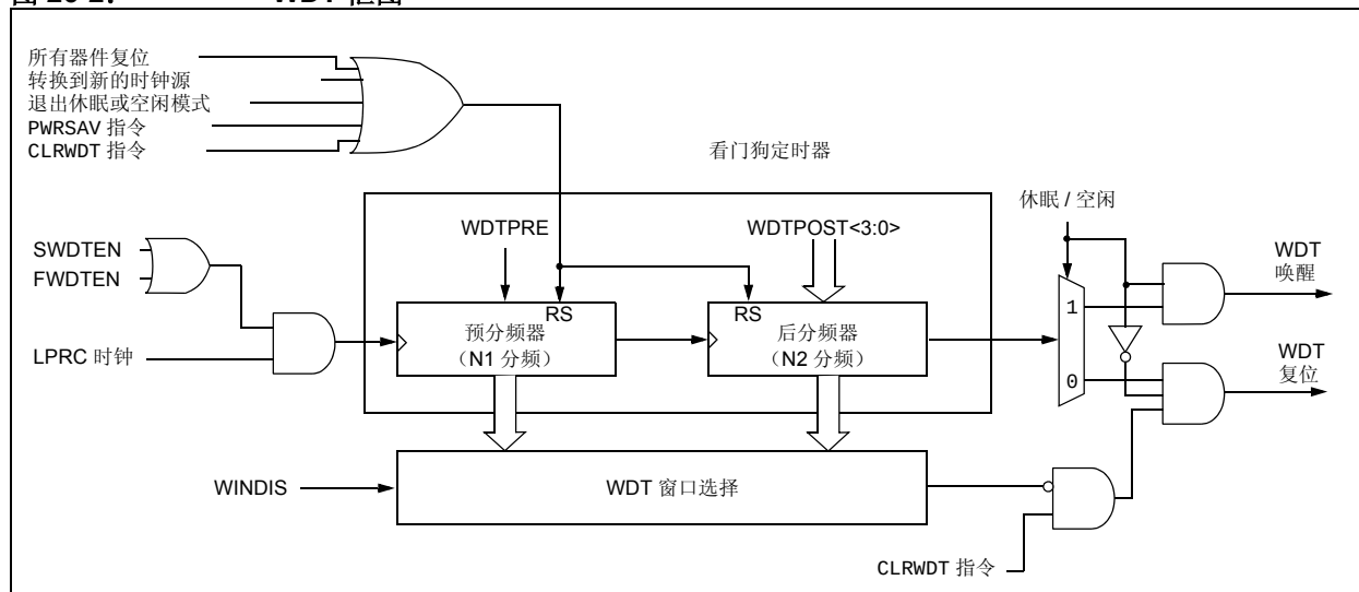
图 26-2: WDT 框图
