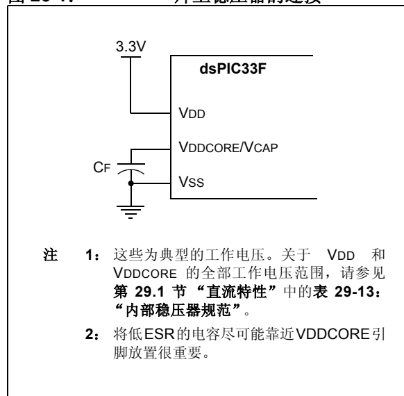
图 26-1: 片上稳压器的连接 (1)
