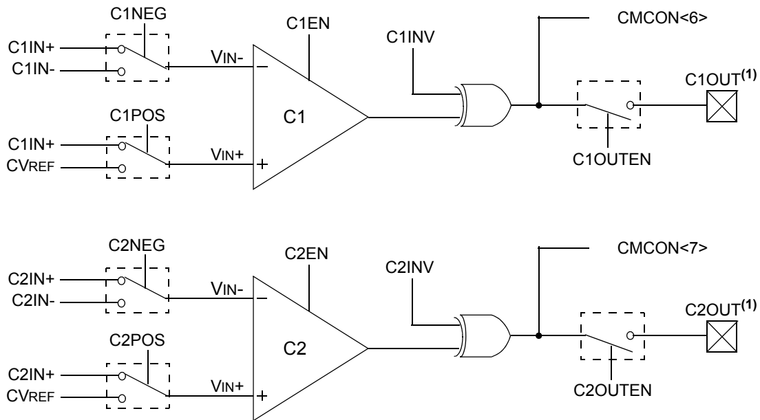
图 22-1: 比较器 I/O 工作模式
