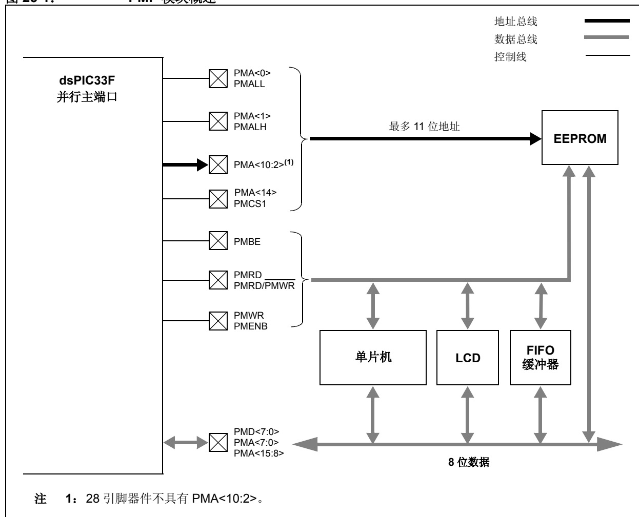
图 25-1: PMP 模块概述
