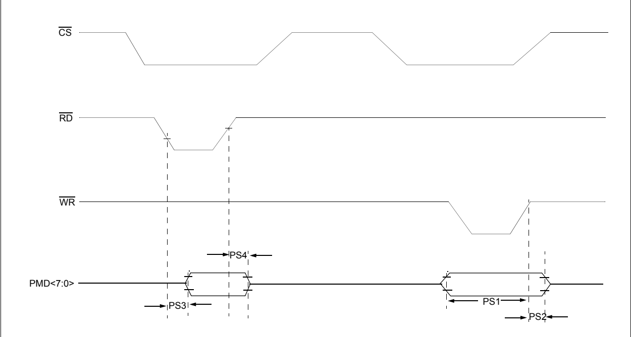
图 29-23: 并行从端口时序图
