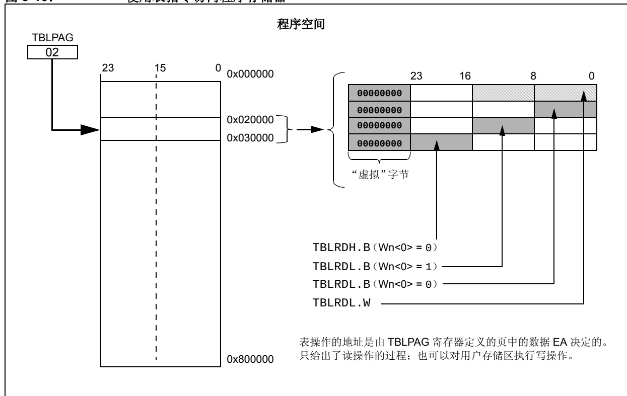
图 3-10： 使用表指令访问程序存储器
