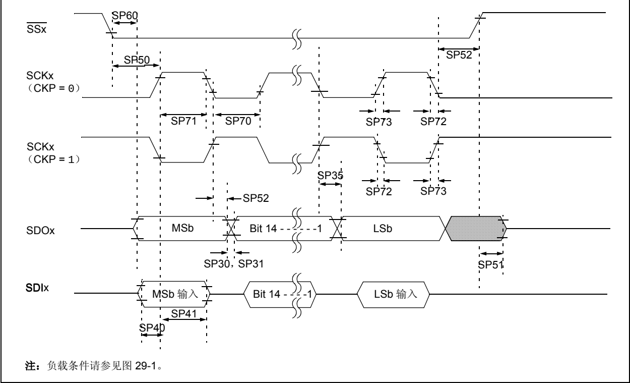
图 29-12: SPIx 模块从模式 (CKE = 1) 时序特性
