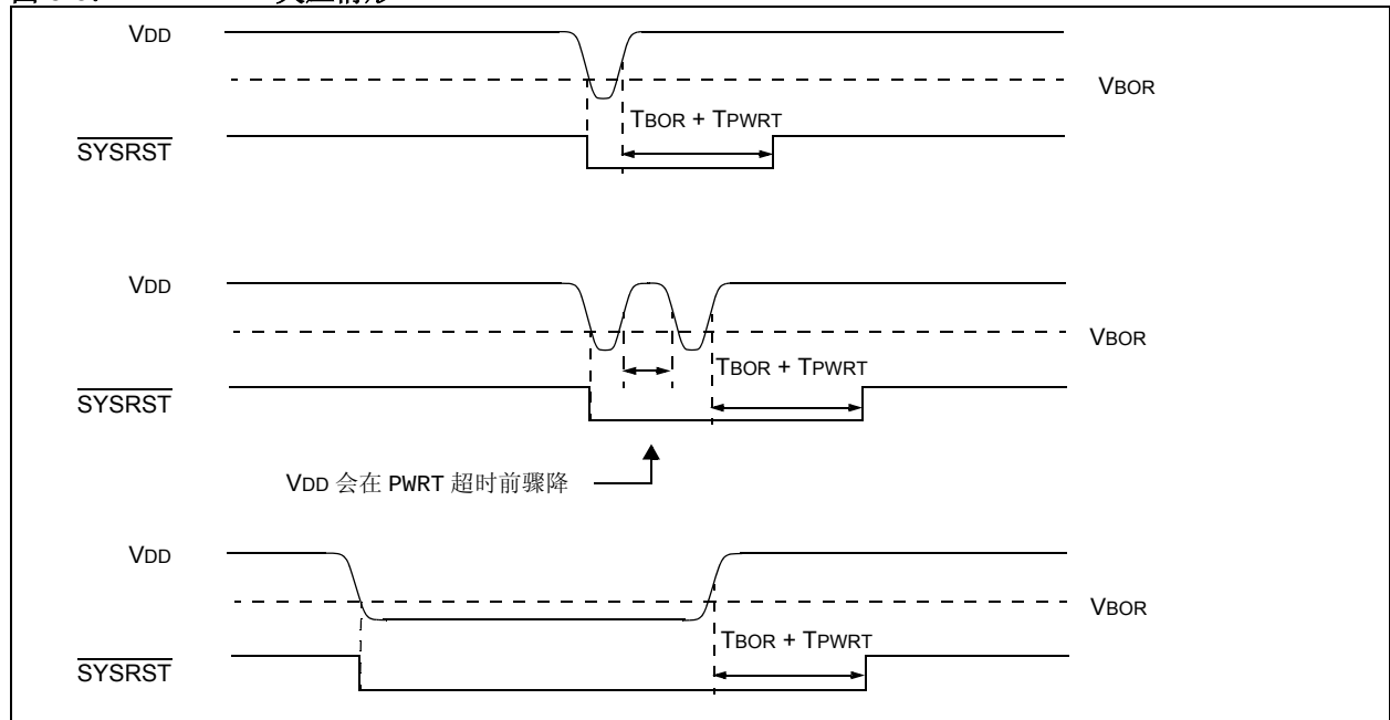
图 5-3: 欠压情形
