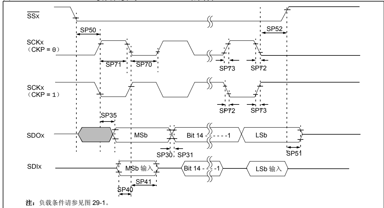
图 29-11: SPIx 模块从模式 (CKE = 0) 时序特性
