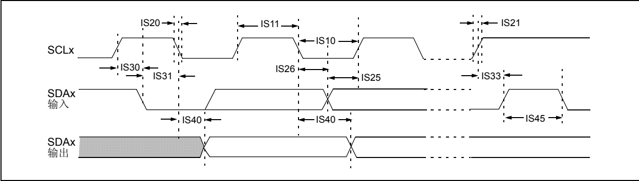
图 29-16: I2Cx 总线数据时序特性 (从模式)
