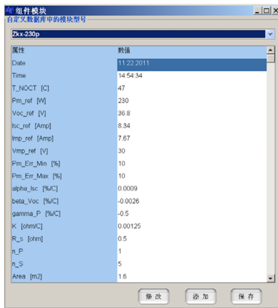
图 B-6 组件模块型号及其参数列表
