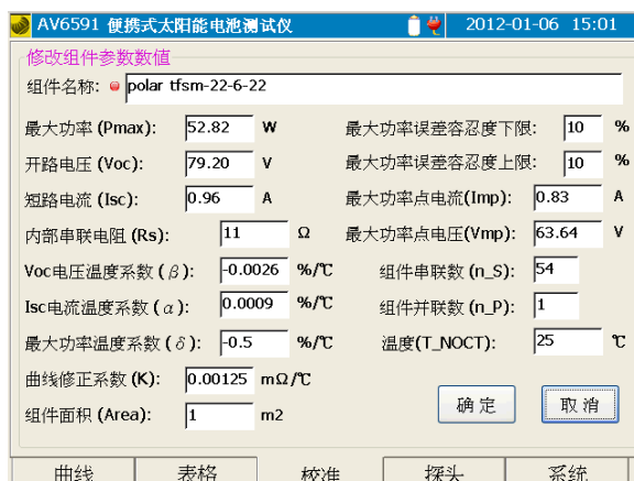
图 5-17 组件参数修改窗口
