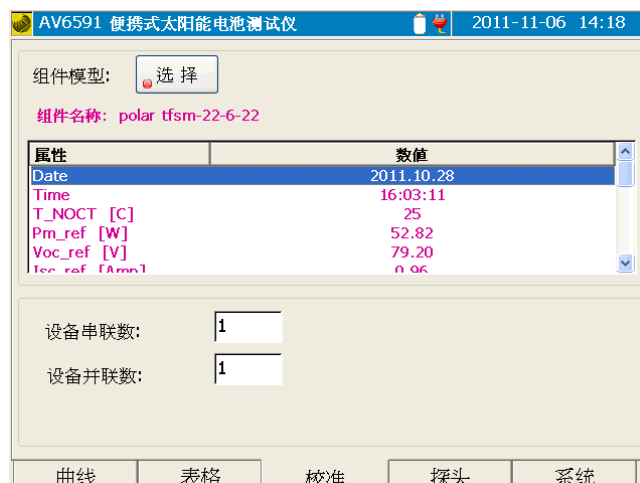
图 4-8 校准界面示意图
