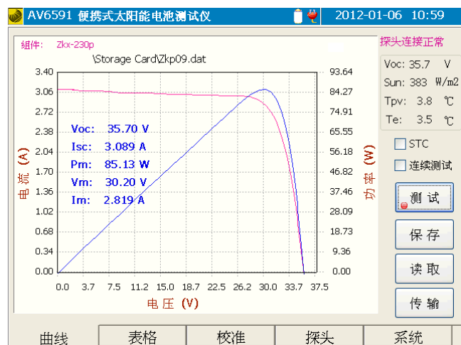
图 4-10 曲线窗口示意图
