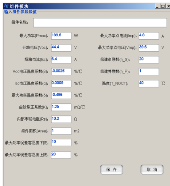
图 B-7 组件名称和参数添加窗口
