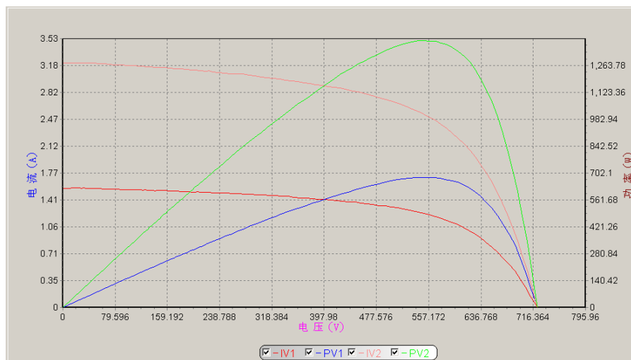
图 B-2 曲线显示窗口示意图
