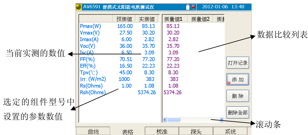
图 5-9 表格窗口示意图
