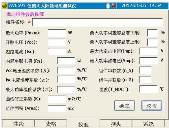
图 5-15 添加组件参数示意图
