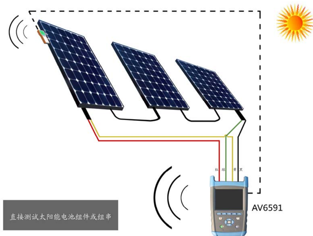
图 4-7 直接测试太阳能电池组串示意图
