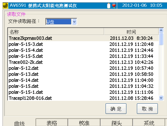
图 5-6 读取文件界面示意图
