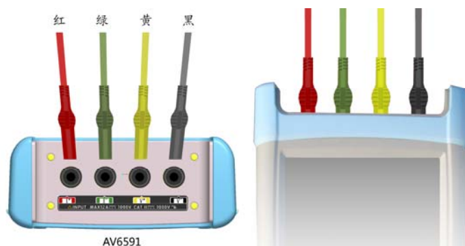
图 4-2 主机与测试线连接示意图
