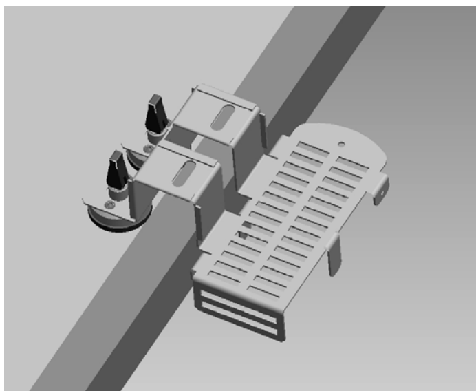
图 4-1 探头盒安装示意图
