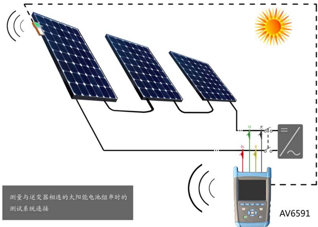
图 4-6 光伏电站中电池组串测试示意图
