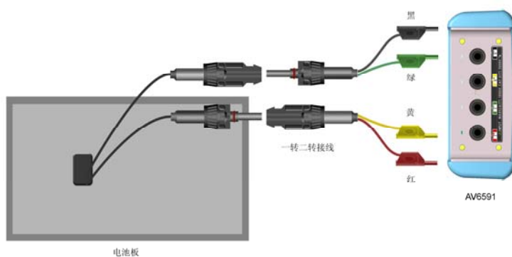
图 4-4 通过转接线缆与电池板直接连接示意图
