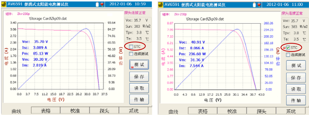
当前测试条件下的原始测试曲线 转换为 STC 下的测试曲线
