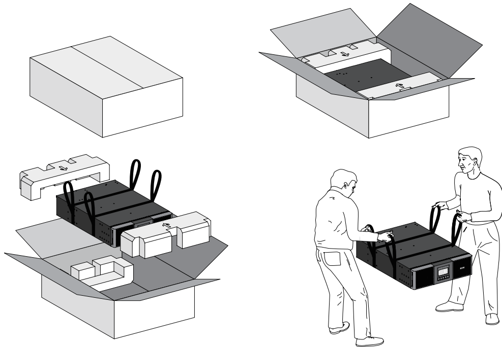
拆箱 UPS 和延长电池模块。
