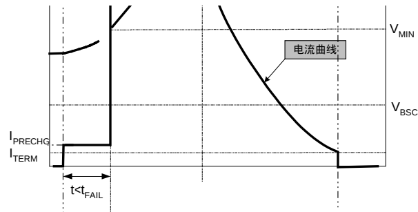
图 4 充电过程中的电流、电压曲线
