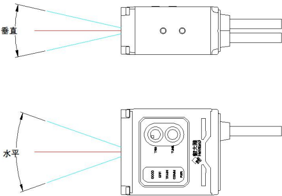
图 3. Soldier100 系列识读角度示意图
