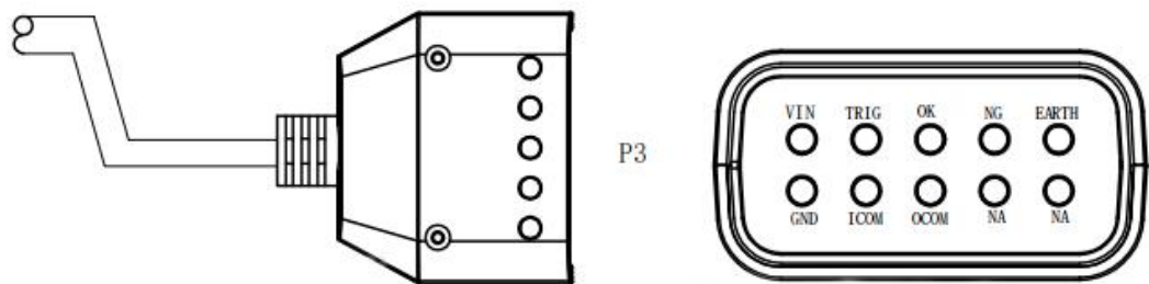
图 5. Soldier100 系列 I/O 接线盒子示意图
