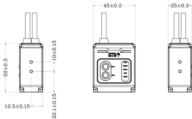
图 2. Soldier100/160 外观尺寸图
