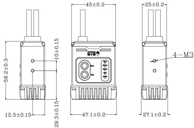
Soldier180 外观尺寸图
