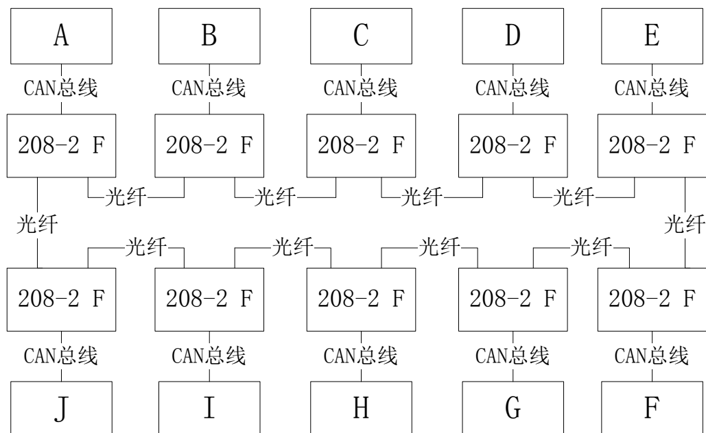
GCAN-208-2 F 典型应用——环网
