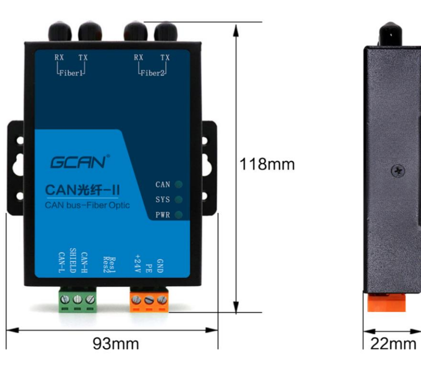
图 2.1 GCAN-208 外形尺寸
