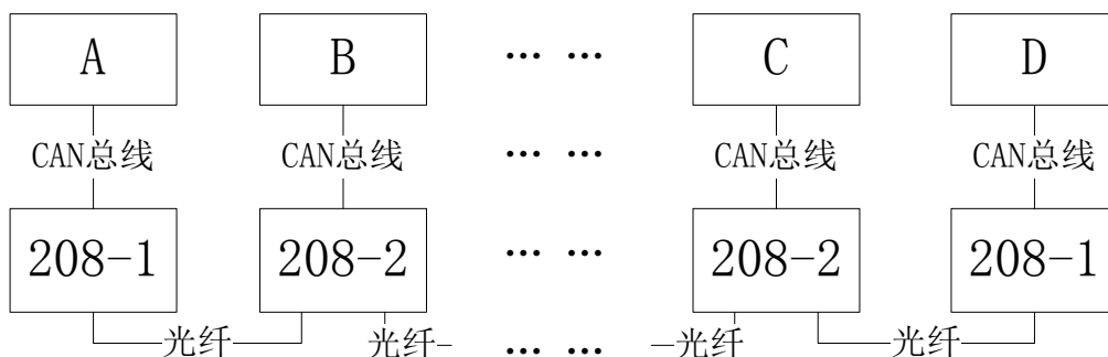
GCAN-208-2 典型应用——手拉手级联
