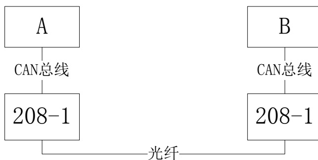
GCAN-208-1 典型应用——成对使用
