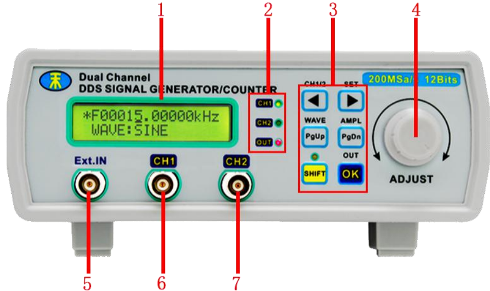
图 2-1-1 MHS5200A 前面板图
