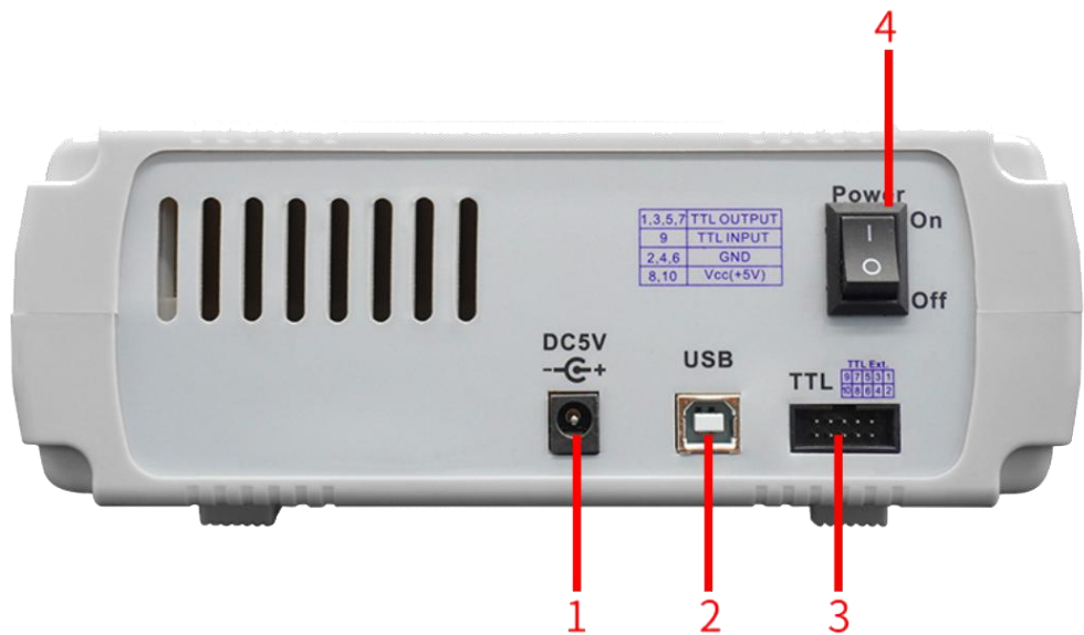
图 2-1-2 MHS5200A 后面板图
