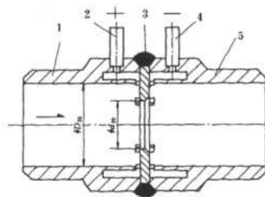
图(5) 环室取压标准孔板结构与安装示意图
