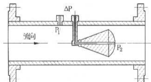
图(40) V型锥流量计结构简图
