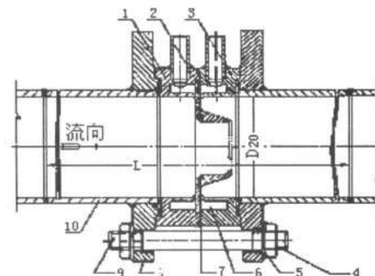
1. 前环室 2. 标准喷嘴 3. 垫片 4. 紧固螺母 5. 垫圈 6. 后环室 7. 垫片 8. 法兰 9. 双头螺栓 10. 管道
