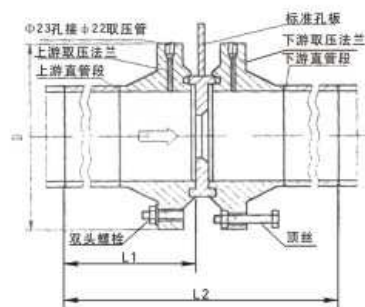
图(11) 法兰取压标准孔板结构与安装示意图 (DN≤400, PN≤10MPa)
