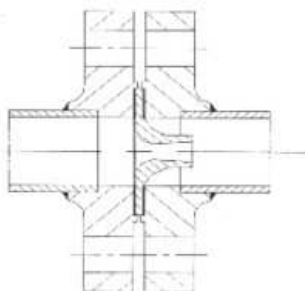
图(47) 音速喷嘴安装示意图
