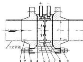
图(3) 环室取压标准孔板结构与安装示意图
