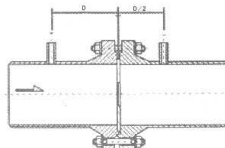
图(14) 径距取压标准孔板结构与安装示意图 (DN≤500, PN≤4MPa)
