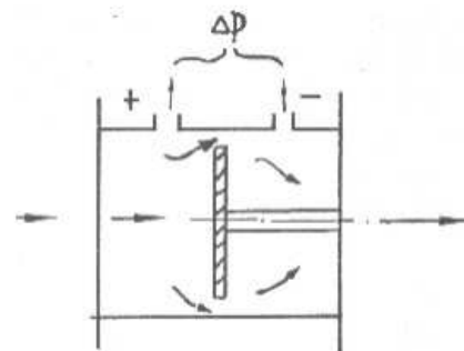
图(15) 环形孔板工作原理图
