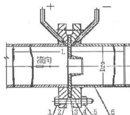
1.螺栓 2.垫片 3.标准喷嘴 4.法兰 5.螺母 6.管道
