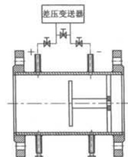
图(21)一体型
