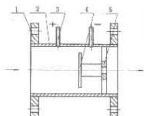
1. 本体法兰 2. 测量管 3. 取压管 4. 测流板 5. 支撑件
