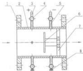
1. 本体法兰 2. 测量管 3. 取压管 4. 均压环 5. 引压管 6. 测流板 7. 支撑件 8. 排污堵头
