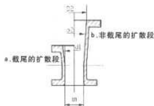
图(30) 文丘里喷嘴外形图
