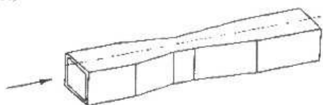
图(41)矩形文丘里管结构简图
