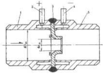
1.前取压环室 2.取压管 3.喷嘴 4.取压管 5.后取压环室 图(27)角接(环室)取压焊接结构标准喷嘴结构与安装示意图 (DN≤250, PN≤32MPa)
