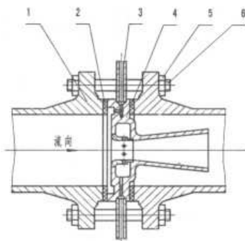
图(31) 文丘里喷嘴结构和安装示意图
