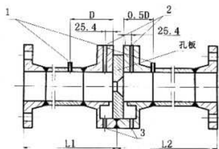
图(1)取压方式和取压位置示意图
