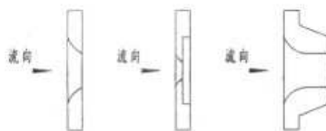
图(32) 四分之一圆孔板
