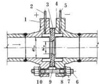
图(4) 环室取压标准孔板结构与安装示意图
