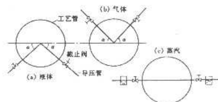
图(48) 取压口位置安装示意图
