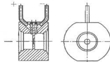
图(43) 内藏孔板
