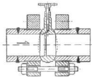
图(8)单独钻孔取压标准孔板结构与安装示意图 (高压透镜孔板)( DN \leq 200 , PN \leq 32MPa )
