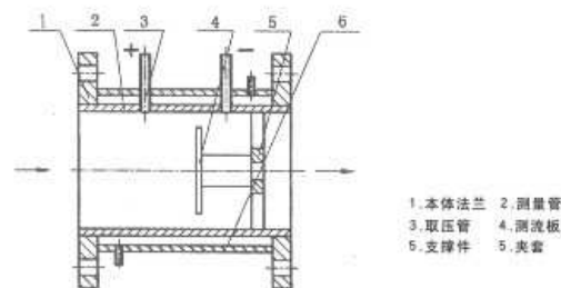
图(18)夹套保温型
