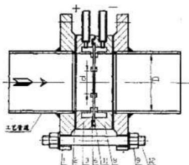
图(2) 环室取压标准孔板结构与安装示意图
