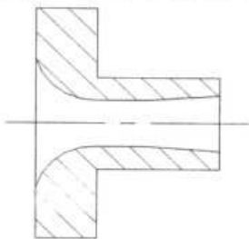
图(44) 圆环形喉部文丘里喷嘴
