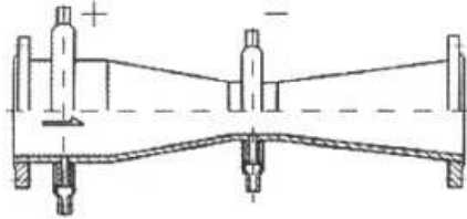
图(29)经典文丘里管结构示意图
