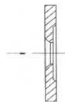
图(34) 锥形入口孔板
