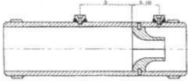
图(28)长径喷嘴结构示意图 Dn50~600, PN≤42MPa
