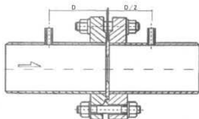
图(13) 径距取压标准孔板结构与安装示意图 (DN≤1600, PN≤2.5Mpa)
