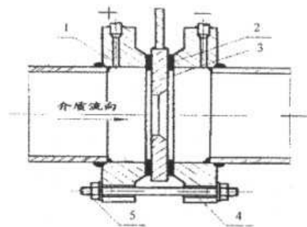
1.平焊法兰 2.垫片 3.标准孔板 4.双头螺柱 5.螺母
