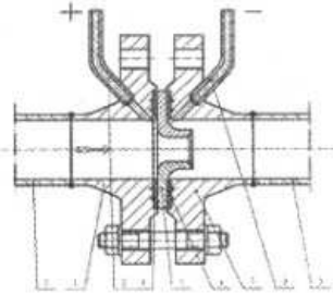
图(25)角接(环室)取压标准喷嘴结构与安装示意图 (DN≤400, PN≤10MPa)
