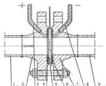
1.前直管段 2.正取压法兰 3.正取压管 4.垫片 5.标准孔板 6.垫片 7.负取压法兰 8.负取压管 9.后直管段
