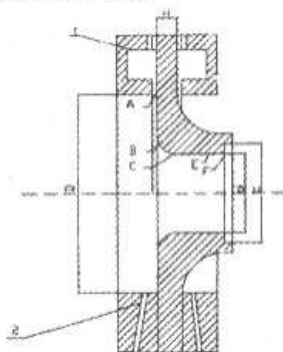
1.环室角接取压 2.单独钻孔角接取压
