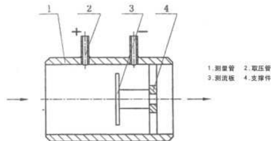
图(19)高压型
