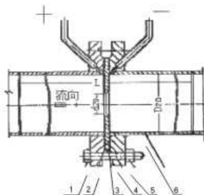
1.螺栓或螺柱 2.垫片 3.标准孔板 4.法兰 5.螺母、垫圈 6.管道
