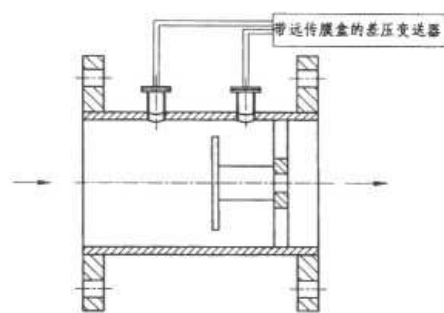
图(20)脏污流体型
