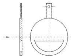
图(35) 圆缺孔板
