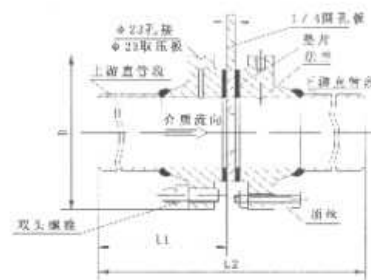
图(33) 四分之一圆孔板结构安装示意图
