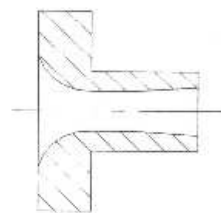
图(45) 圆筒形喉部文丘里喷嘴
