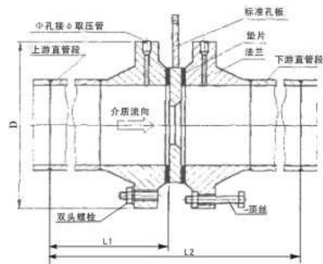
图(10)法兰取压标准孔板结构与安装示意图 ( DN \leq 500 , PN \leq 4MPa )
