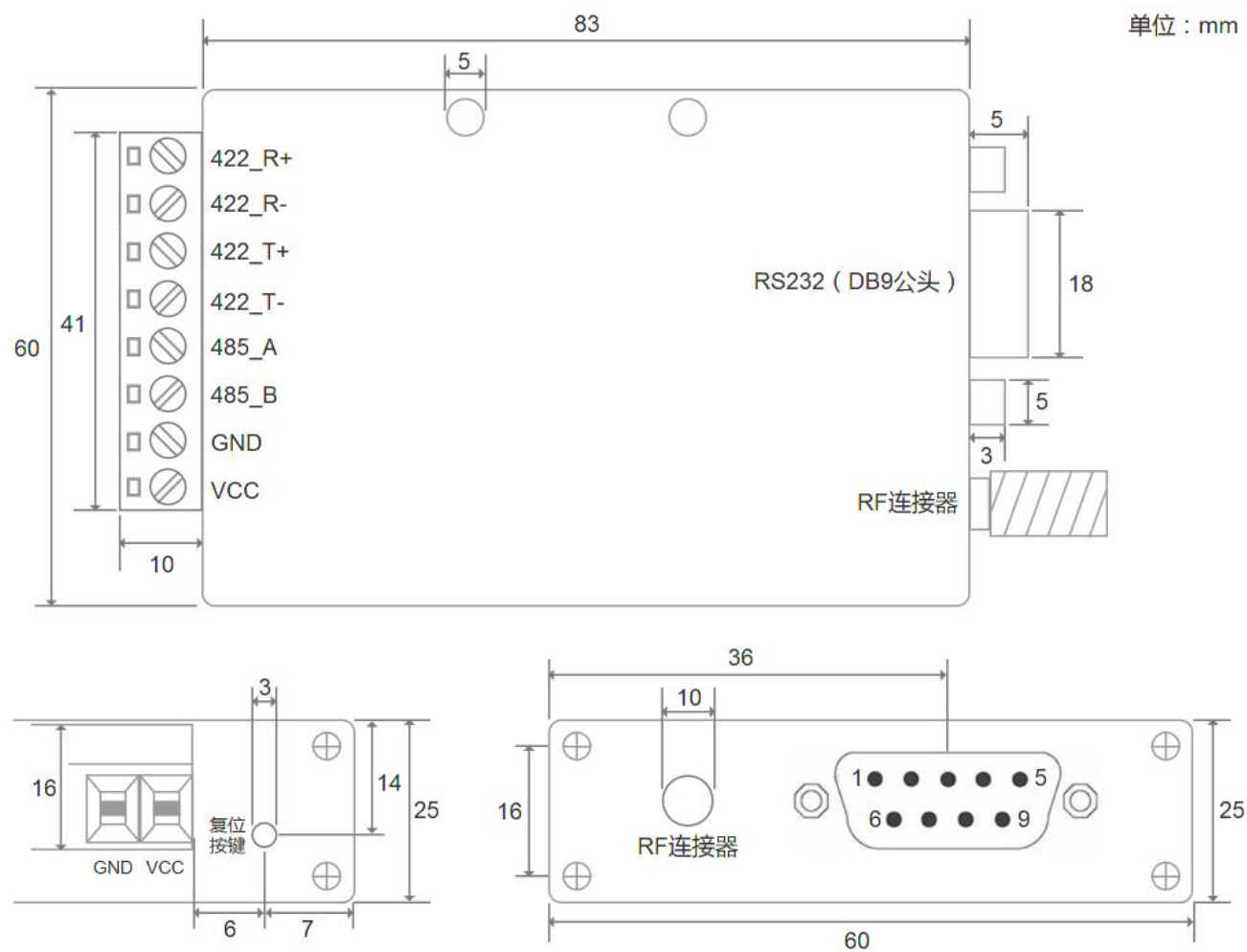
图 3.1 LR100 尺寸图
