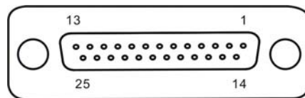
图 B-3 串行接口插座引脚序号
