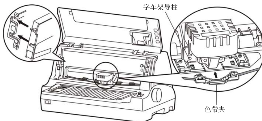
图 2-10 安装色带盒
