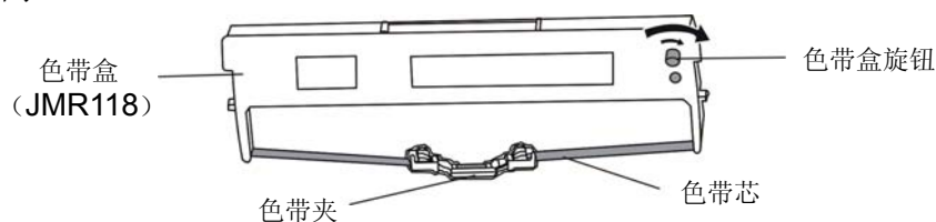
图 2-9 色带盒
