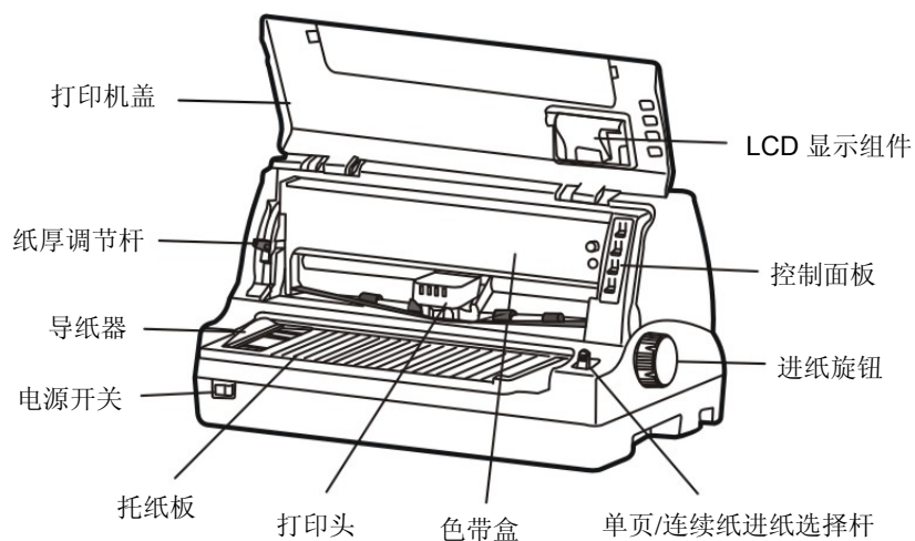
图 2-3 打印机主要部件（前视图）
