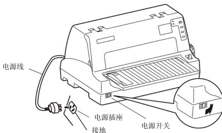
图 2-15 连接电源线
