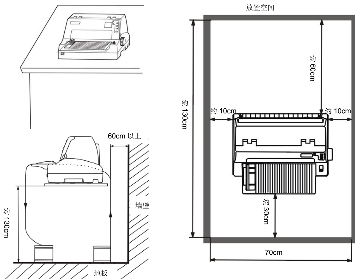
图 2-5 打印机放置
