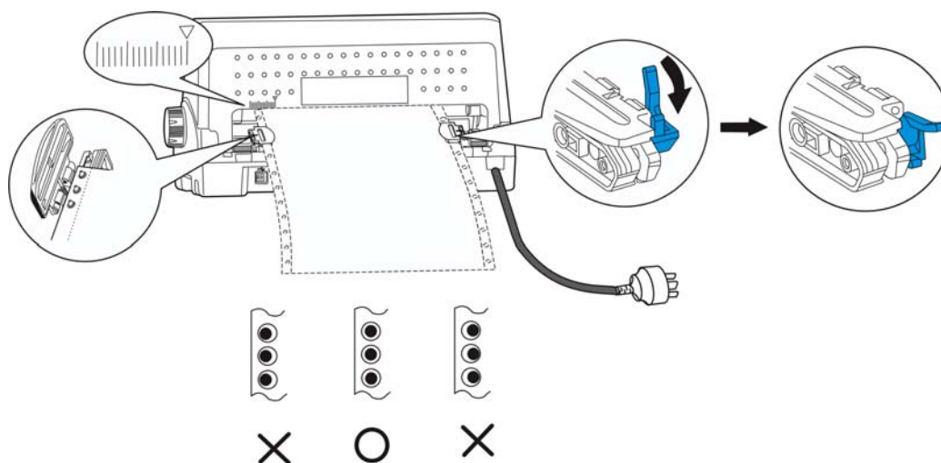
图 3-10 调整连续纸位置
