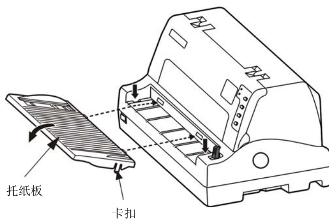
图 2-6 安装托纸板
