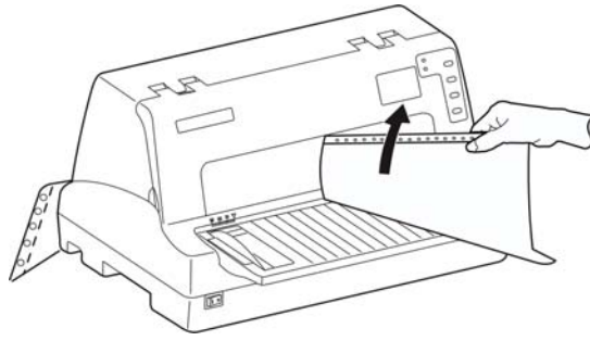
图 3-11 撕连续纸
