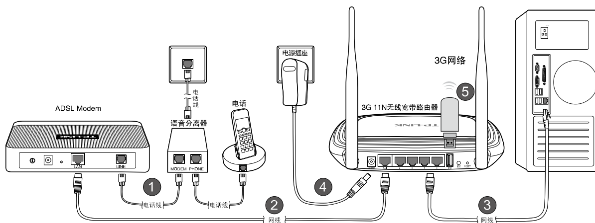
图 4-1 TL-MR3420 硬件安装示意图
