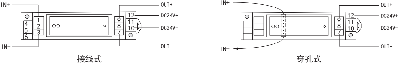
四线制输出接线图（输入/输出/电源三隔离）
