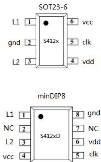
图2 脚位图
