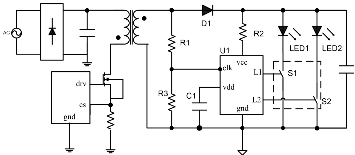
图1 S4120/D的典型应用图
