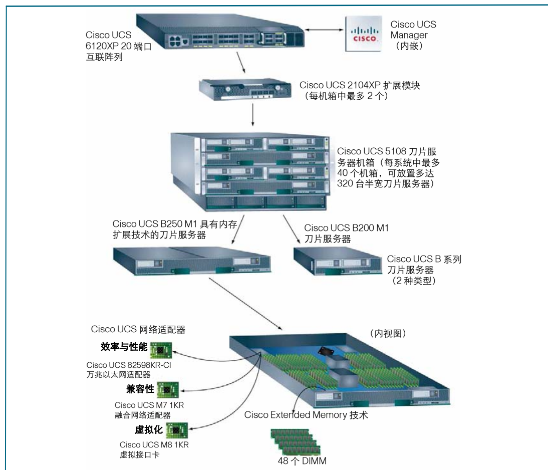
图 1. 思科统一计算系统是一个紧密结合的高可用性架构
