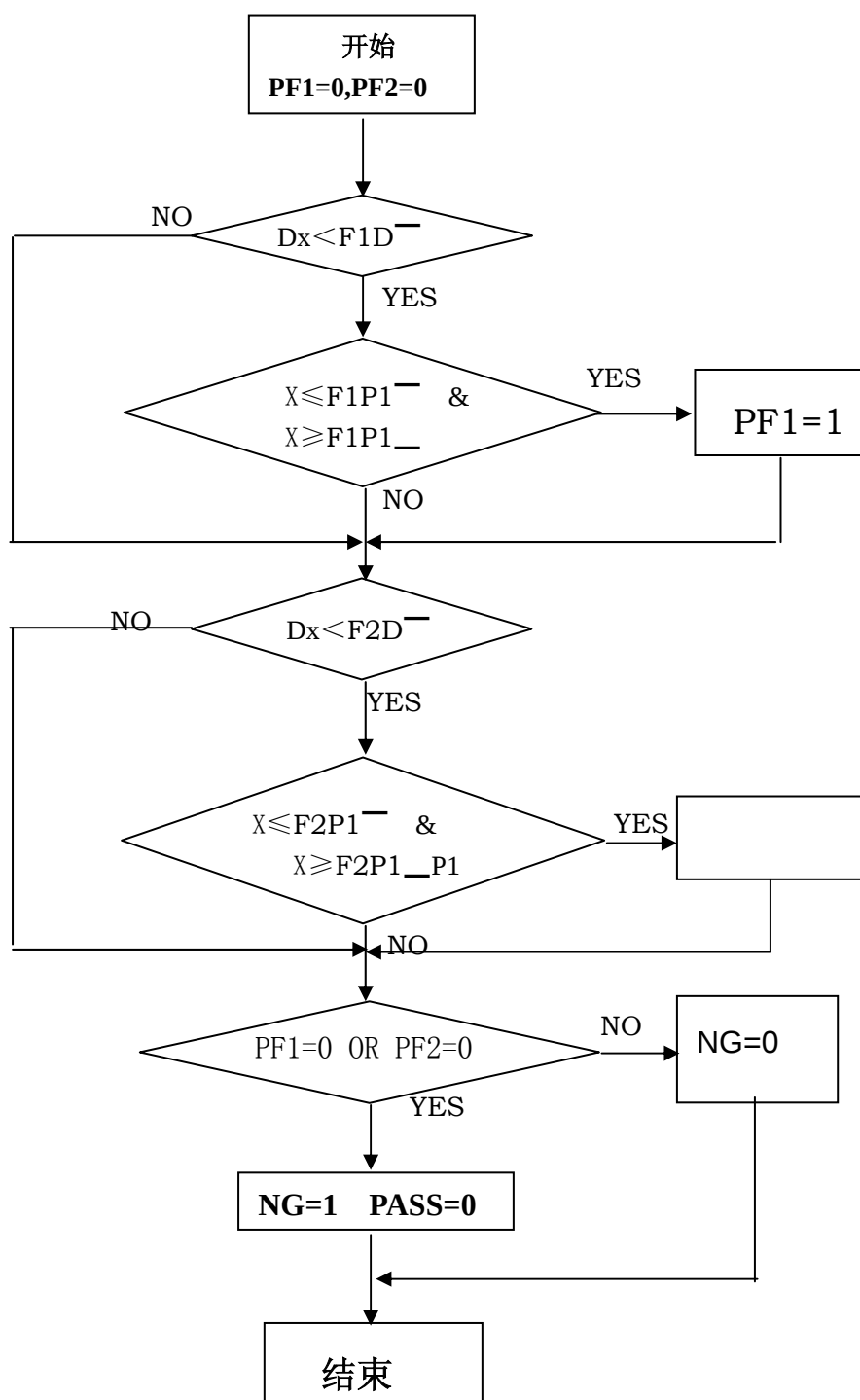
图 2-6A 为 TH2617、TH2617A 单频时的分选判别流程，
