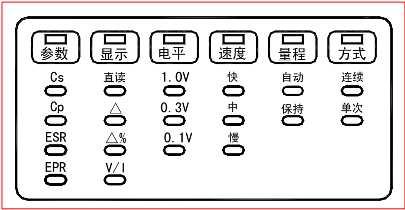
图 2-2A TH2617 状态指示示意图
