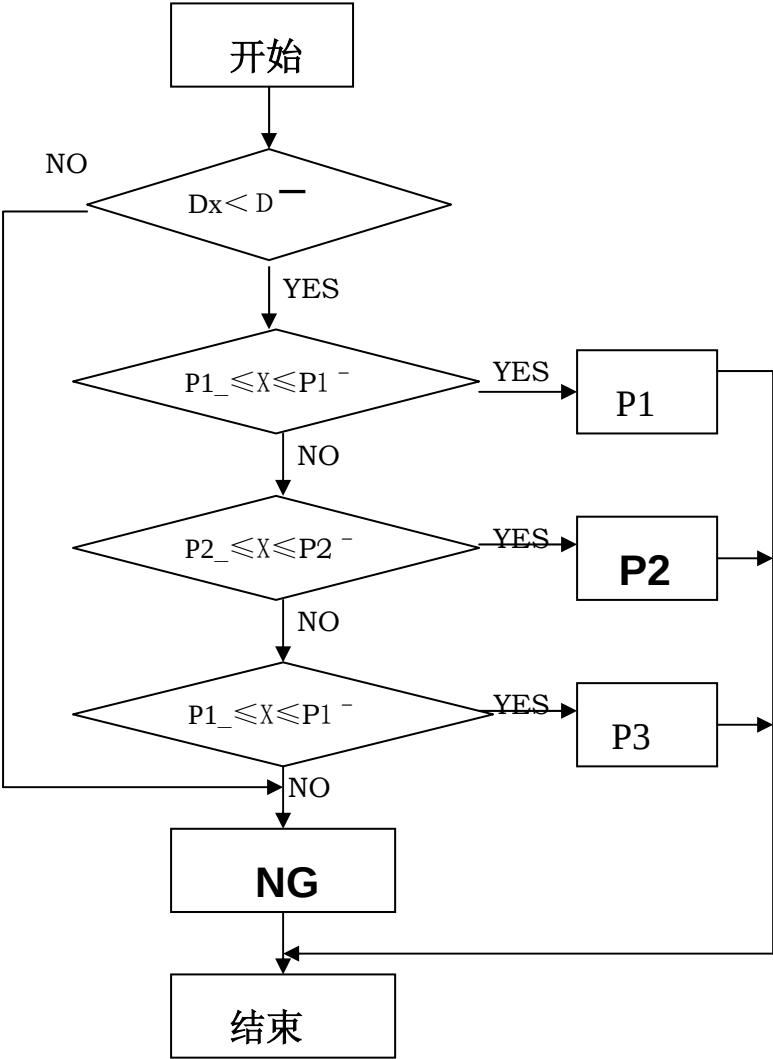
图 2-6A 分选判别流程
