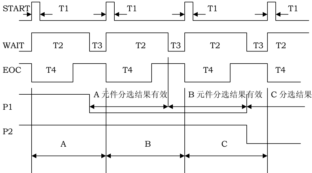
图 2-9 HANDLER 接口工作时序
