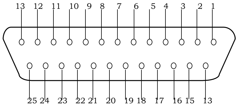
图 2-10 打印接口引脚示意图
