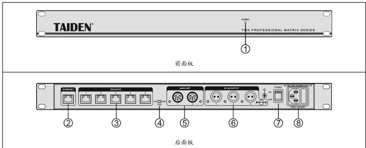
图 6.6.1 HCS-8300KMx2 会议专用千兆网交换机
