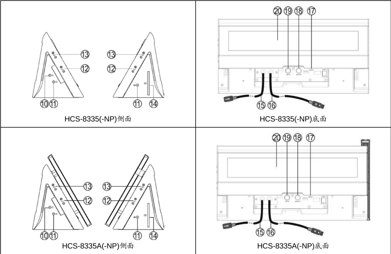
图 3.4.1 HCS-8335 系列经济型多媒体会议终端
