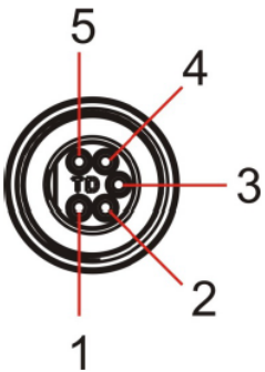
MIC-SK-V 和 MIC-SK-H 引脚定义
