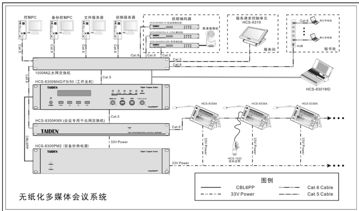
图 6.8.1 HCS-8338 系列无纸化多媒体会议系统连接图
