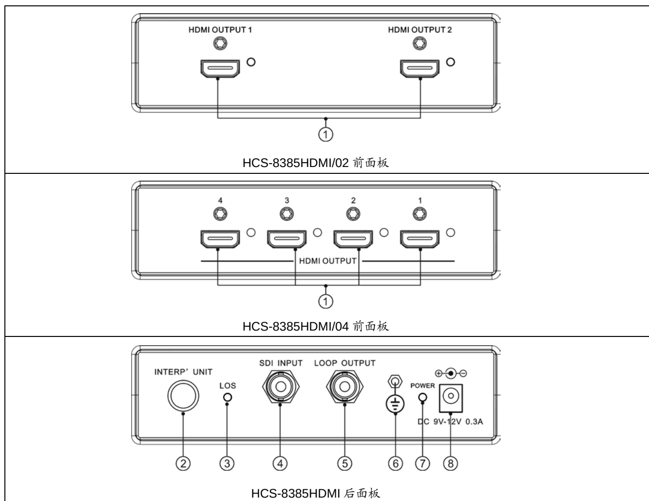
图 4.2.9 HCS-8385HDMI 视频转换器
