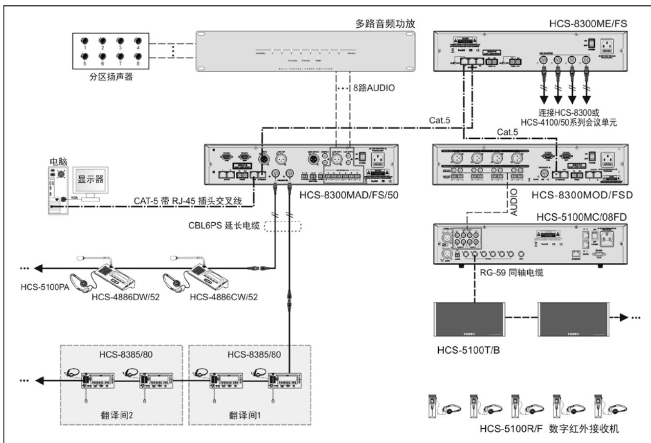
图 5.1.4 会议系统主机通过 HCS-5100MC/F 连接数字红外语言分配系统
