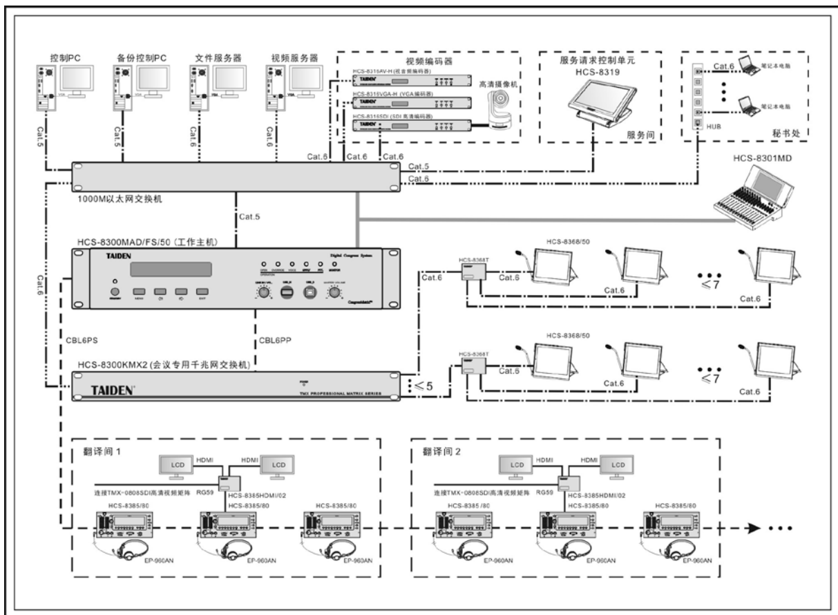
图 6.6.2 HCS-8368/50 系列台式无纸化多媒体会议系统连接图 (PoE 供电)
