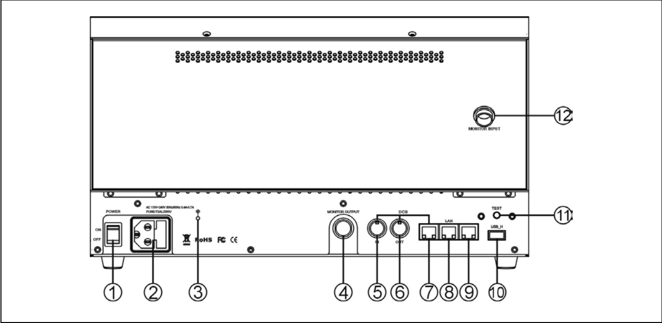
图 6.11.2 HCS-8301 系列数字调音台后面板
