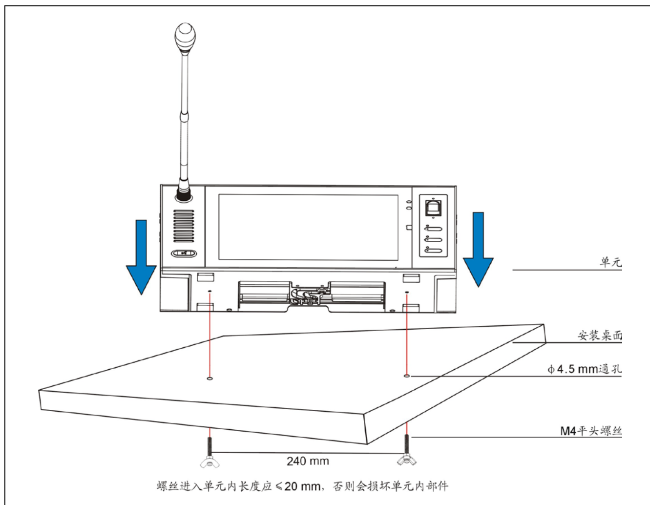
图 3.3.2 HCS-8338 系列无纸化多媒体终端的桌面固定安装
