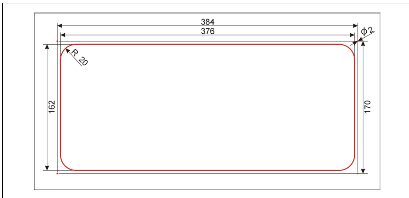
图 3.3.3 HCS-8338/FM 系列无纸化多媒体终端的桌面开孔图（单位：mm）
