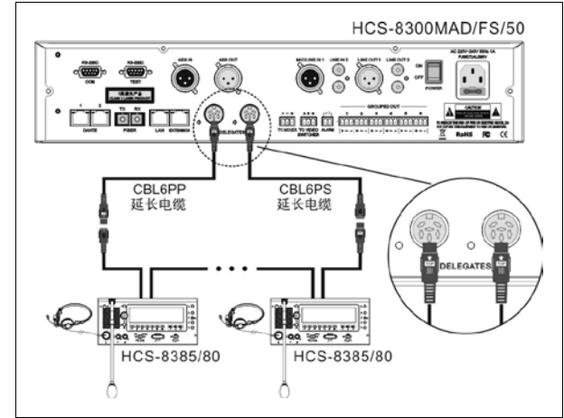
图 4.2.4 会议控制主机与 HCS-8385/80 翻译单元环形连接
