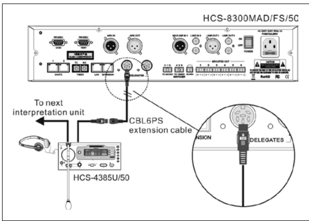
图 4.1.3 HCS-4385U/50 翻译单元与会议控制主机或扩展主机的连接
