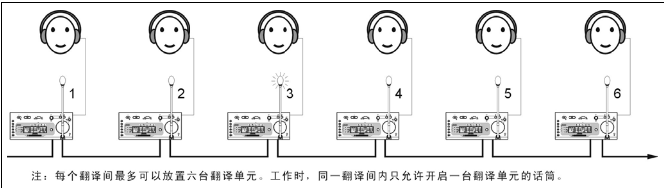
图 4.1.8 翻译单元连接示意图
