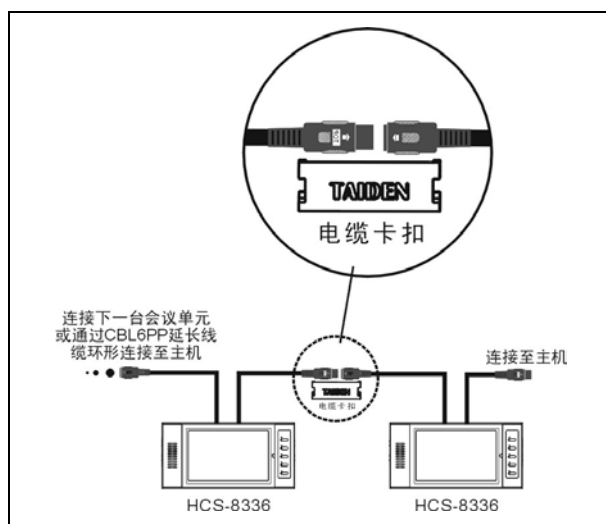
图 3.5.5 HCS-8336 SDI 监视器之间的连接
