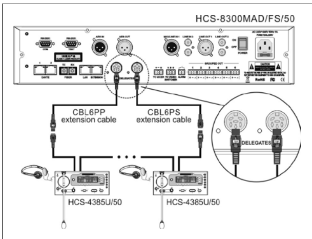
图 4.1.4 会议控制主机与 HCS-4385U/50 翻译单元环形连接
