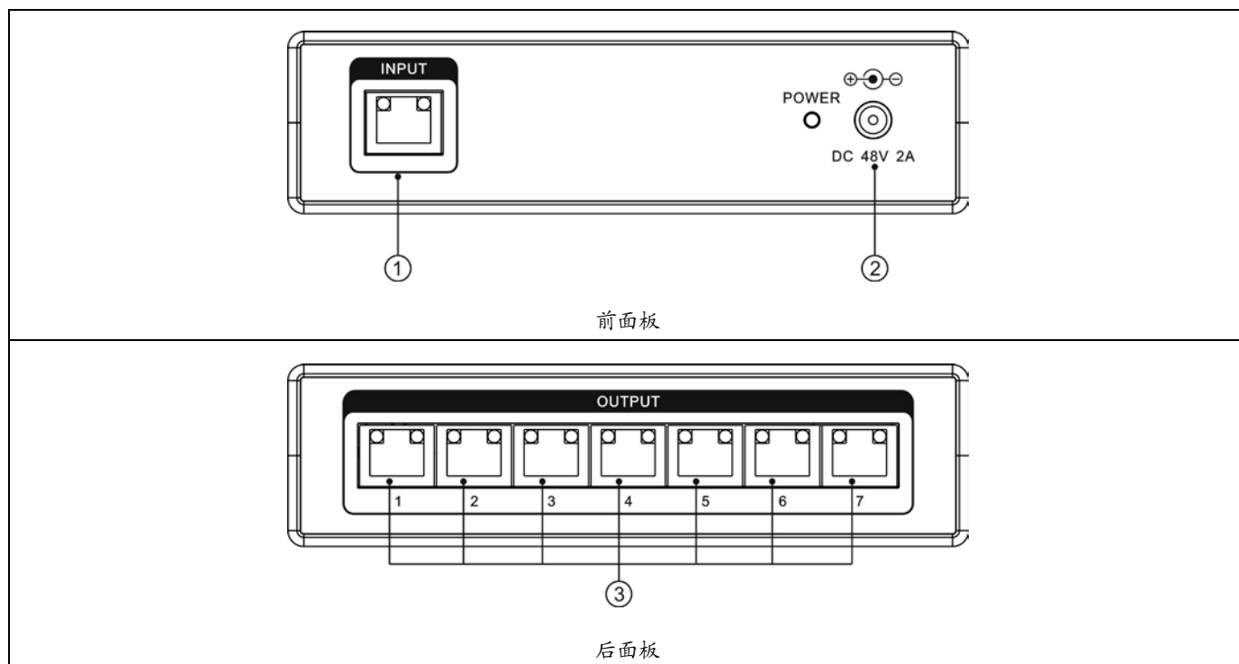
图 6.7.1 HCS-8368T 分配器
