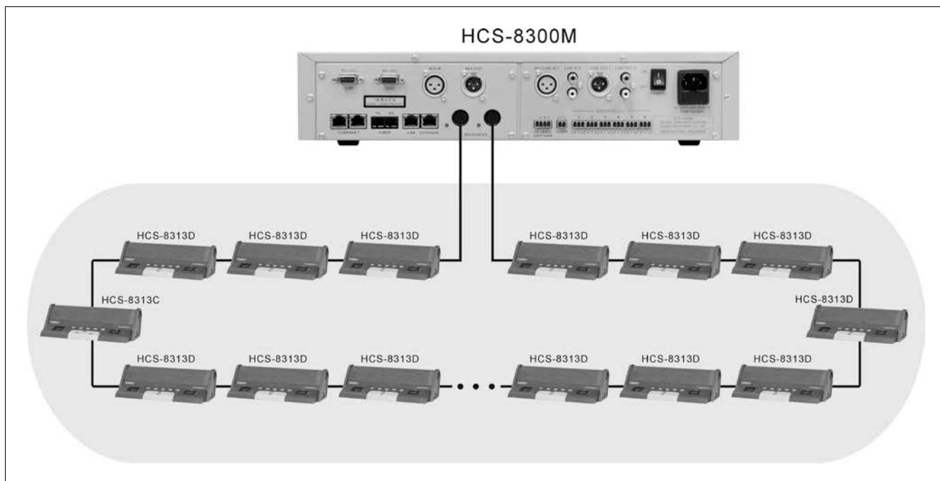
图 1.1.11 “环形手拉手”连接
