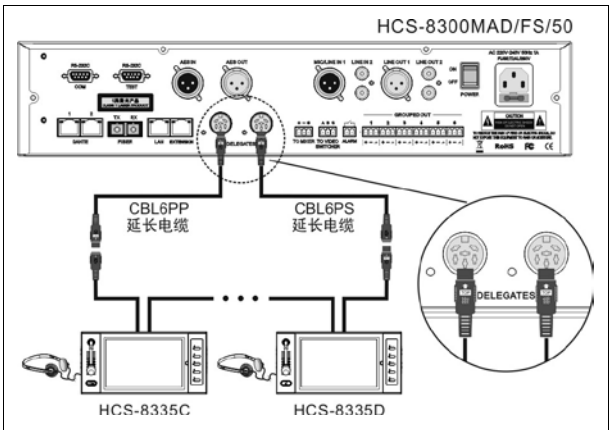
图 3.4.4 会议控制主机与 HCS-8335 系列经济型多媒体终端的环形连接
