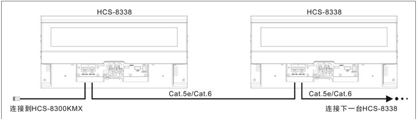
图 3.3.4 HCS-8338/8348 系列无纸化多媒体会议终端之间的连接
