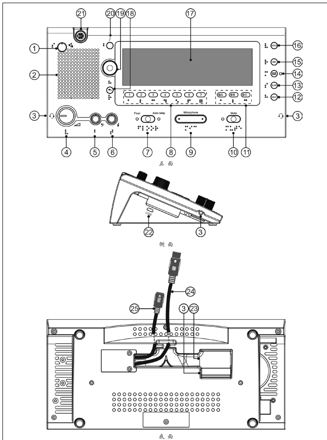
图 4.2.1 HCS-8385/80 翻译单元
