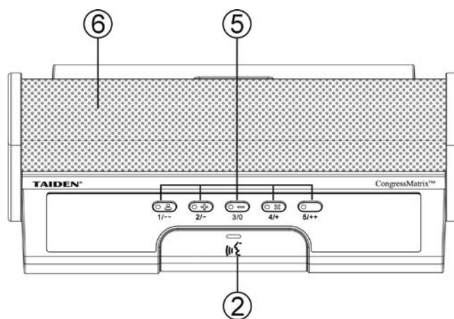
HCS-8314D 代表单元前面板
