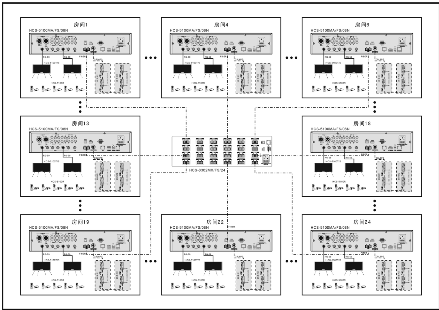
图 6.5.2b 通过 HCS-8302MX/FS 多会议室译员间总控制器拆分、合并多个译员间 (HCS-5100MA/FS/N)
