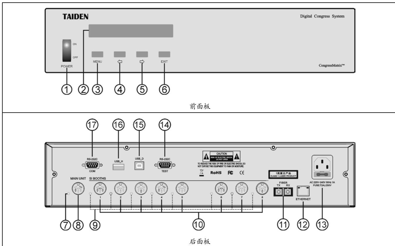
图 6.4.1 HCS-8300MX/FS 多译员间控制器
