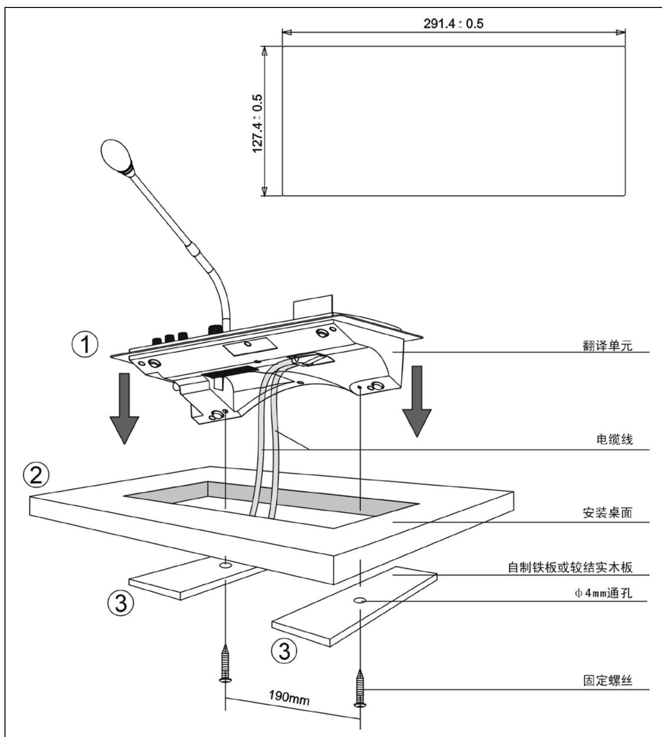
图 4.1.2 HCS-4385U/50 翻译单元嵌入式安装图（单位：mm）
