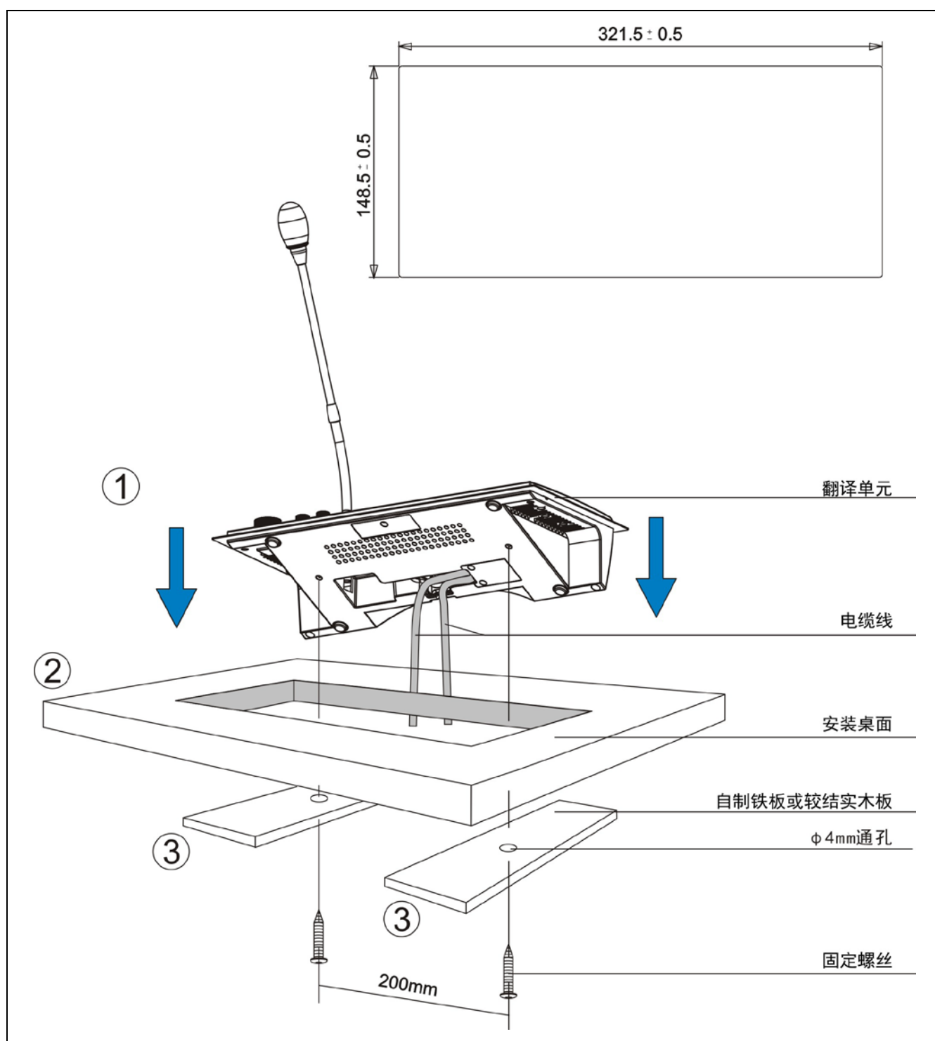
图 4.2.2 HCS-8385/80 翻译单元嵌入式安装图（单位：mm）
