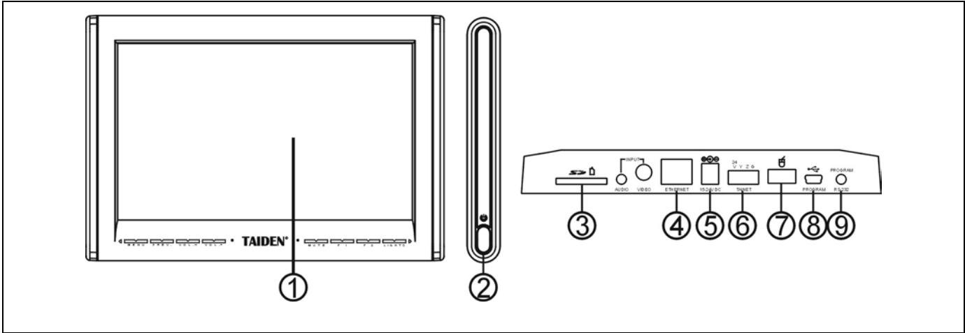
图 6.10.1. HCS-8319 服务请求控制单元
