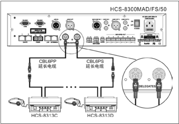
图 3.6.3 会议系统主机与 HCS-8315 系列会议单元的环形连接
