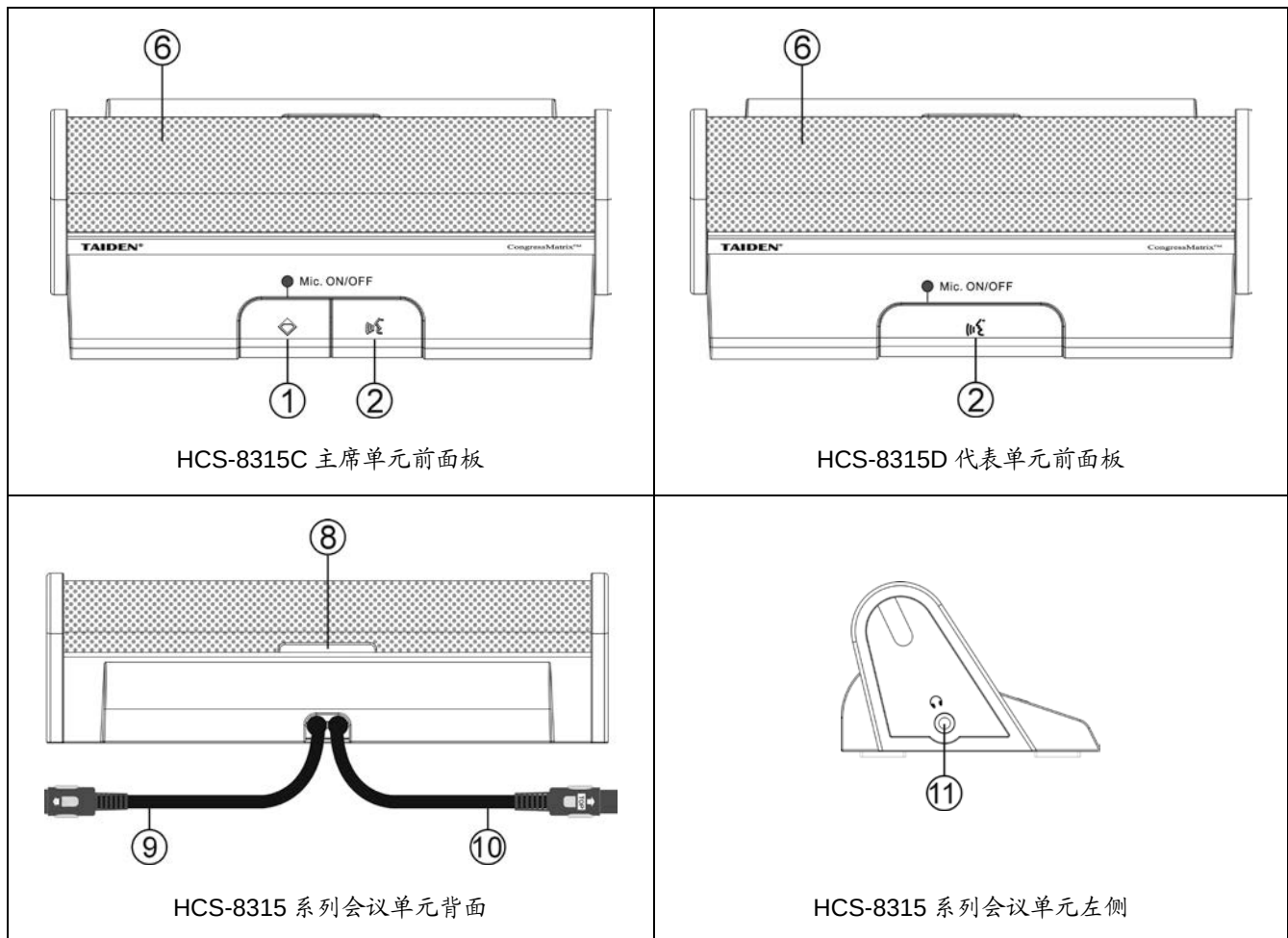
图 3.6.1 HCS-8315 系列会议单元
