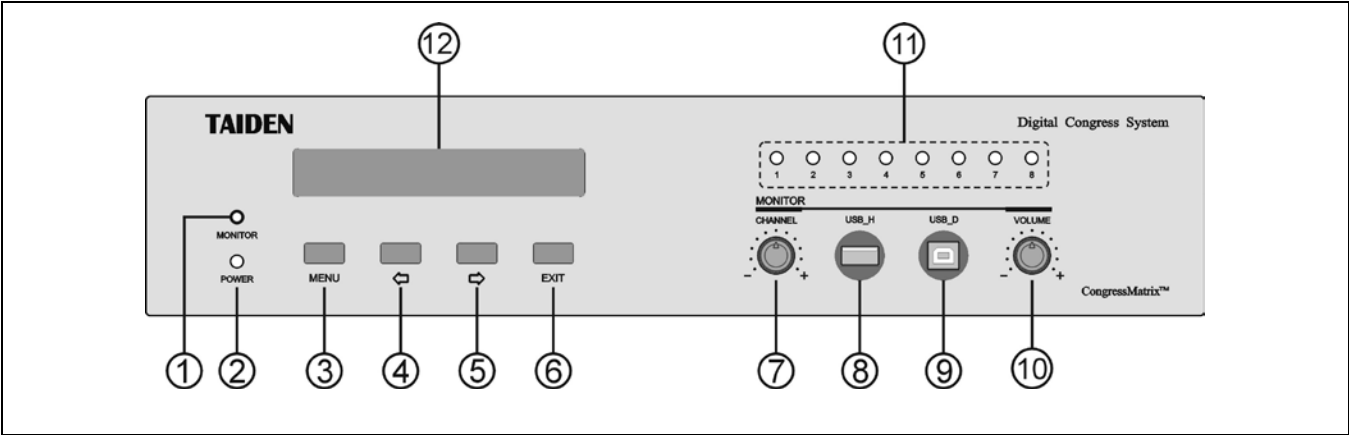
图 6.2.1 HCS-8300MI 8 通道音频输入接口前面板
