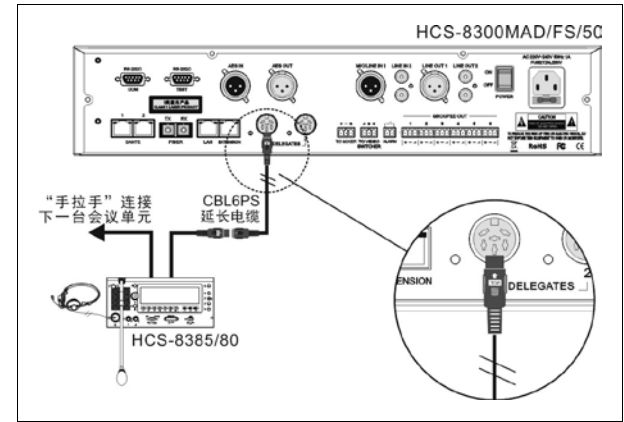
图 4.2.3 HCS-8385/80 翻译单元与会议控制主机或扩展主机的连接
