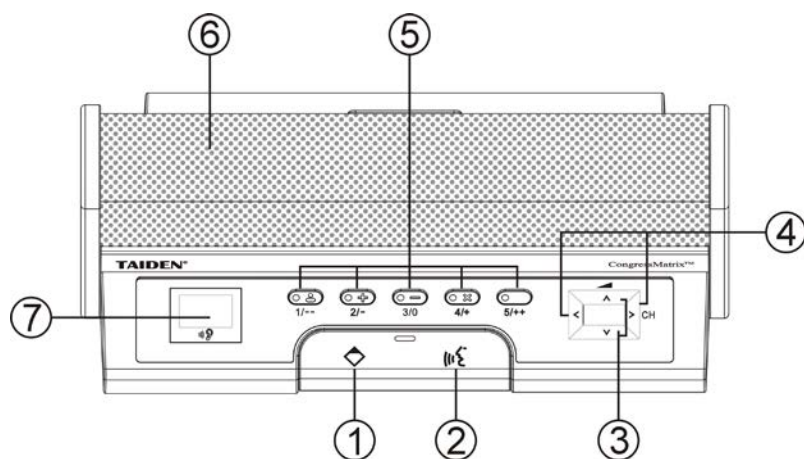
HCS-8313C 主席单元前面板
