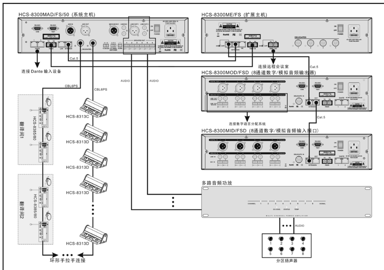
图 1.1.1 系统概览
