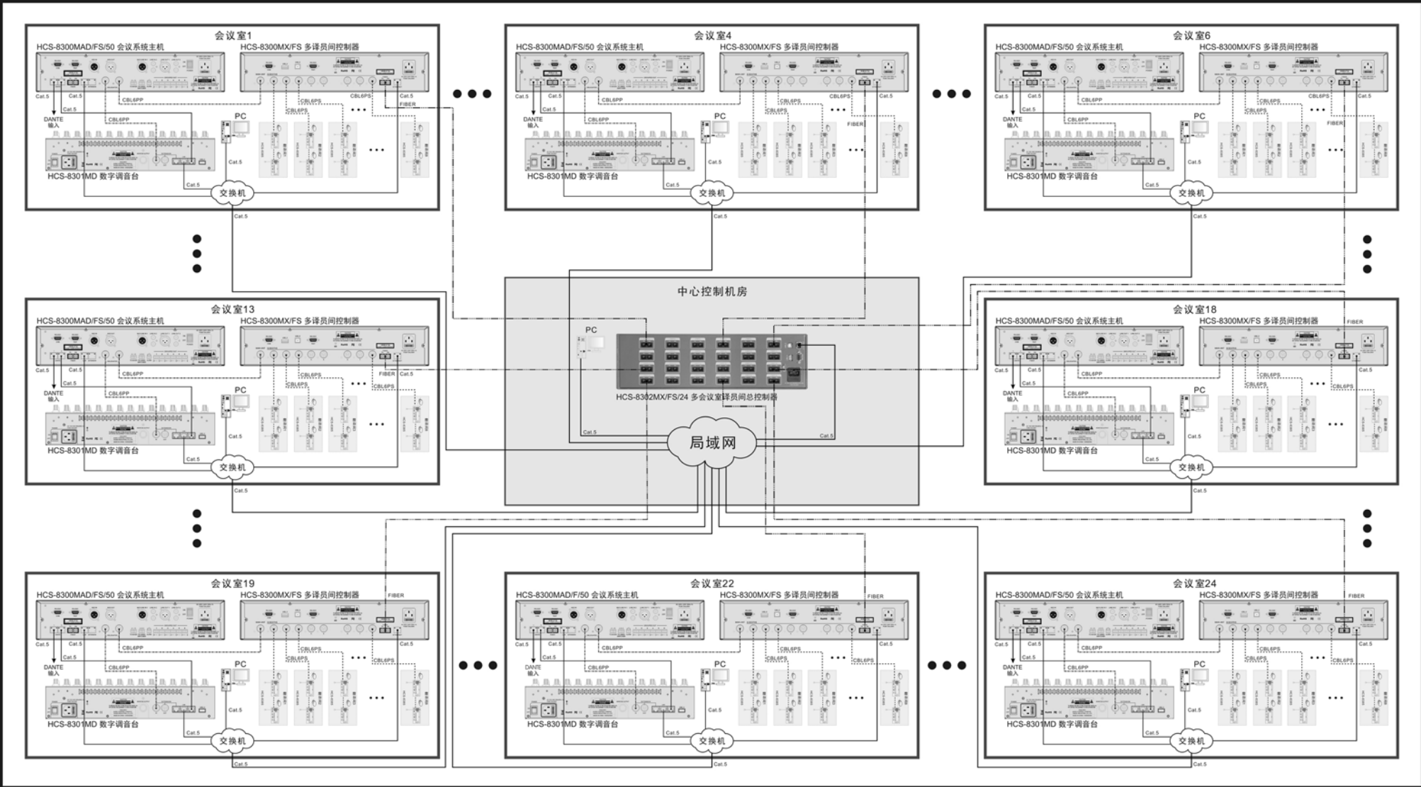
图 6.5.2a 通过 HCS-8302MX/FS 多会议室译员间总控制器拆分、合并多个译员间（HCS-8300MX/FS）
