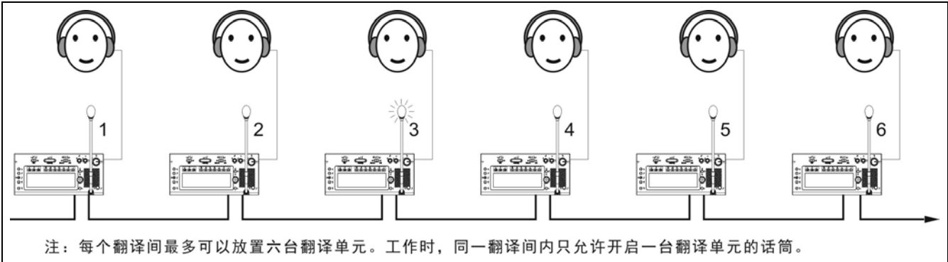
图 4.2.8 翻译单元连接示意图
