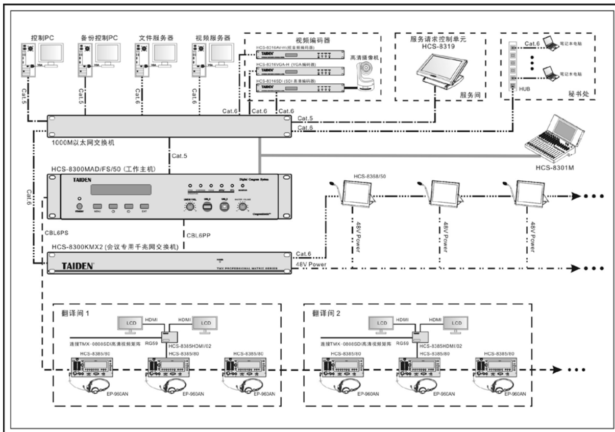
图 6.6.1 HCS-8368/50 系列无纸化多媒体会议系统连接图
