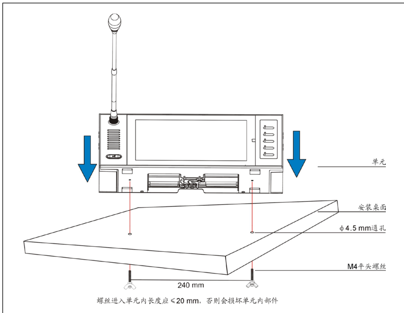
图 3.4.2 HCS-8335 系列经济型多媒体终端的桌面固定安装
