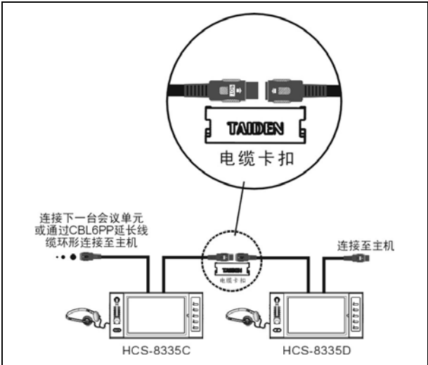
图 3.4.5 HCS-8335 系列经济型多媒体终端之间的连接
