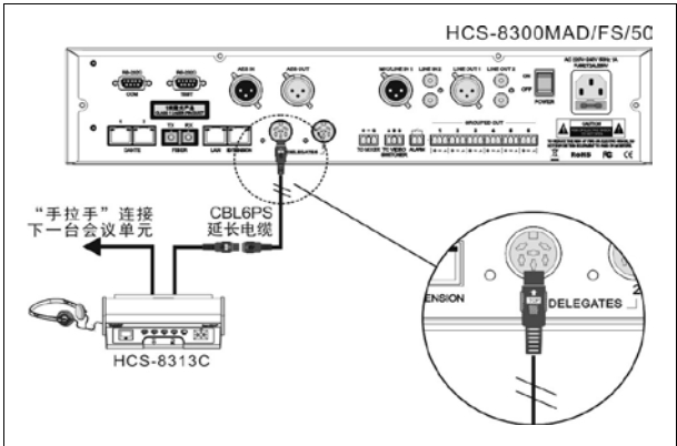
图 3.6.2 HCS-8315 系列会议单元与会议系统主机或扩展主机的连接
