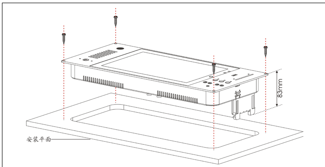
图 3.3.4 HCS-8338/FM 系列无纸化多媒体终端的安装图
