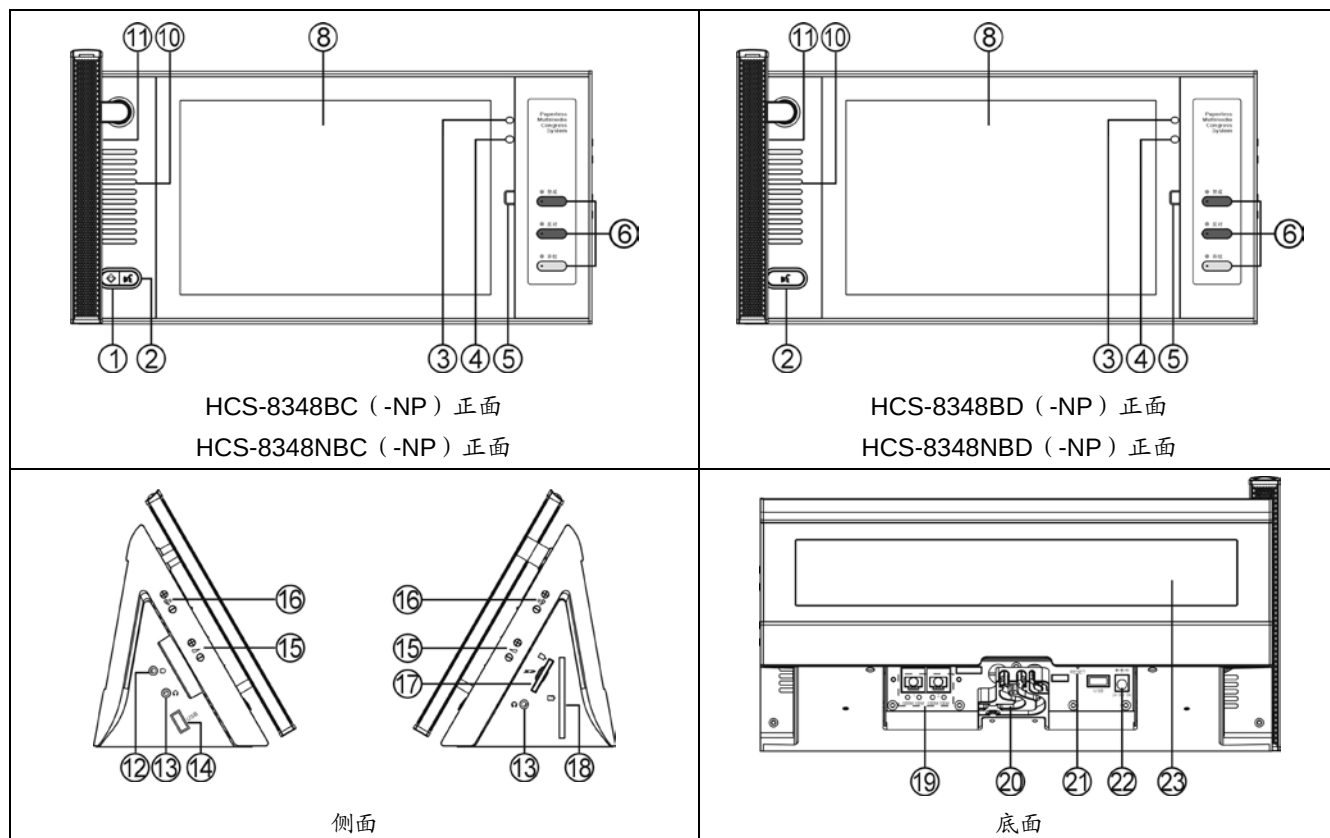
图 3.3.1b HCS-8348 系列无纸化多媒体会议终端
