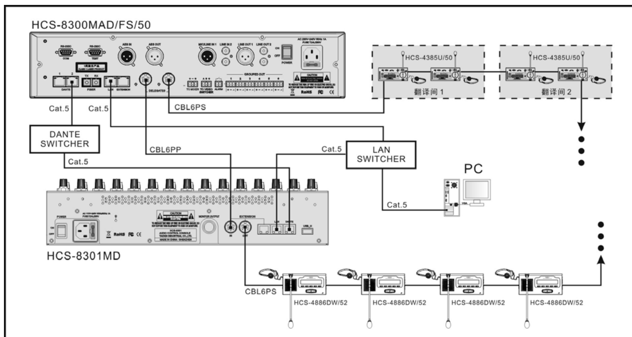
图 6.11.4 HCS-8301M 数字调音台与 HCS-8300MAD/FS/50 会议系统主机的连接
