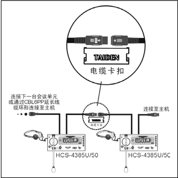
图 4.1.5 翻译单元之间“手拉手”的连接
