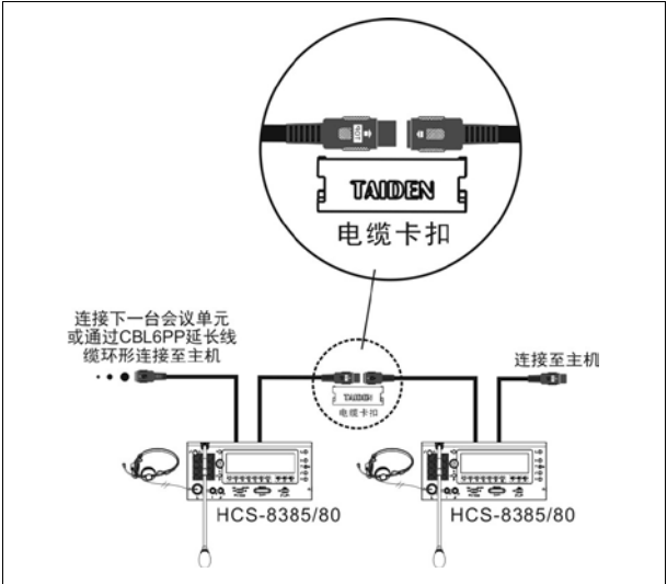
图 4.2.5 翻译单元之间“手拉手”的连接
