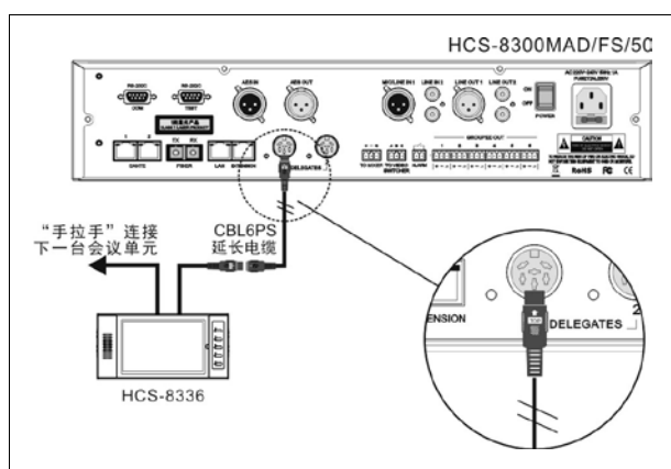
图 3.5.3 HCS-8336 SDI 监视器与会议控制主机或扩展主机的连接
