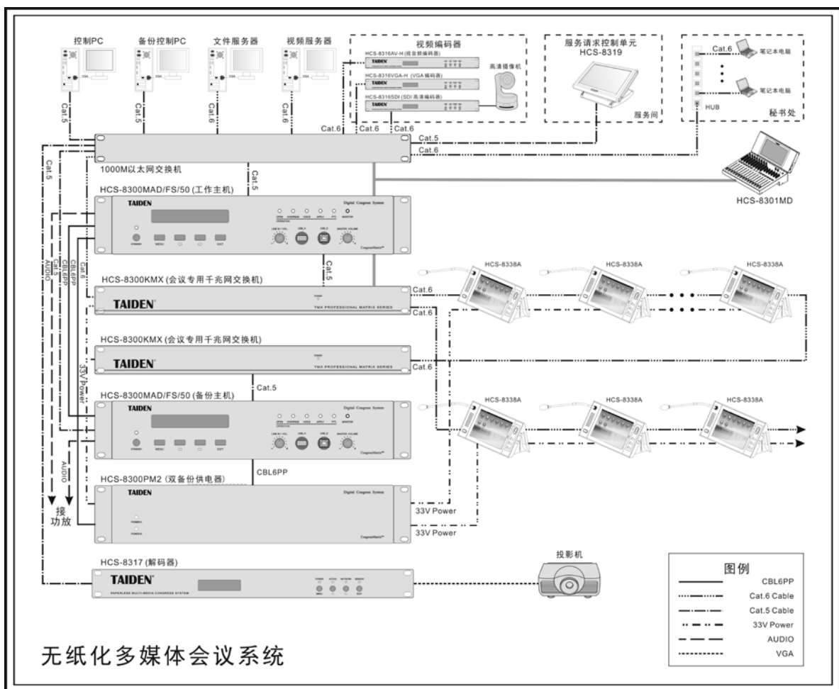
图 6.8.2 HCS-8338 系列无纸化多媒体会议系统连接图（带双机热备份及“环形手拉手”连接）
