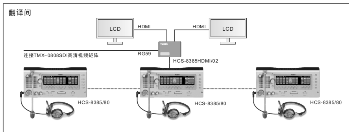
图 4.2.10 全高清翻译间视频解决方案
