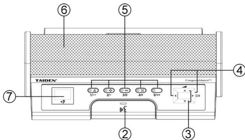
HCS-8313D 代表单元前面板
