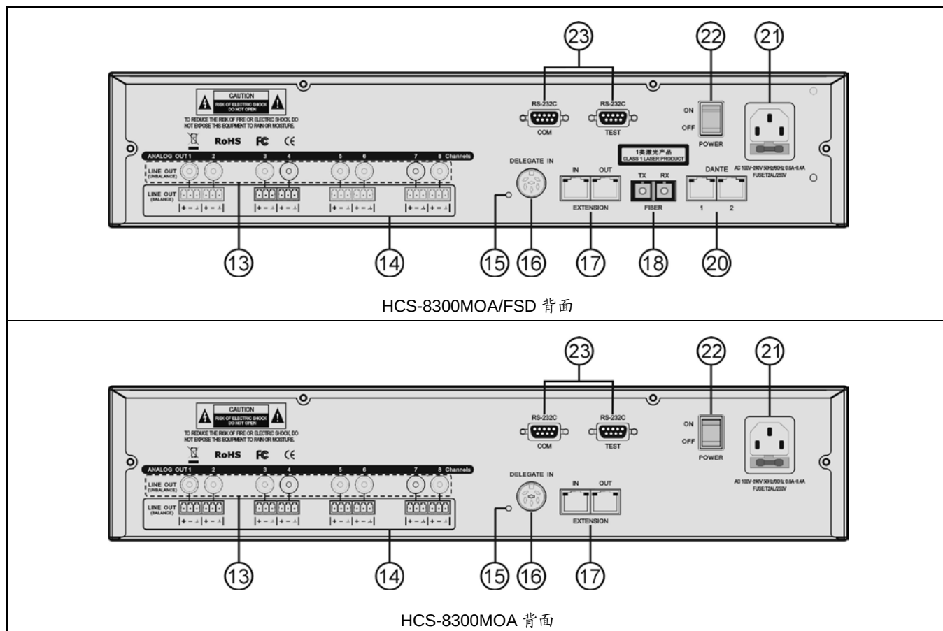
图 6.1.2 HCS-8300MO 8 通道音频输出器后面板
