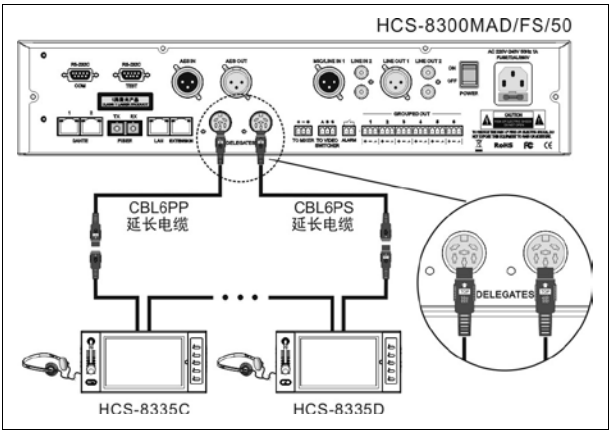
图 2.1.6 会议系统主机与会议单元的环形连接
