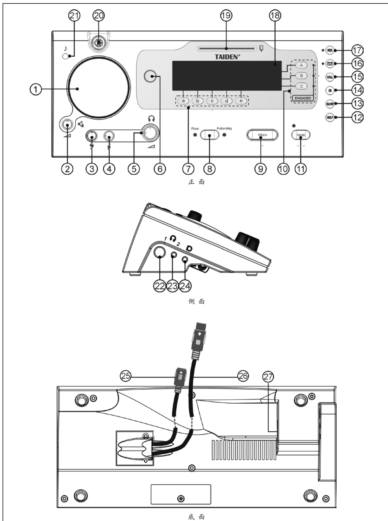
图 4.1.1 HCS-4385U/50 翻译单元
