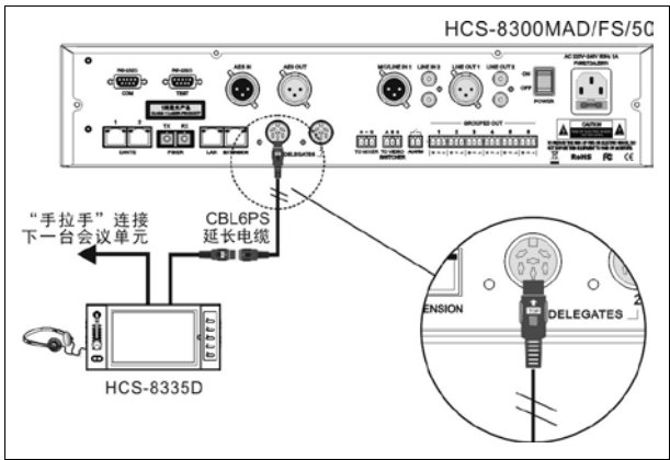
图 3.4.3 HCS-8335 系列经济型多媒体终端与会议控制主机或扩展主机的连接
