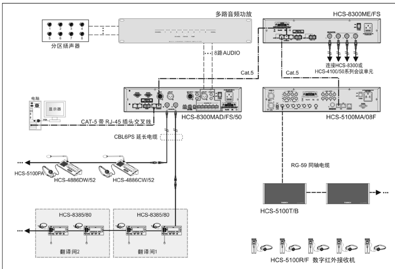
图 5.1.3 会议系统主机通过 HCS-5100MA/F 连接数字红外语言分配系统
