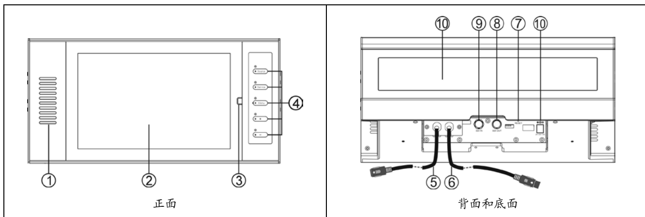
图 3.5.1 HCS-8336 SDI 监视器
