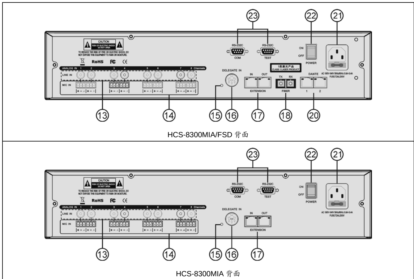
图 6.2.2 HCS-8300MI 8 通道音频输入接口后面板
