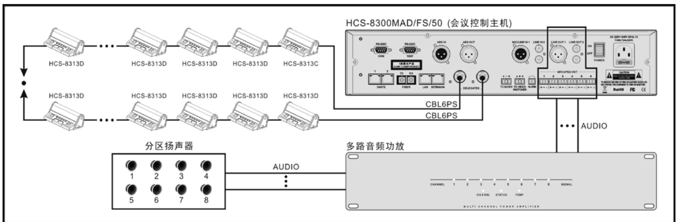
图 5.1.1 会议系统主机与 HCS-8315 系列会议单元之间的连接
