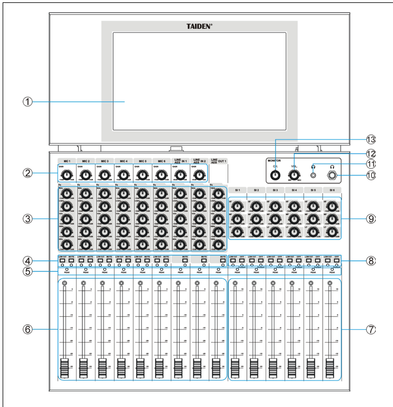
图 6.11.1 HCS-8301 系列数字调音台前面板
