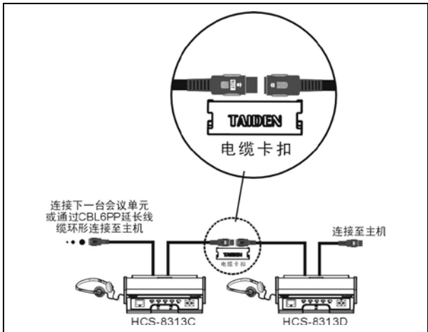
图 3.6.4 HCS-8315 系列会议单元“手拉手”连接
