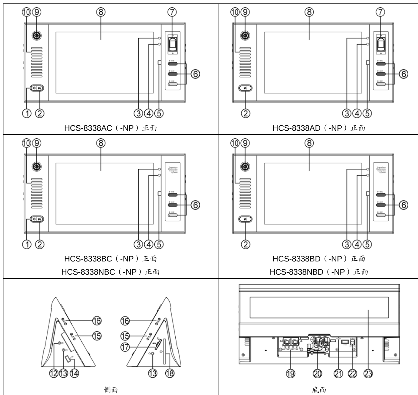
图 3.3.1a HCS-8338 系列无纸化多媒体会议终端
