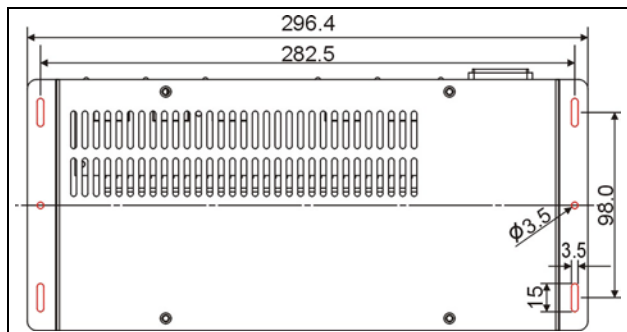
图 2.3.2 会议扩展单元的固定安装
