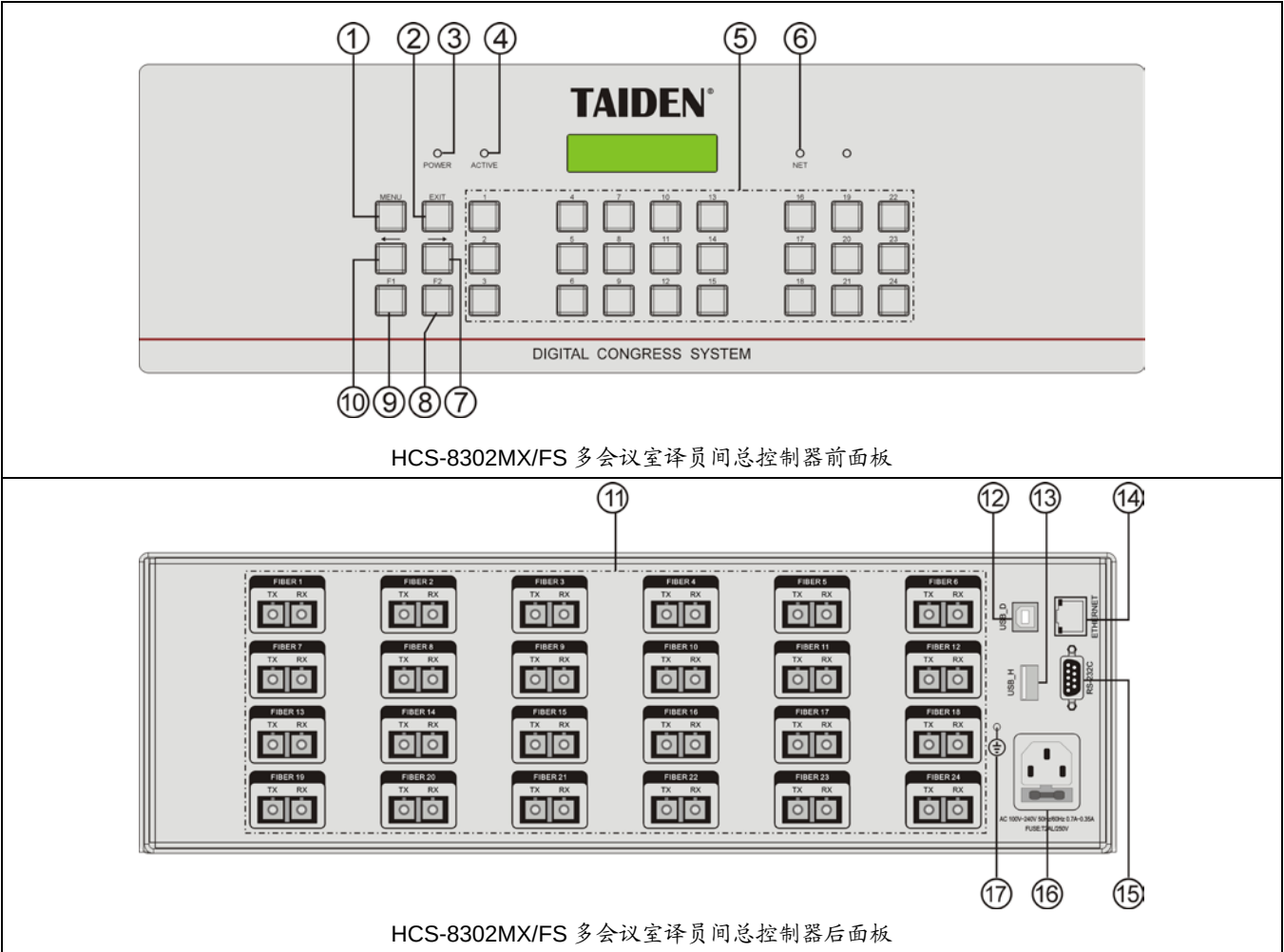
图 6.5.1 HCS-8302MX/FS 多会议室译员间总控制器
