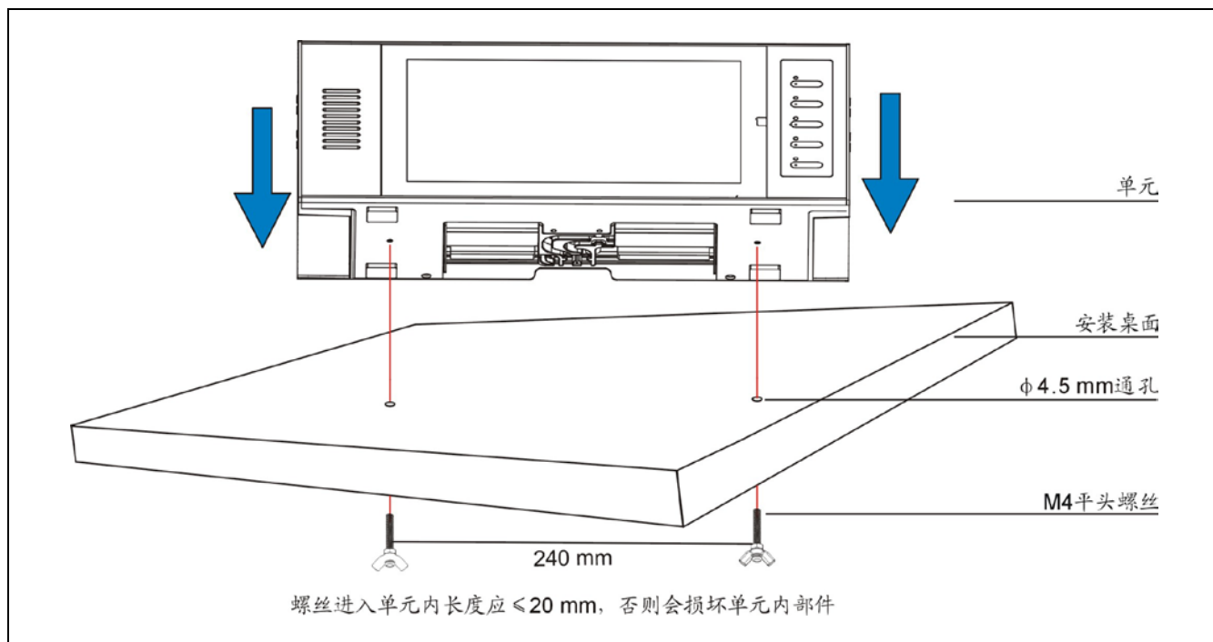
图 3.5.2 HCS-8336 SDI 监视器的桌面固定安装
