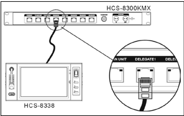
图 3.3.3 HCS-8338 系列无纸化多媒体会议终端与千兆网交换机的连接
