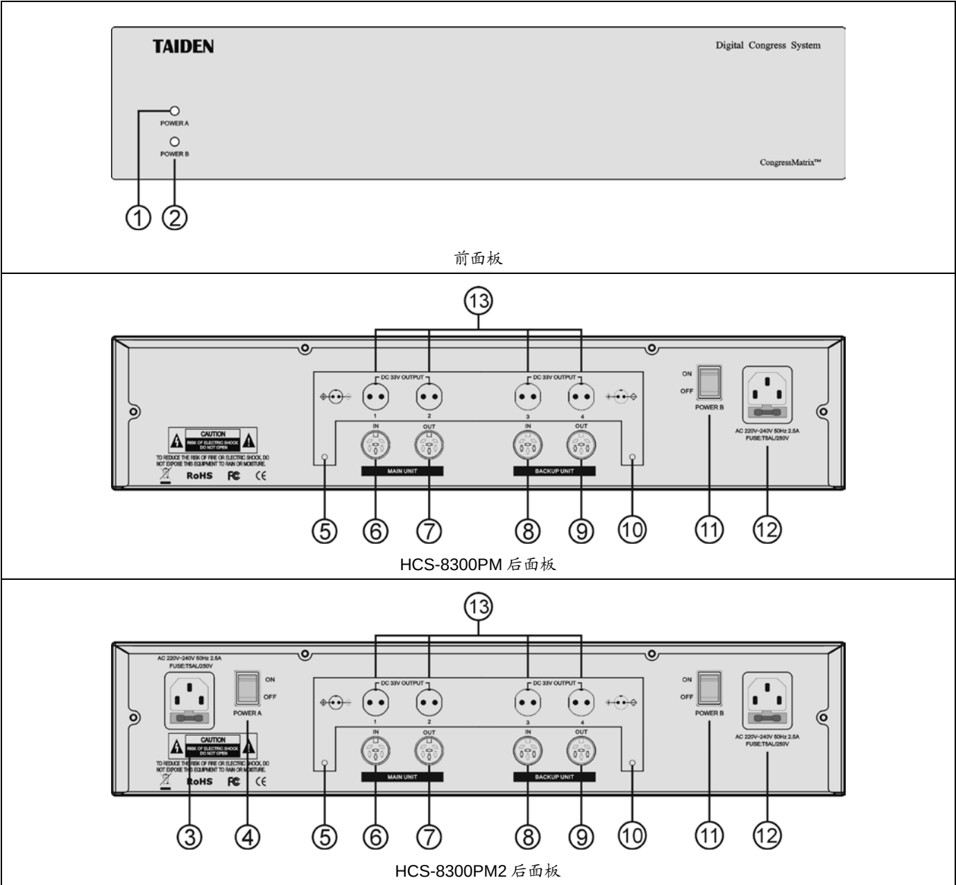
图 6.9.1 HCS-8300PM 会议专用供电
