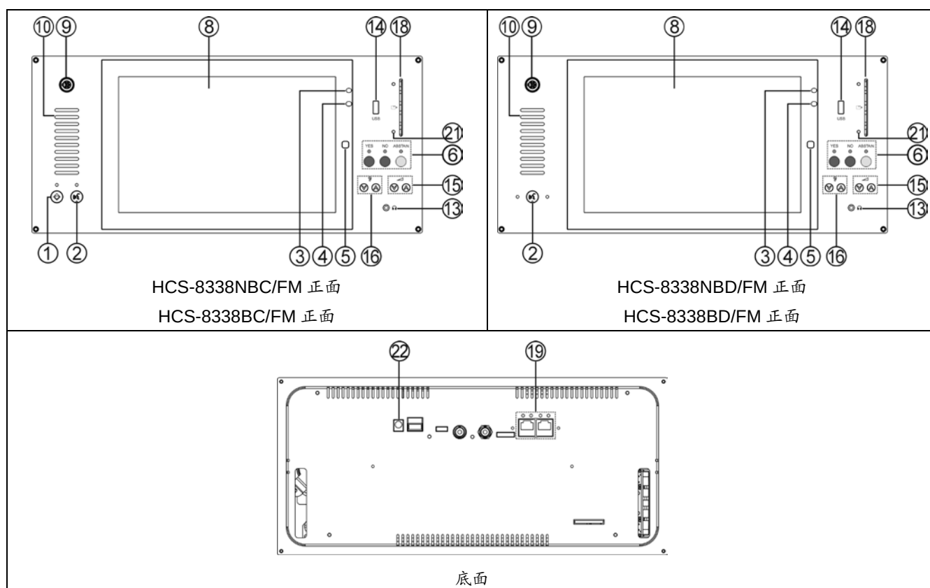
图 3.3.1c HCS-8338/FM 系列无纸化多媒体会议终端
