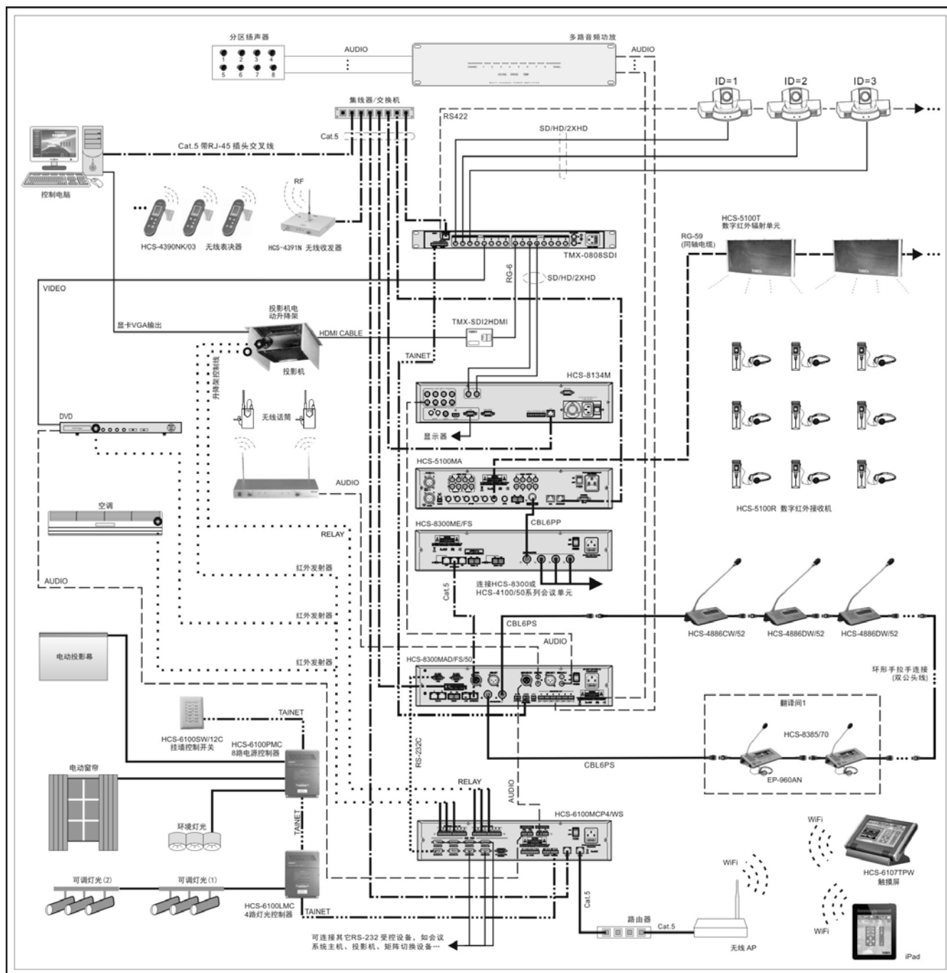
图 5.1.5 会议系统主机与中央控制系统的连接
