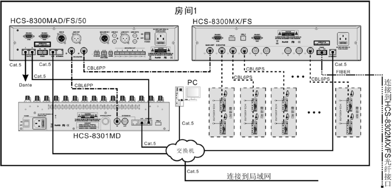
图 6.4.2 HCS-8300MX/FS 多译员间控制器单个会议室的连接
