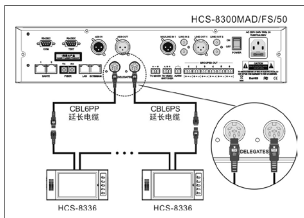
图 3.5.4 会议控制主机与 HCS-8336 SDI 监视器的环形连接
