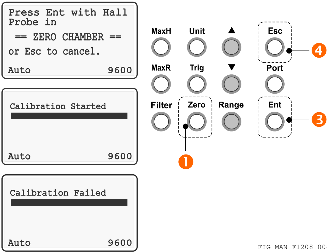
图 3-29 使用 Zero 键进行探头自动校零
