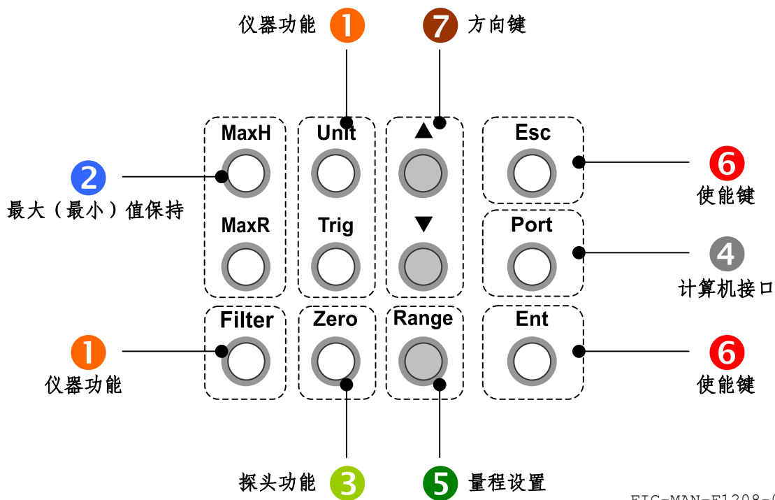
图 3-4 F1208 的键盘分区
