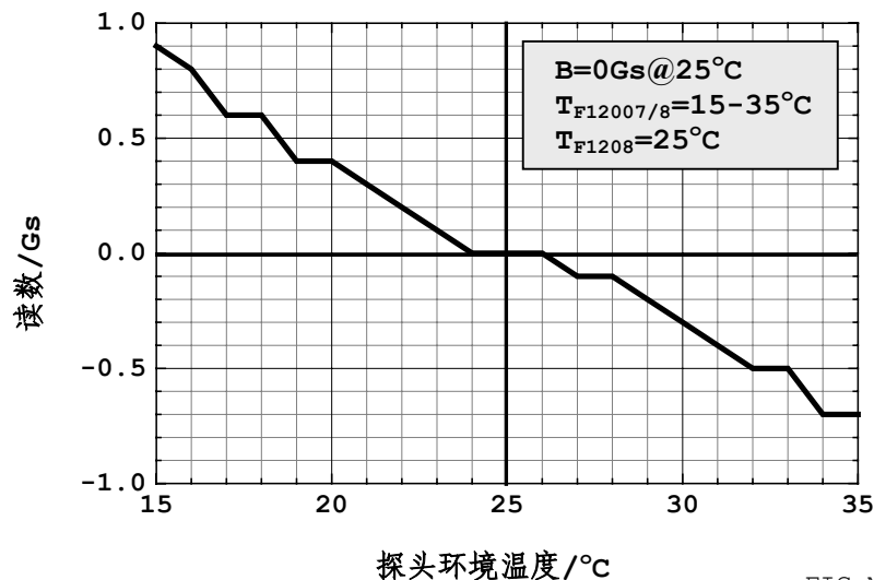
图 5-6 F12007/F12008 的零磁场读数平均温度系数 ZdT
