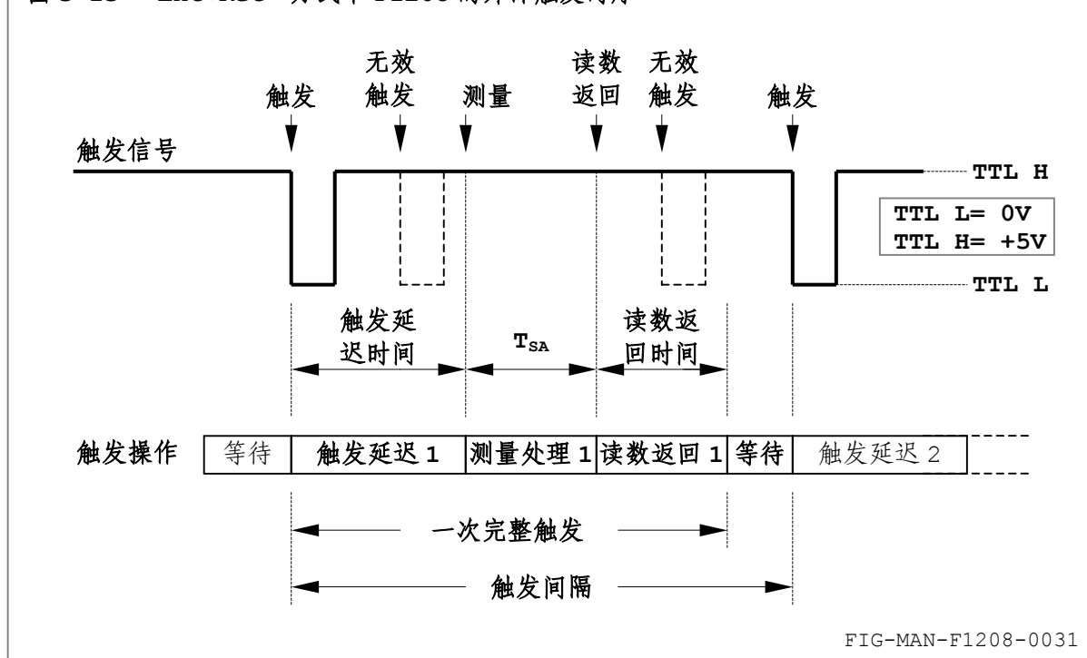
图 3-13 “Ext+Ret” 方式下 F1208 的外部触发时序
