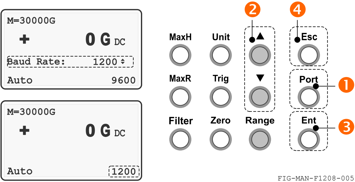
图 3-32 设置波特率
