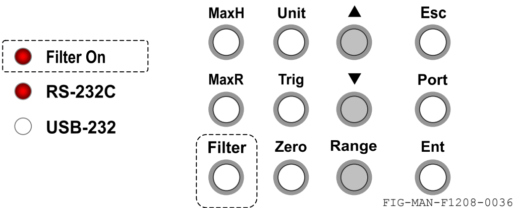
图 3-18 使用 Filter 键开启或关闭显示滤波功能
