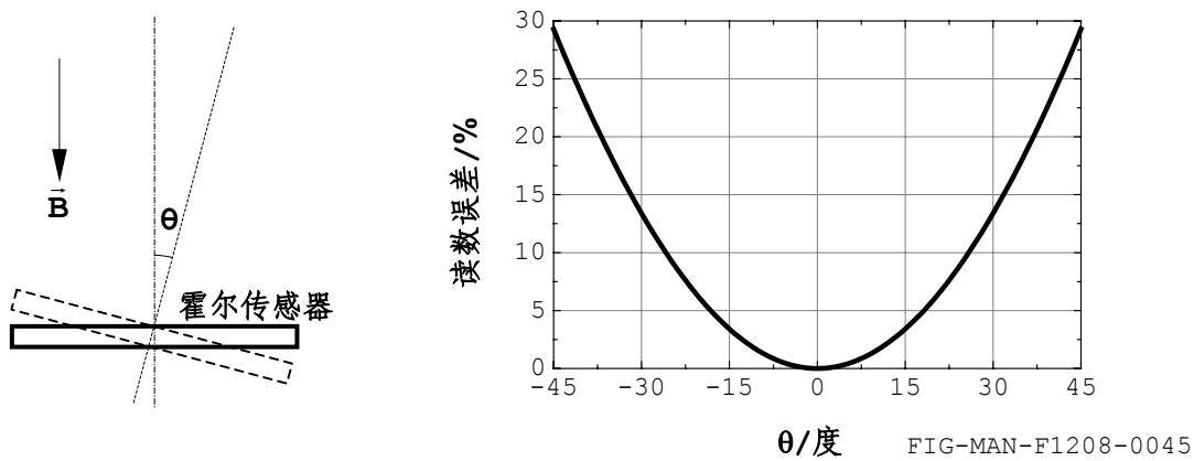
图 3-27 探头读数误差与传感器方向的关系
