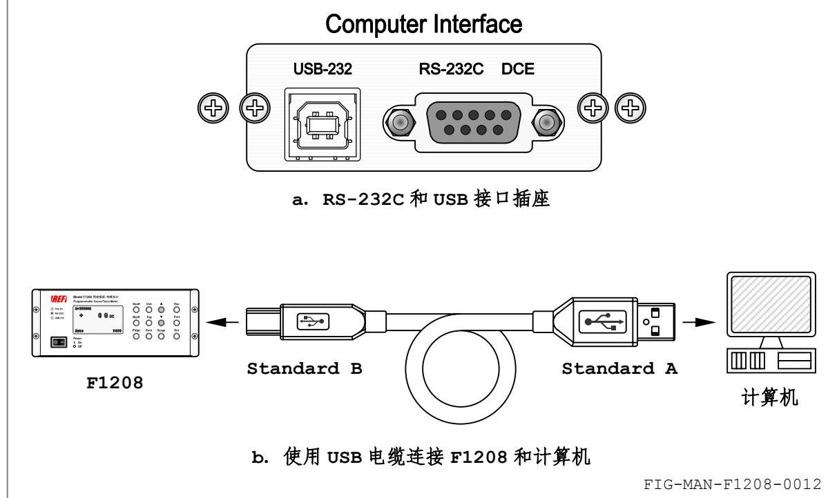
图 2-8 计算机接口连接器以及使用 USB 电缆连接 F1208 和计算机
