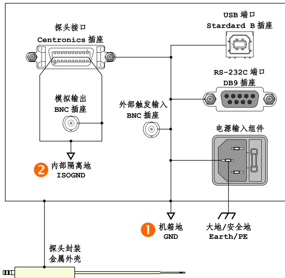
图 3-41 F1208 的接地关系
