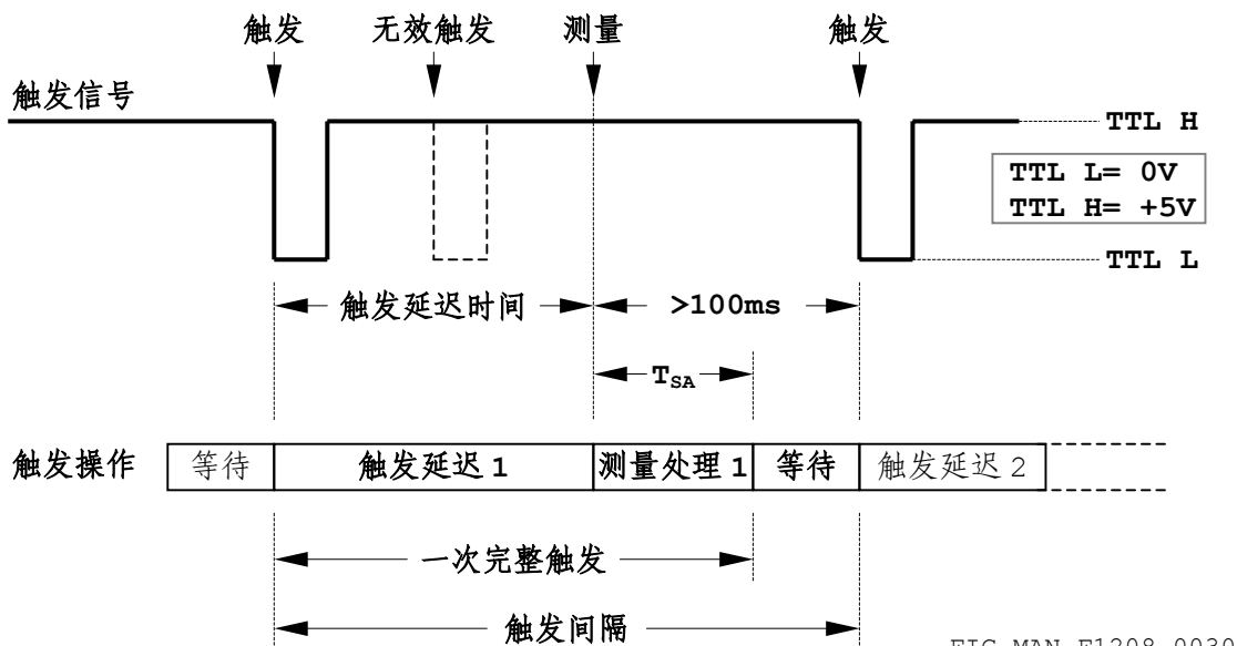
图 3-12 “Ext+Mem”方式下 F1208 的外部触发时序
