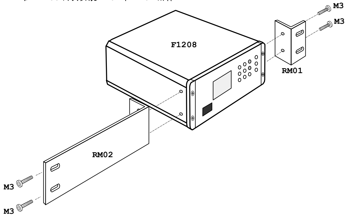
图 2-4 在 F1208 两侧安装 RM01 和 RM02 附件
