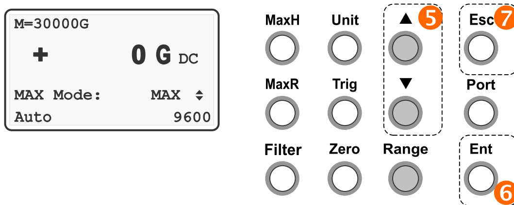
图 3-20 设置最大（最小）值模式
