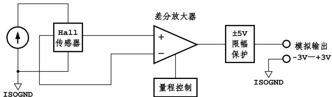
图 3-40 模拟输出电路框图
