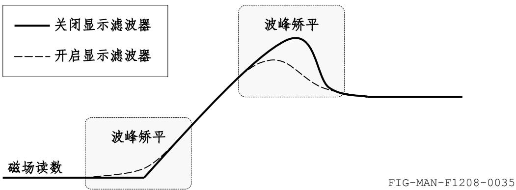
图 3-17 显示滤波器造成的波峰矫平现象
