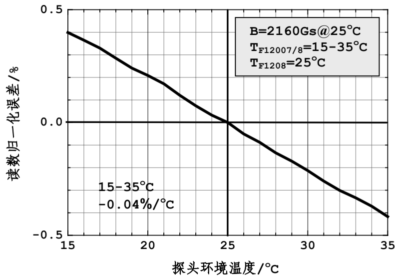
图 5-5 F12007/F12008 的平均温度系数 PdT
