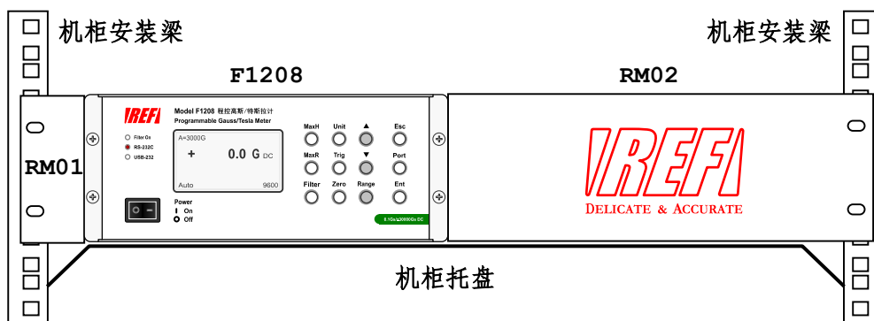
图 2-5 F1208 与机柜的连接安装方法
