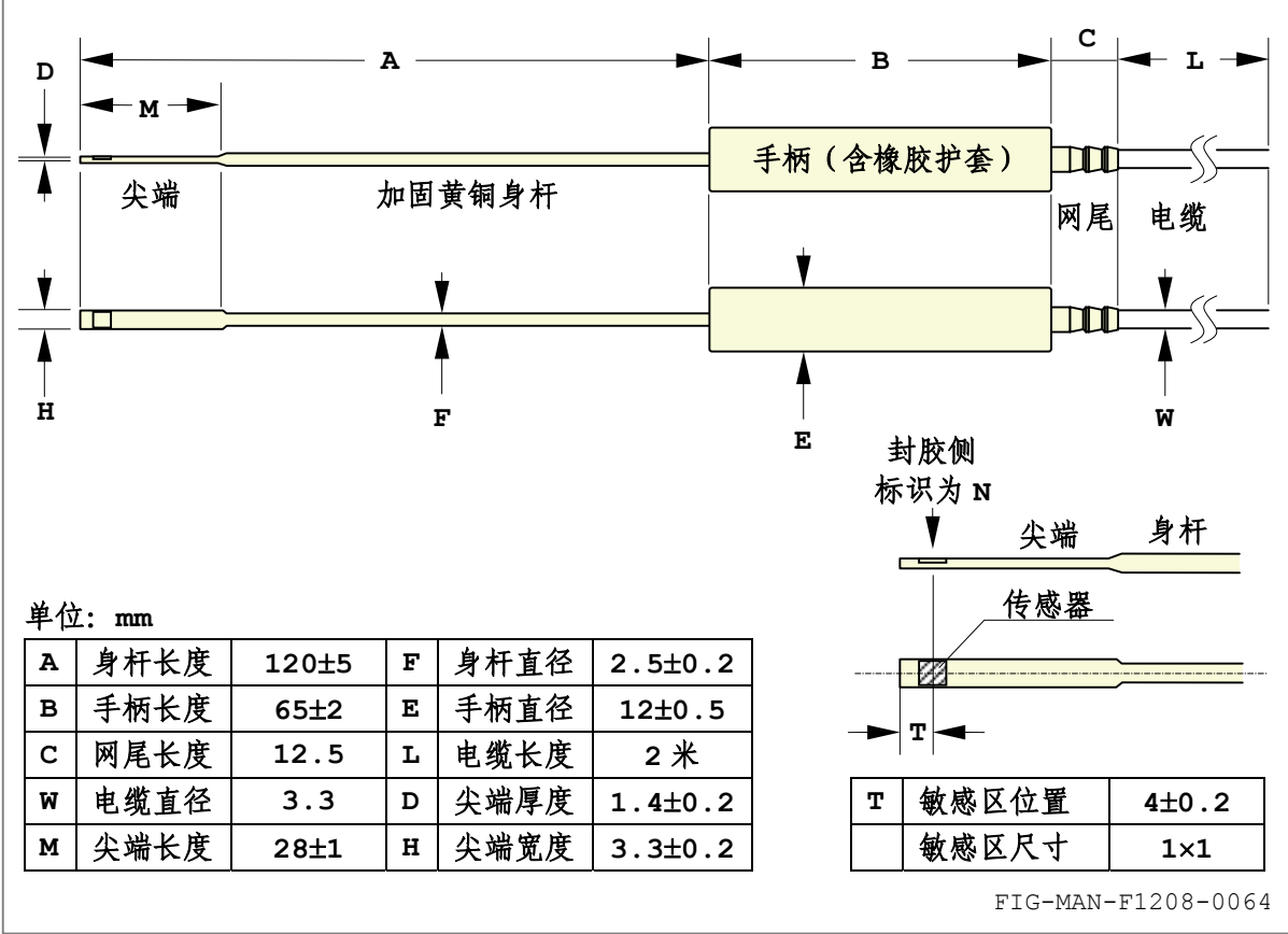
图 5-1 F12007 通用数字化横向霍尔探头二视图
