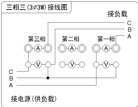
图 4-5 3P3W 接线图
