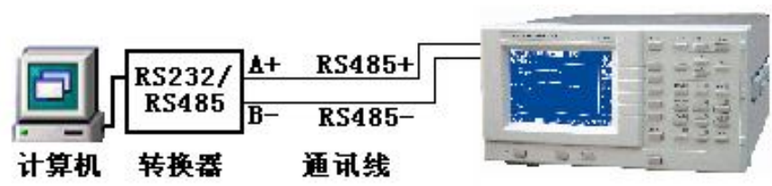
图 16-1 测试仪与计算机通讯—RS485
