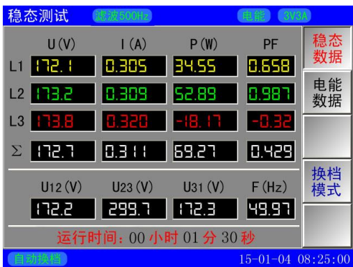
图14-4 滤波后的变频器输出的测量数据
