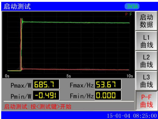
图 11-3 P-F 曲线
