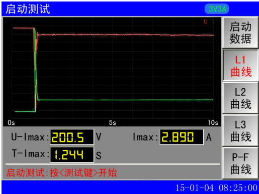
图 11-2 L1 曲线
