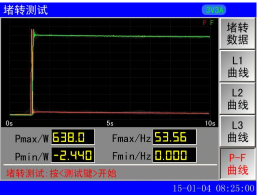
图 12-3 P-F 曲线
