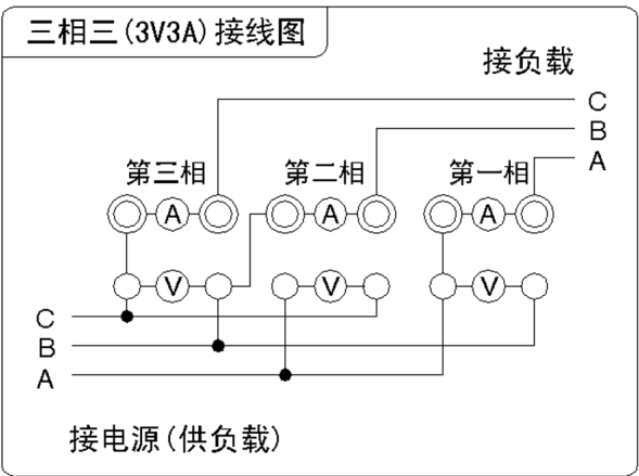
图 4-7 3V3A 接线图
