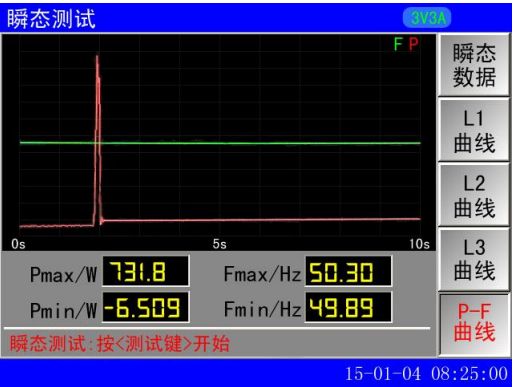
图 9-3 P-F 曲线
