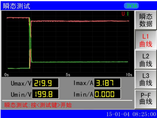
图 9-2 L1 曲线
