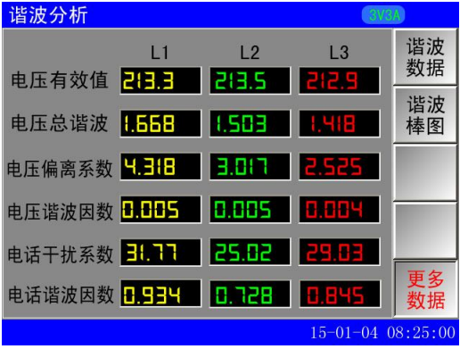
图 7-3 谐波更多数据
