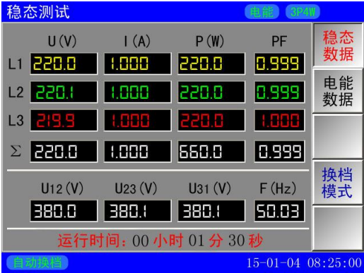
图 5-1 稳态测试
