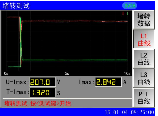
图 12-2 L1 曲线
