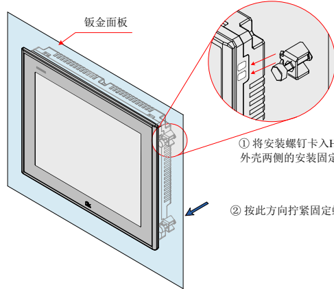
图3 安装示意图
