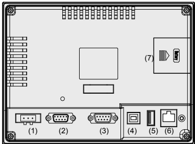
图4 外部接线端子分布及部件介绍
