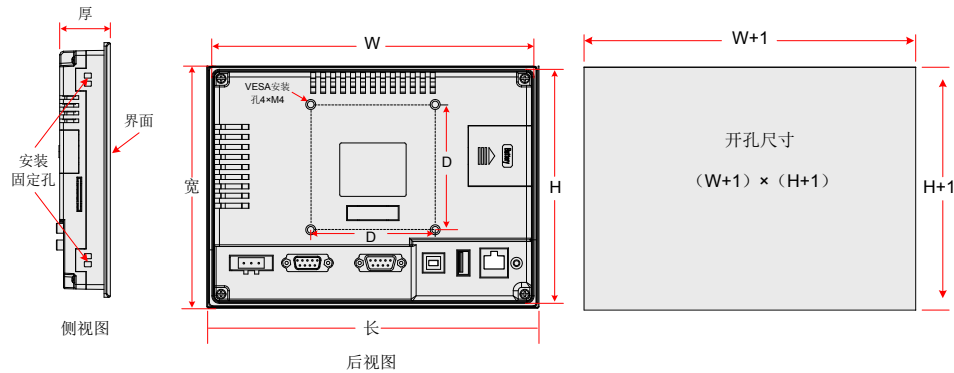
图2 产品尺寸图（单位：mm）
