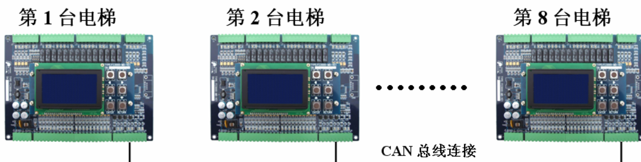
FC3000 系列串行电梯群控系统 CAN 总线接线示意图
