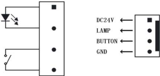
图：3. 3. 3. 3 扩展内选按钮接线图
