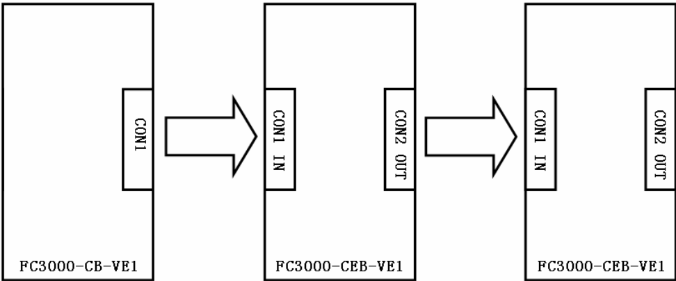
图：3. 3. 3. 2 轿厢控制板与内呼扩展板连接图
