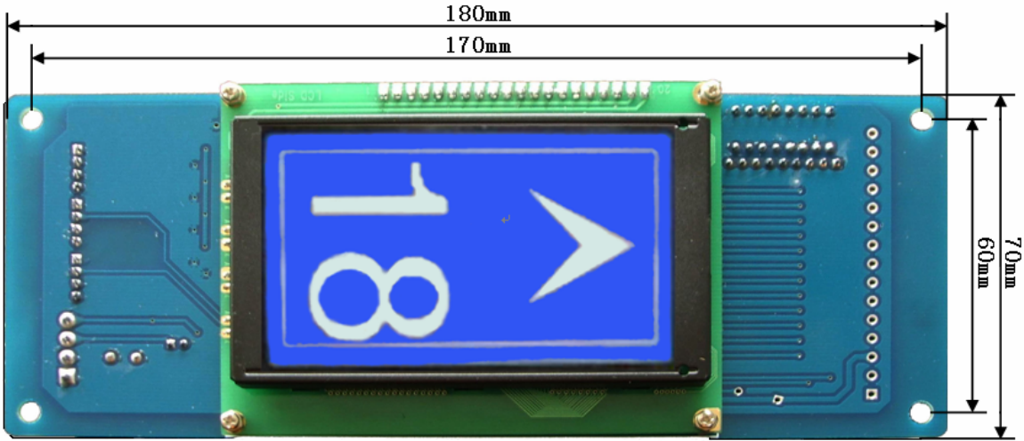
图：3.3.4.3.1 外呼控制板（轿内显示板）ME-LIFT-HC-VE3 外形及安装尺寸
