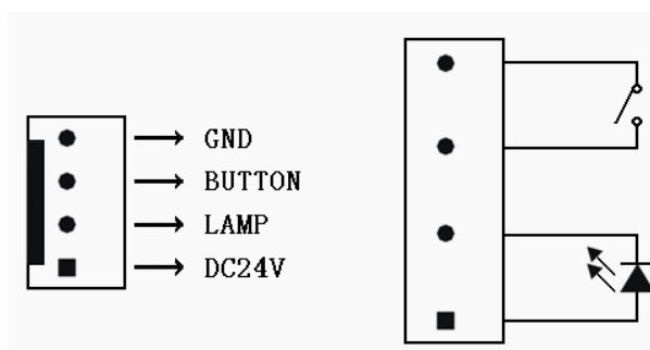
图：3.3.2.2 内选按钮接线图
