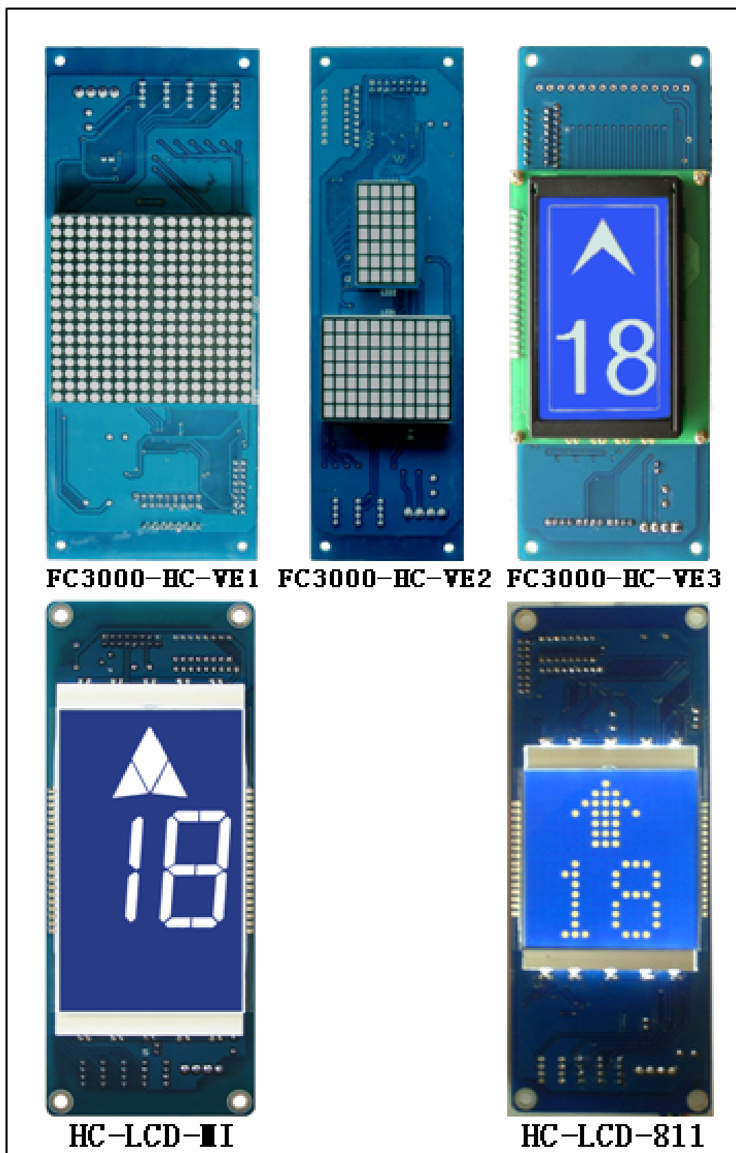
图：3.3.4.1ME-LIFT 系列外呼控制板及轿内显示板产品图片
