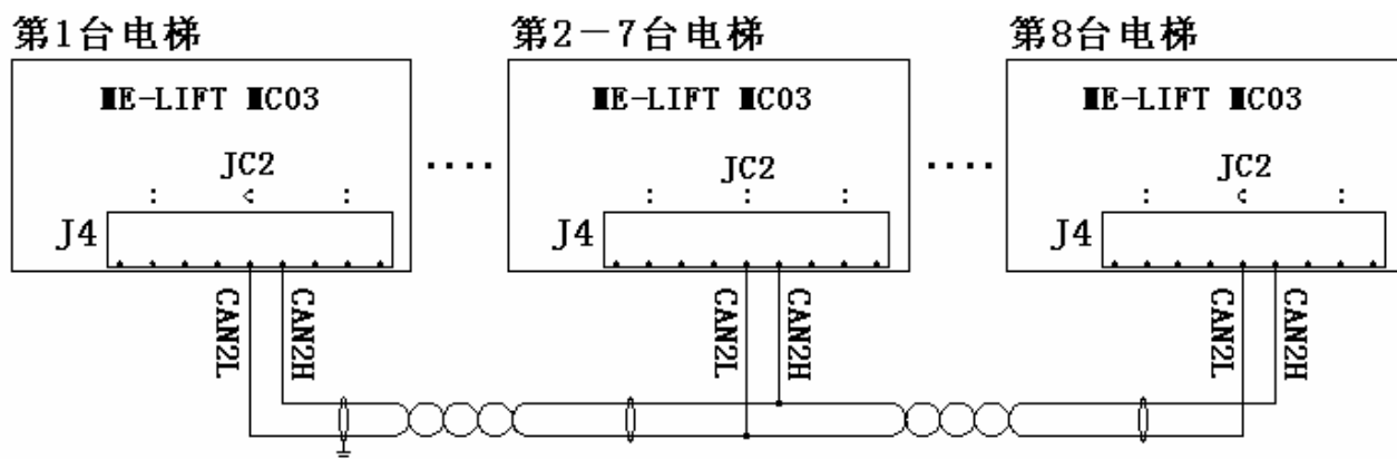
图：7.1.2 ME-LIFT 系列串行控制系统群控 CAN 总线接线示意图
