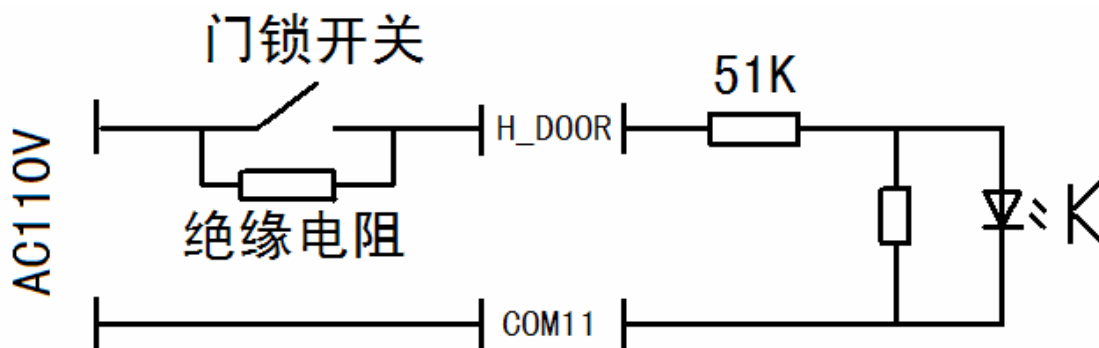
J4 端口外部接线示意图
