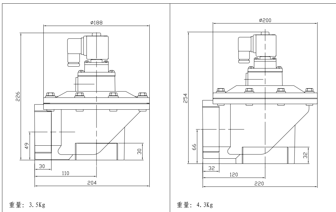
图6. DMF-Z-62S型电磁脉冲阀外形尺寸图
