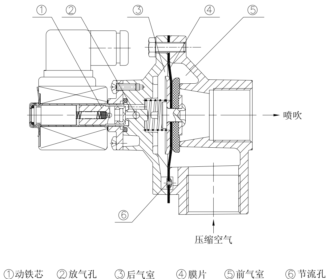
图1. DMF-Z型电磁脉冲阀工作原理图
