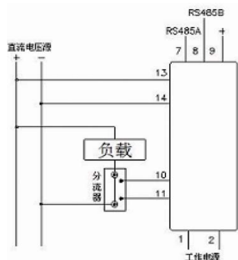
分流器接线方式
