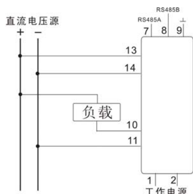
一般接线方式
