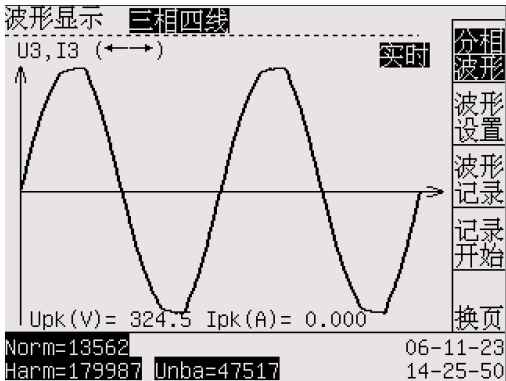
图 6-4 分相电压波形
