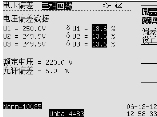
图 9-2 电压偏差屏幕——显示数据
