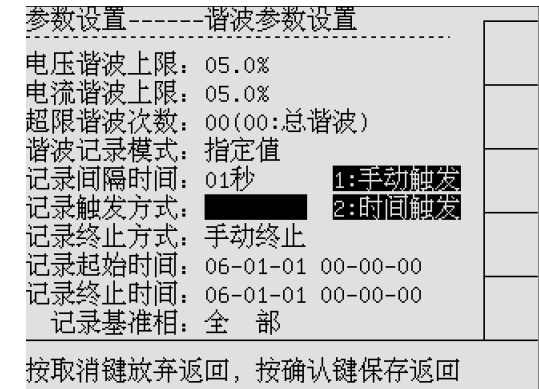
图 11-5 谐波参数—记录触发
