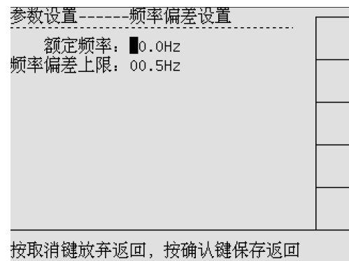
图 10-3 频率偏差屏幕——偏差设置
