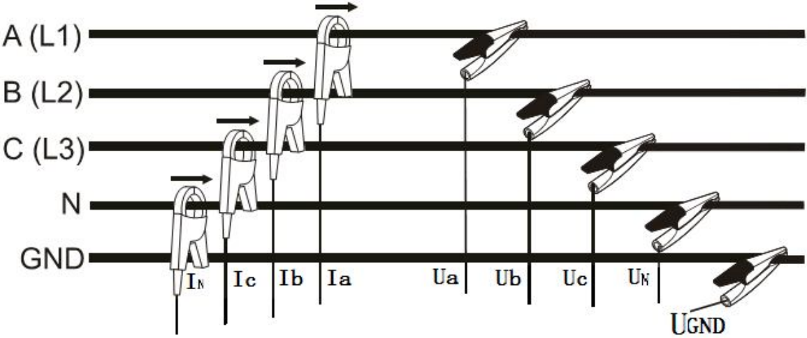
8910C 典型接线示意图——三相四线带地线
