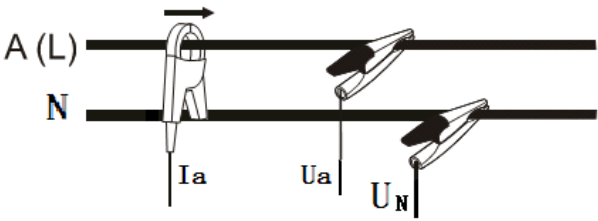
8910C 典型接线示意图——单相
