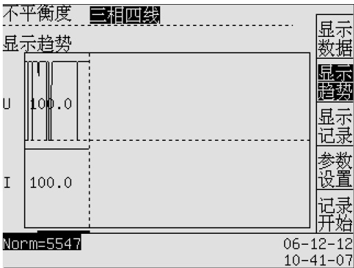
图 8-3 不平衡度—显示趋势
