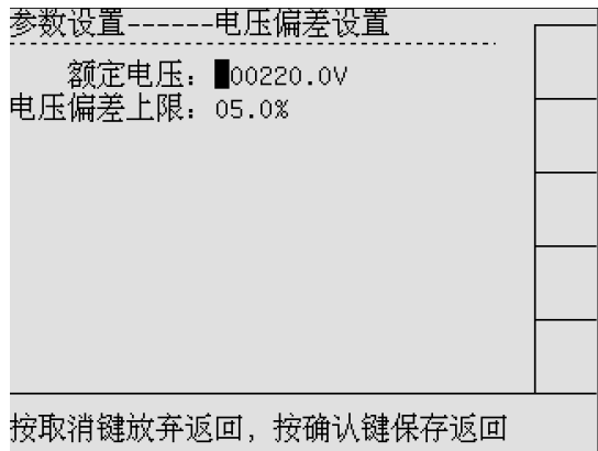
图 9-3 电压偏差屏幕——偏差设置
