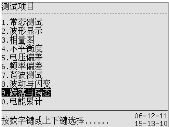
图 13-1 测试项目主菜单
