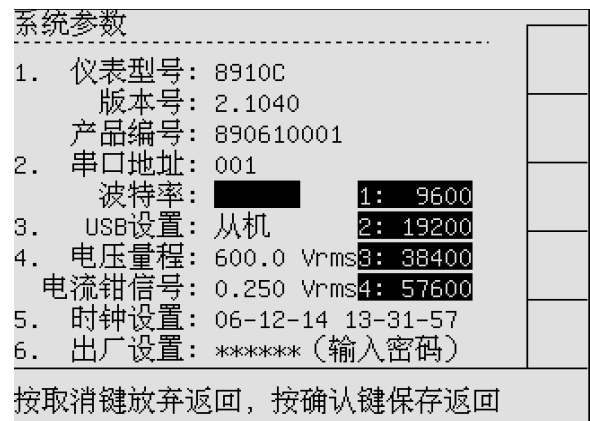
图 3-3 SYSTEM 设置—波特率
