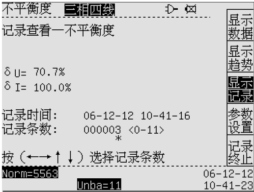
图 8-4 不平衡度—显示记录
