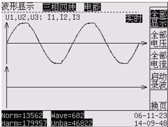
图 6-2a 波形显示屏幕（1）
