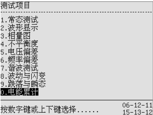
图 14-1 测试项目主菜单
