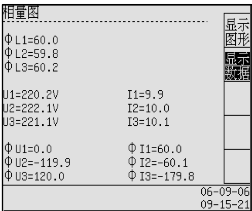
图 7-3 相量图屏幕——显示数据
