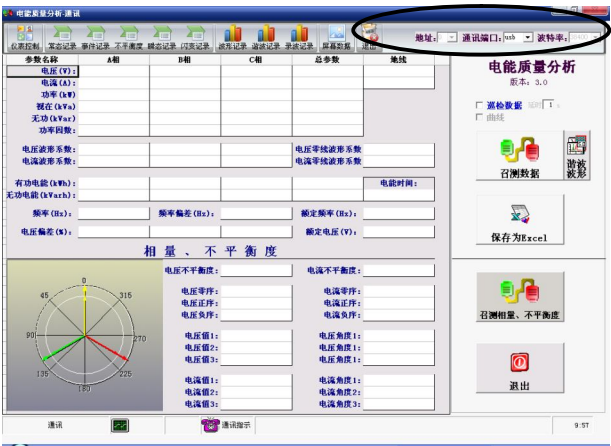
图 16-2 计算机软件界面
