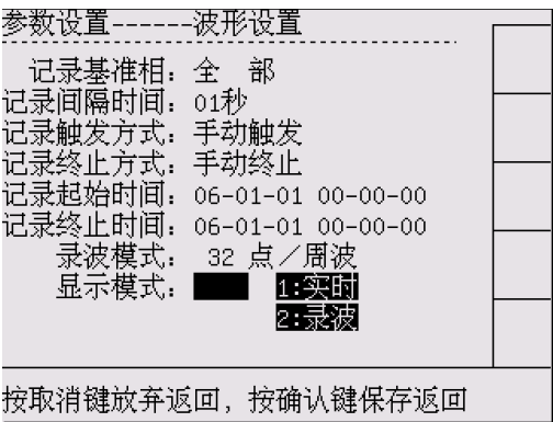
图 6-7 波形设置—显示模式
