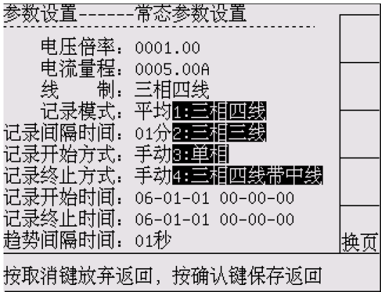
图 5-6 常态设置—线制
