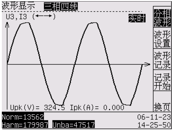
图 6-2b 波形显示屏幕（2）
