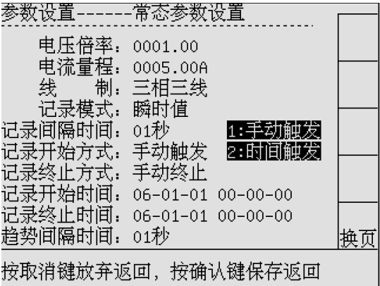
图 5-8 常态设置—记录开始
