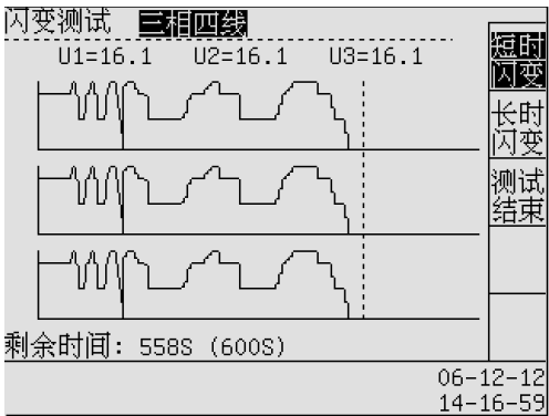
图 12-2 闪变测试屏幕——短时闪变
