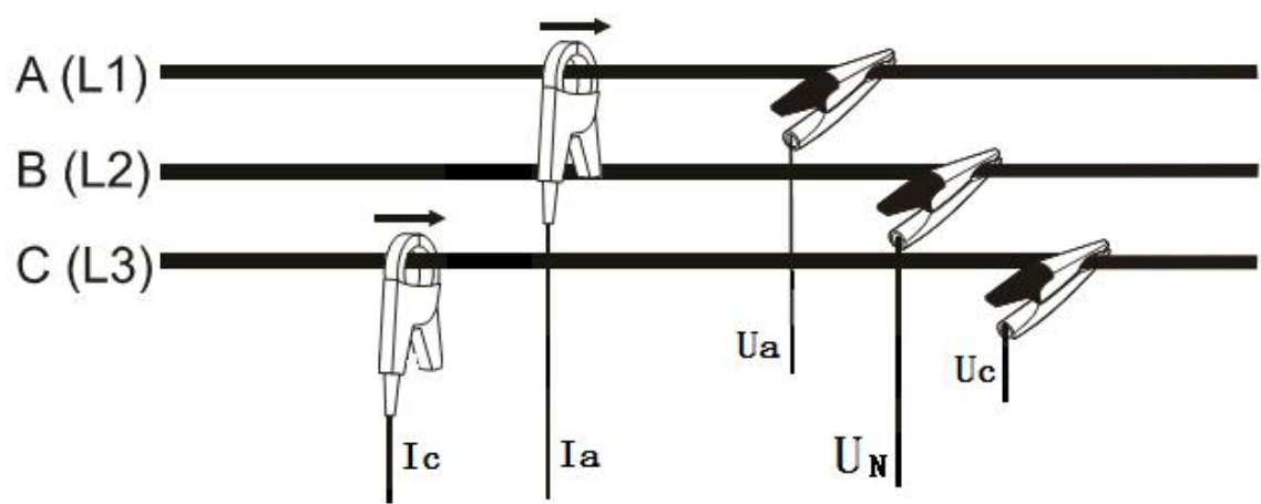
8910C 典型接线示意图——三相三线
