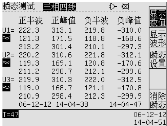
图 13-2 瞬态测试——显示数值
