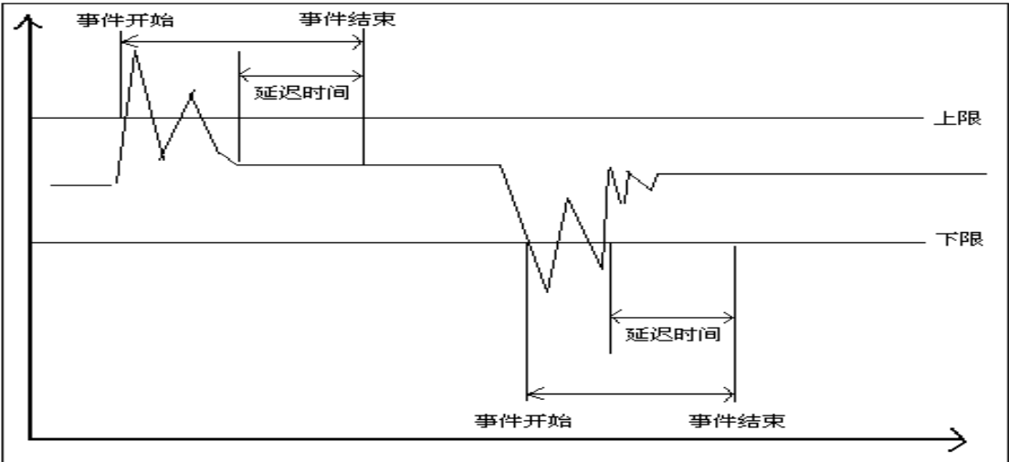
图 5-12 事件描述
