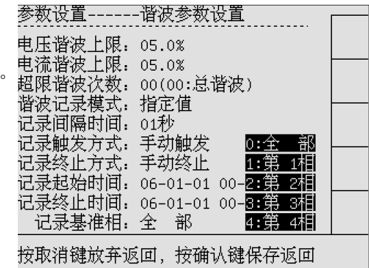
图 11-6 谐波参数—记录基准相
