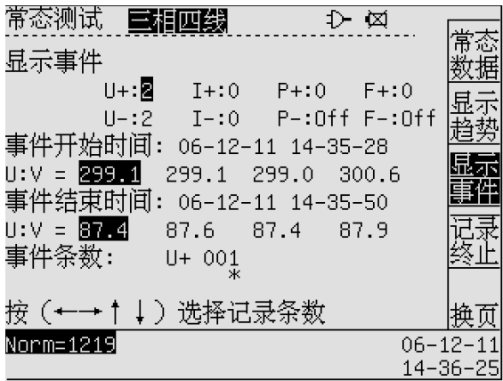
图 5-14 常态—显示事件
