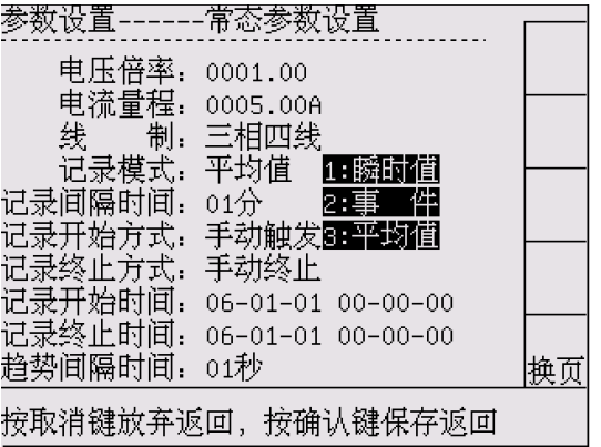
图 5-7 常态设置—记录模式
