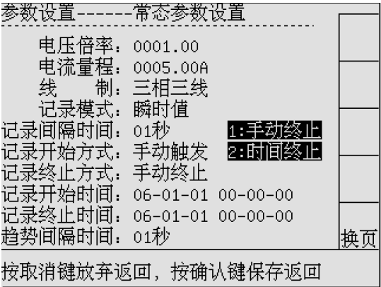
图 5-9 常态设置—记录终止
