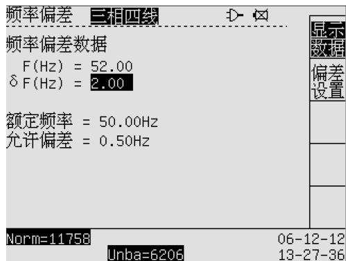
图 10-2 频率偏差屏幕——显示数据
