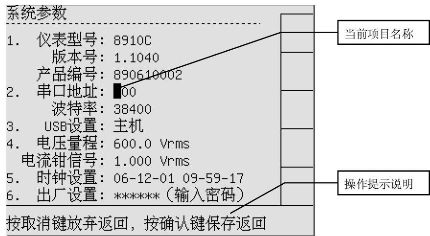
图 3-2 SYSTEM 设置
