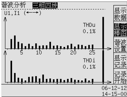
图 11-3 谐波——显示棒图
