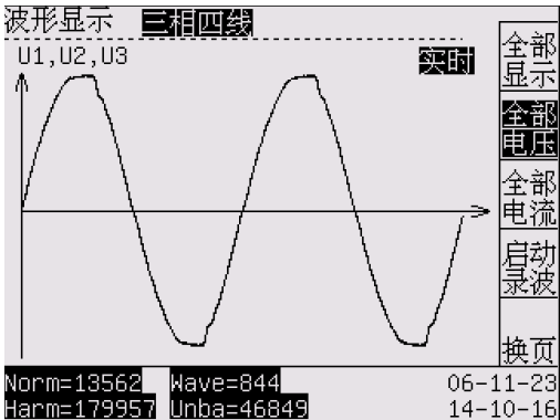
图 6-3 实时电压波形
