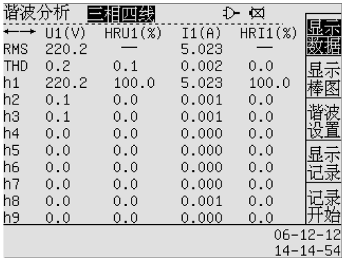
图 11-2 谐波——显示数据
