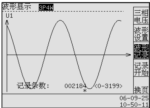
图 6-8 波形记录
