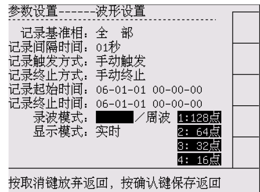
图 6-6 波形设置—录波模式
