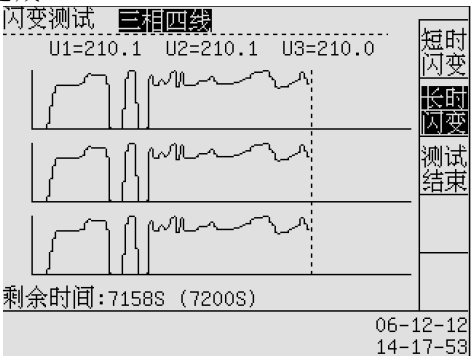
图 12-3 闪变测试屏幕——长时闪变
