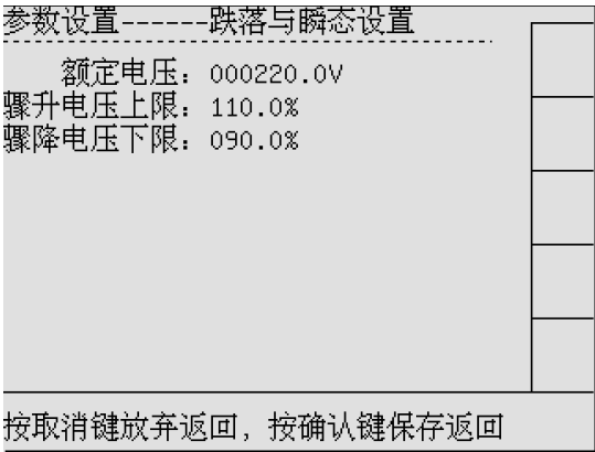
图 13-5 瞬态测试---设置
