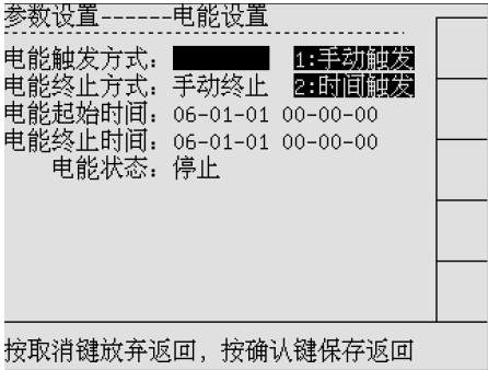
图 14-3 电能设置—触发
