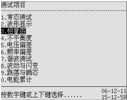
图 7-1 测试项目主菜单
