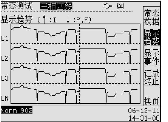
图 5-13 常态—显示趋势
