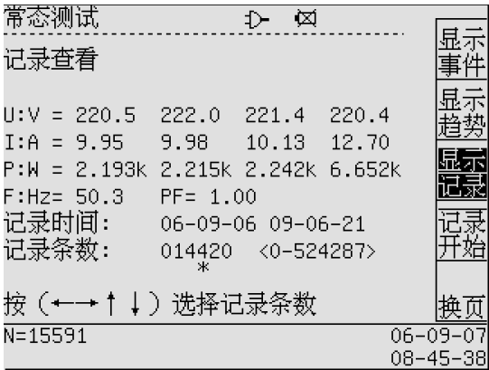
图 5-4 常态记录
