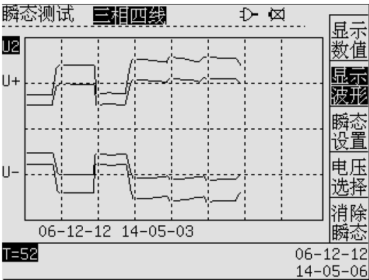
图 13-4 瞬态测试---显示波形
