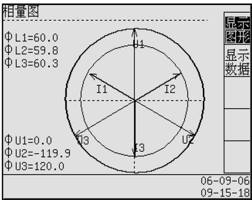
图 7-2 相量图屏幕——显示图形
