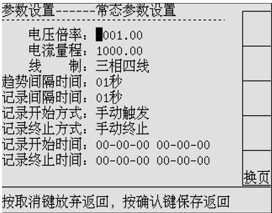
图 5-5 常态参数设置
