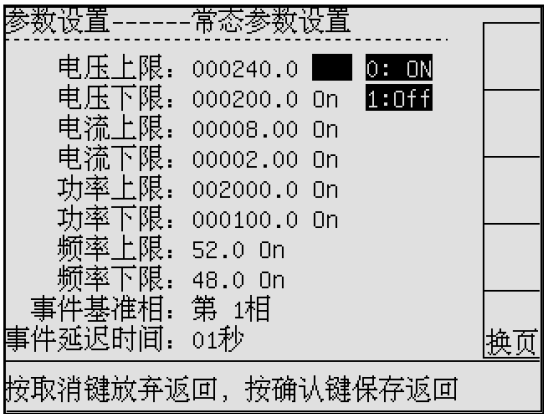
图 5-10 常态设置—极限值
