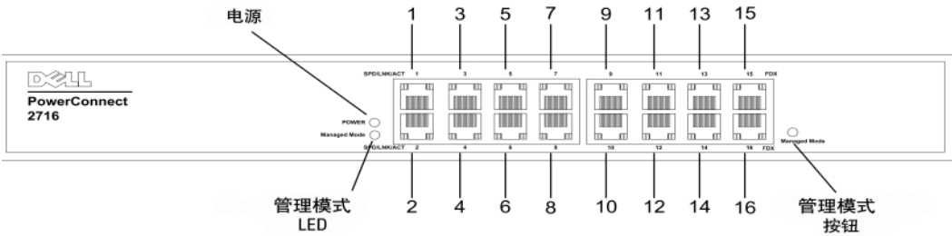
图 2-3. PowerConnect 2716 前面板
