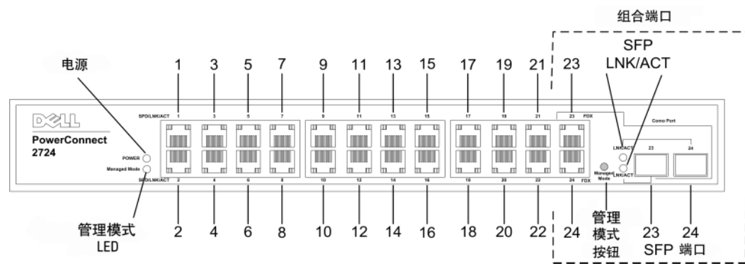
图 2-5. PowerConnect 2724 前面板
