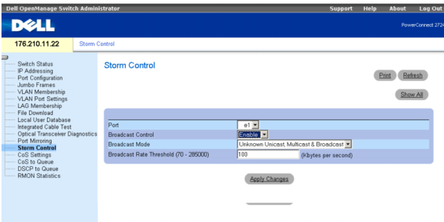
图 6-16. 风暴控制（PowerConnect 2708 配置）
