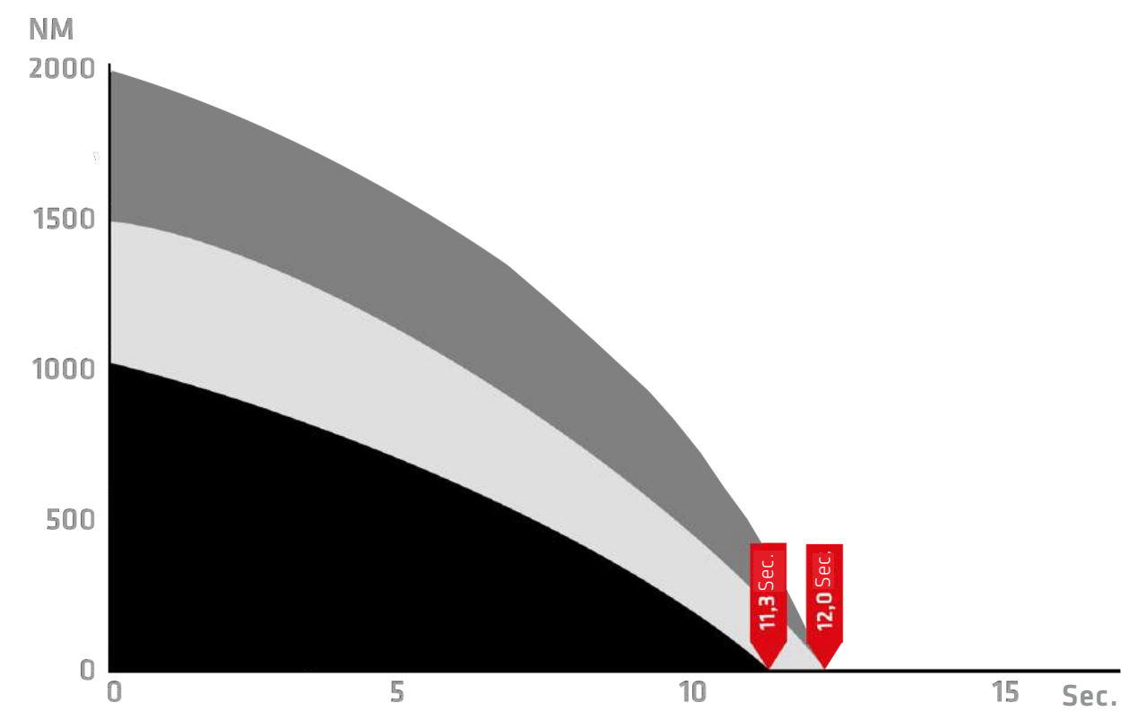
Luzowanie: Porównanie krzywej momentu
