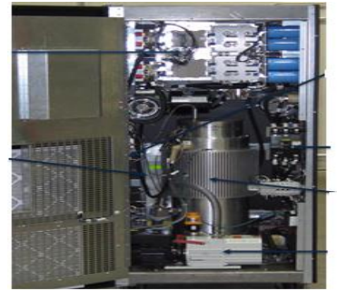
飞轮储能
