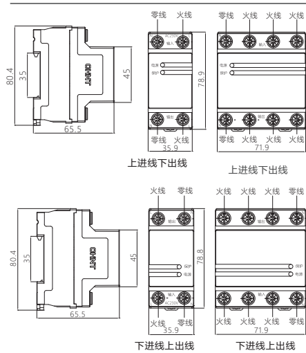
图1 OUVR-1自恢复式过欠压保护器外形与安装尺寸图
