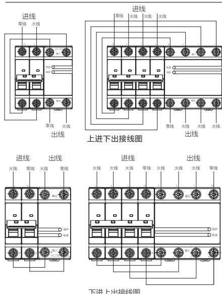
图2 OUVR-1自恢复式过欠压保护器进出线方式图
