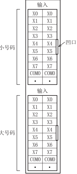
FX5-C32EX/DS
