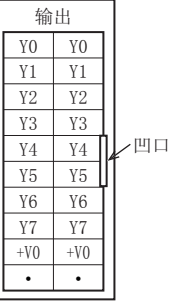
FX5-C16EYT/DSS
