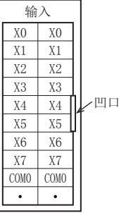
FX5-C16EX/DS
