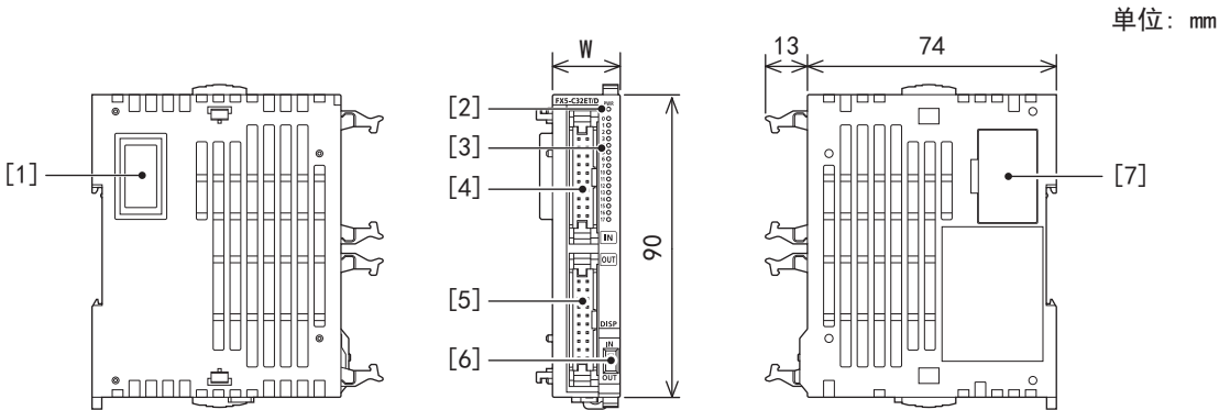
外形尺寸
