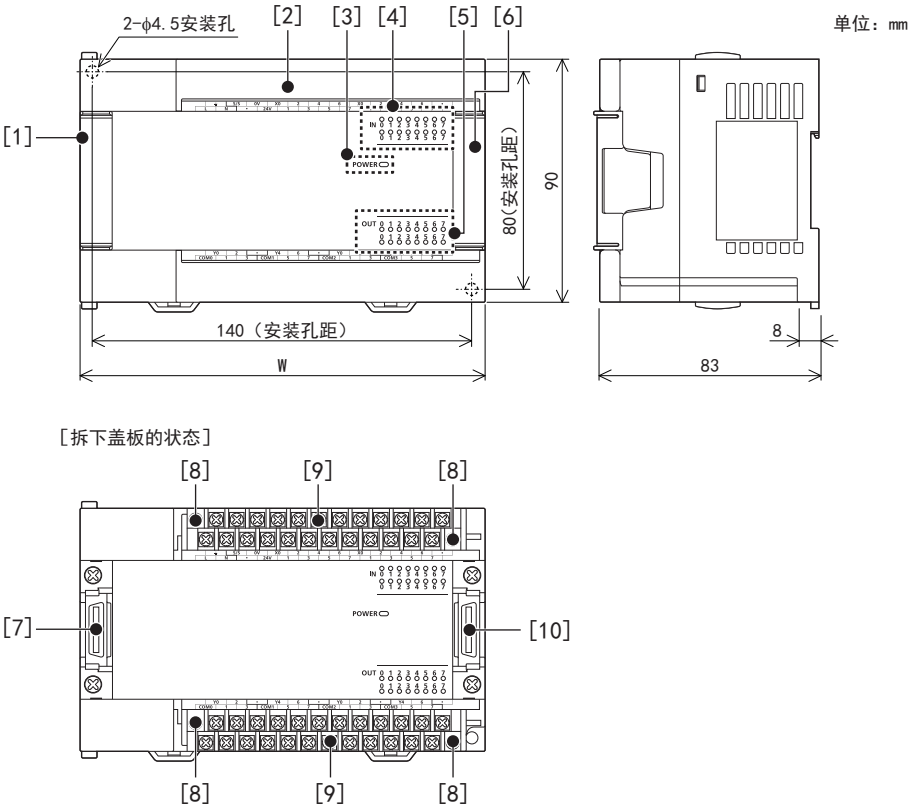
外形尺寸
