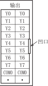
FX5-C16EYT/D
