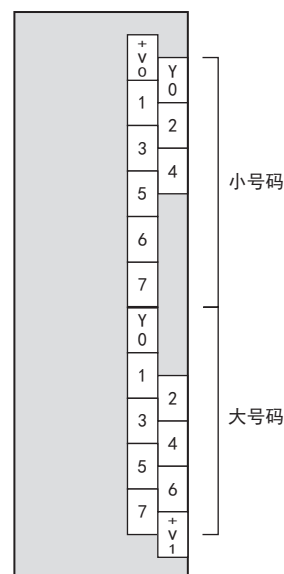
FX5-16EYT/ESS
