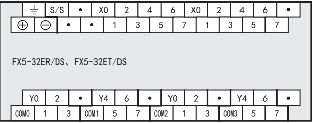
FX5-32E□/D□
