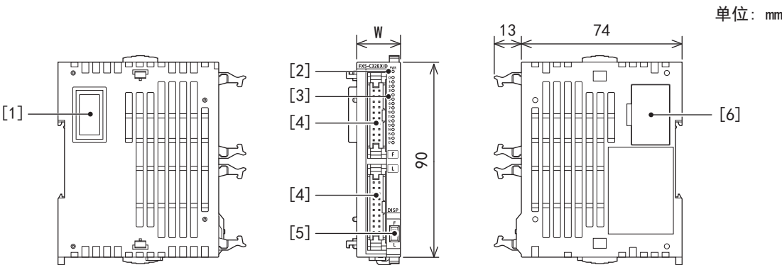
外形尺寸
