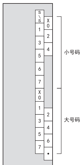
FX5-16EX/ES
