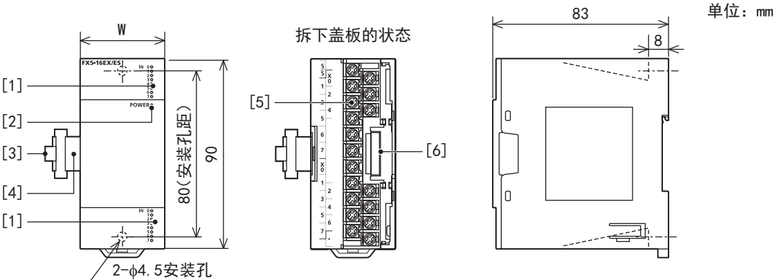
外形尺寸
