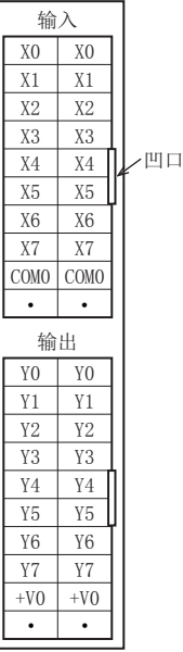
FX5-C32ET/DSS
