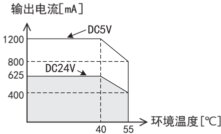
■FX5-C1PS-5V的情况下
