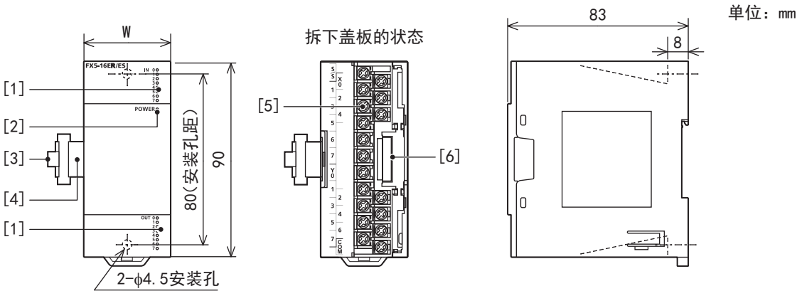
外形尺寸
