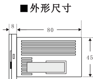
侧面图
