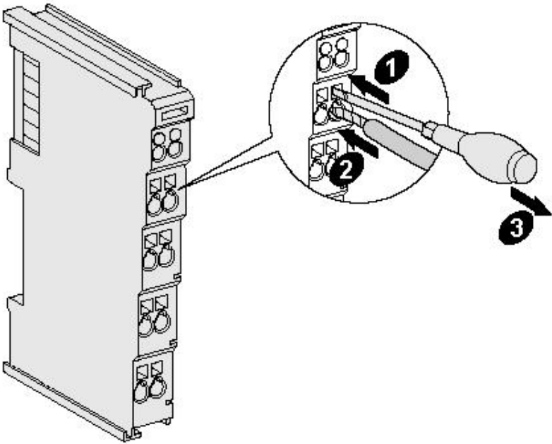
图2.2 GC-4662模块安装
