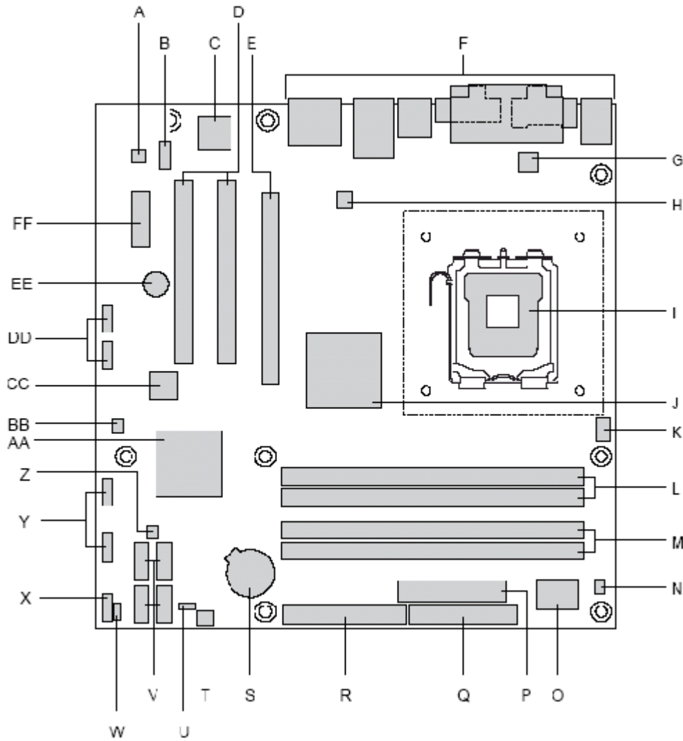
附1 美仑3400E 1100工作站主板结构说明
