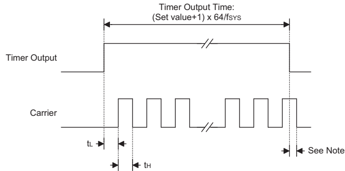
载波输出时定时器的输出
