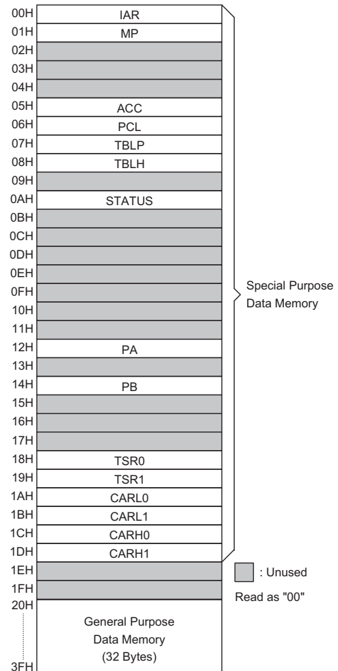
数据存储器
