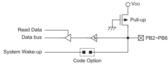
PB2~PB6 输入口
