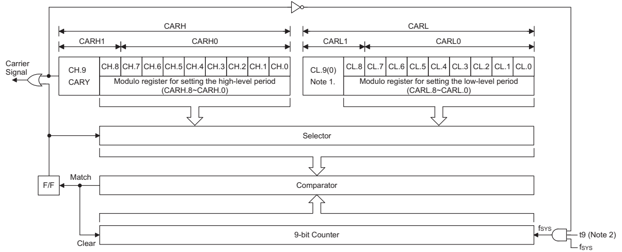
遥控器载波发生器的结构
