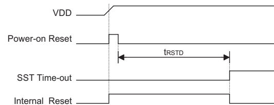
复位时序图
