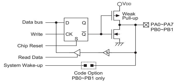
PA, PB0~PB1 输入/输出口
