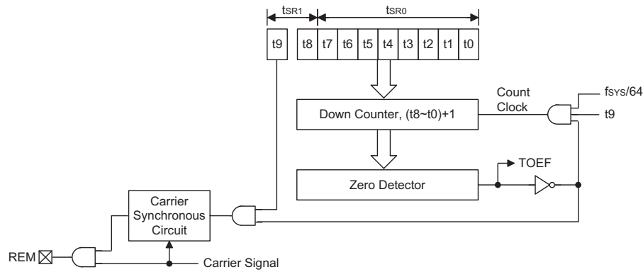
定时器结构
