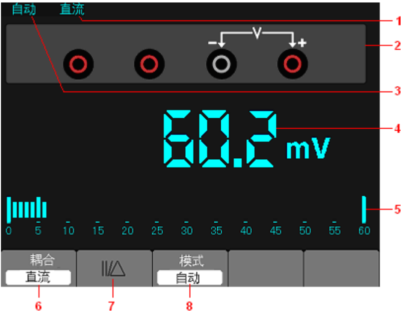
图4-1万用表界面
