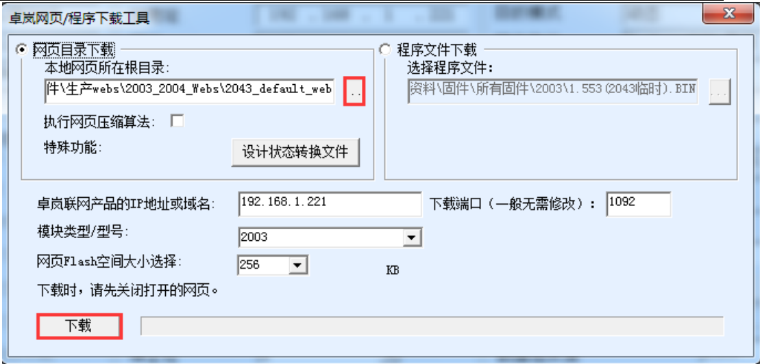
图 52 ZLSN2003 web 升级方法
