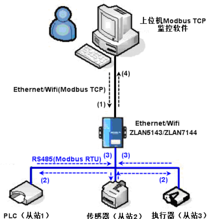
图 35 存储型 Modbus 网关工作方式
