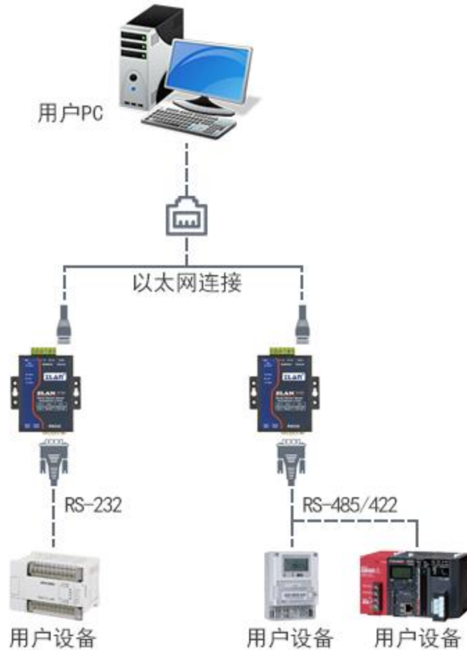
图 2 连接示意图
