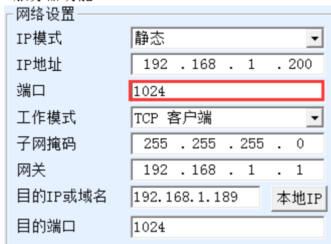
图 25 既做客户端也做服务器
