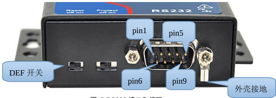
图 5 RS232 接口和拨码
