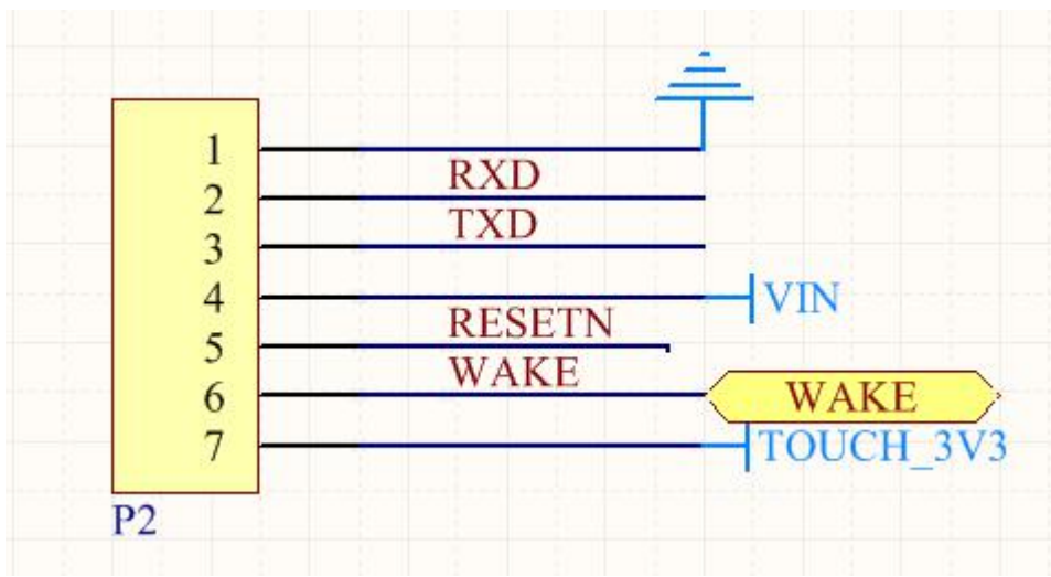
图 3-3 BFM563A 串口接口(P2)
