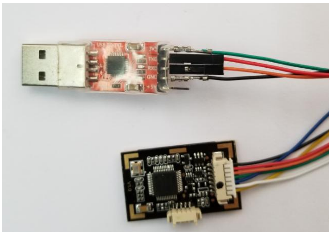
图 4- 3 串口通信方式连接图
