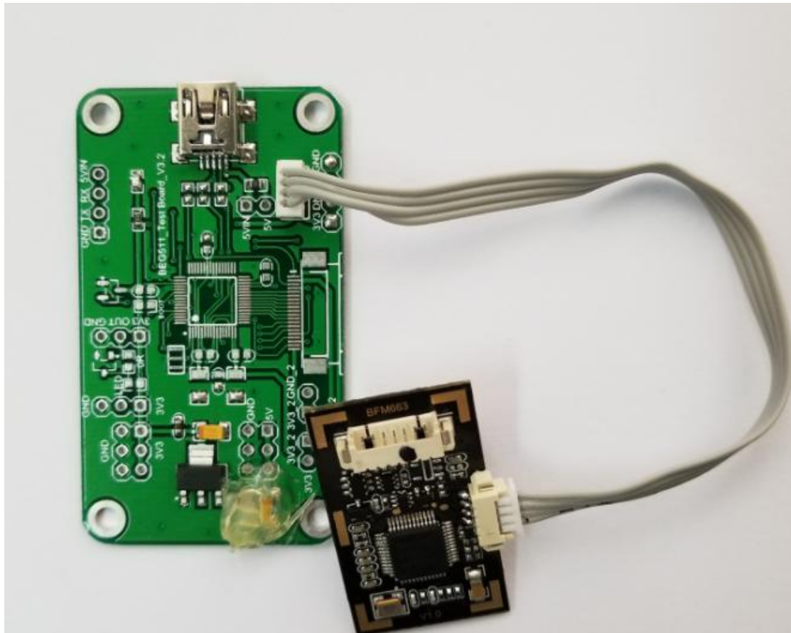
图 4-1 USB 通信方式连接图
