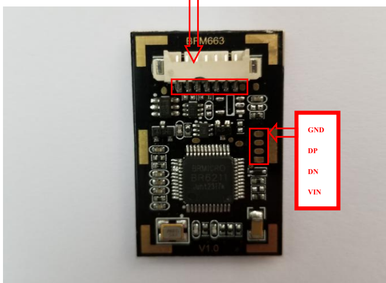
图 3-2 BFM563A 模块图反面
