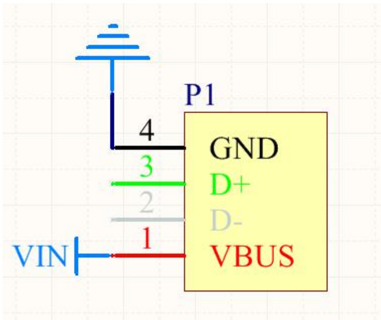
图 3-4 BFM563A USB 接口(P1)
