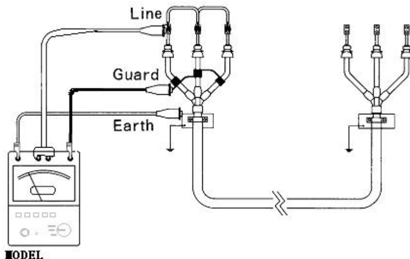
电缆芯对表皮绝缘测试图示 (由此图示可变化电缆芯对芯的绝缘)
