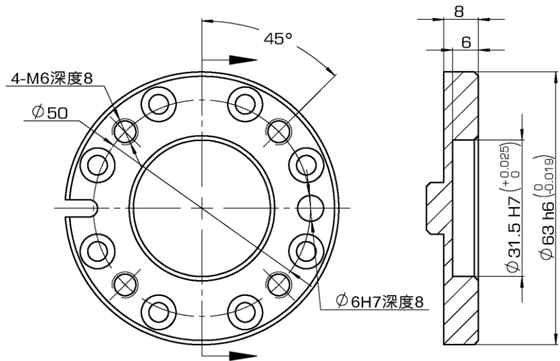
图 6-7 AIR7-920B 型操作机腕部法兰尺寸示意图
