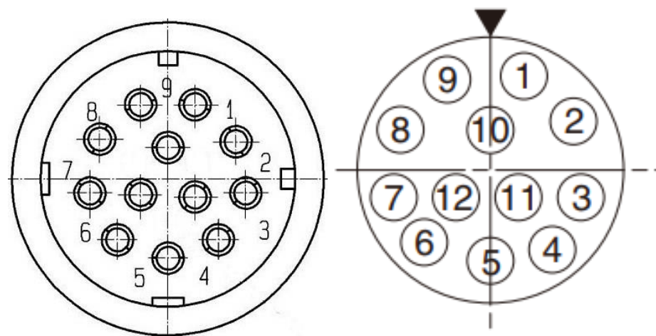
图 4-4 AIR7-920B 型操作机小臂 IO 接口
