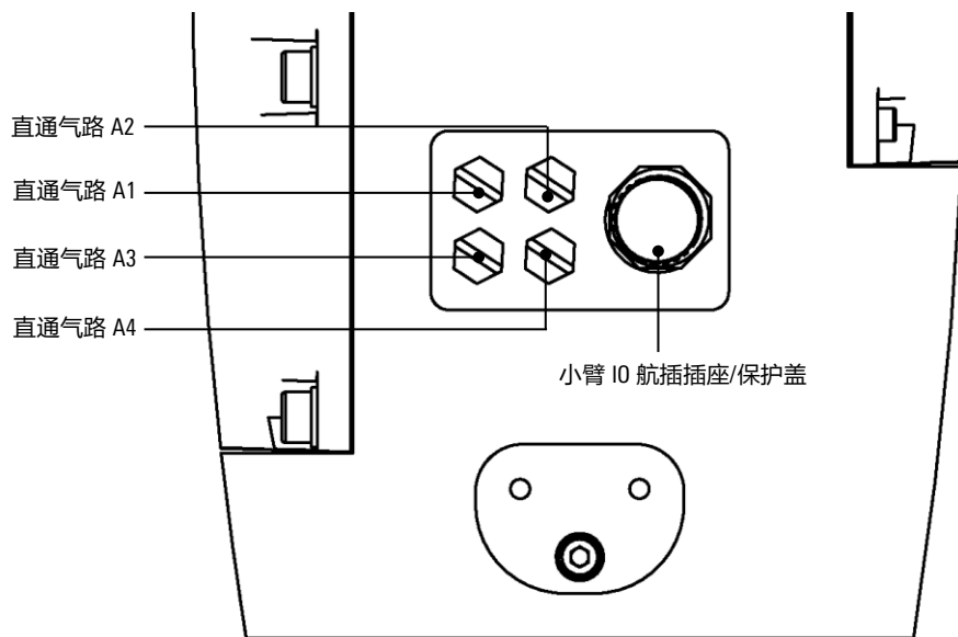
图 4-2 AIR7-920B 型操作机小臂上接口
