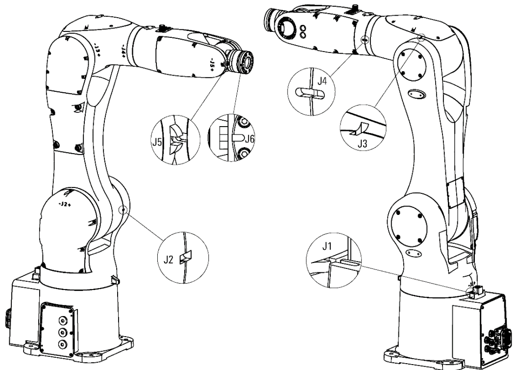
图 6-3 AIR7-920B 各轴零点示意图
