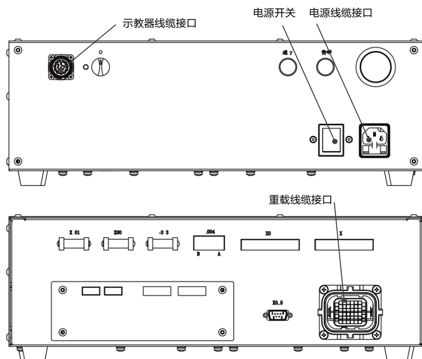
图 5-4 AIR7-920B 控制柜示意图
