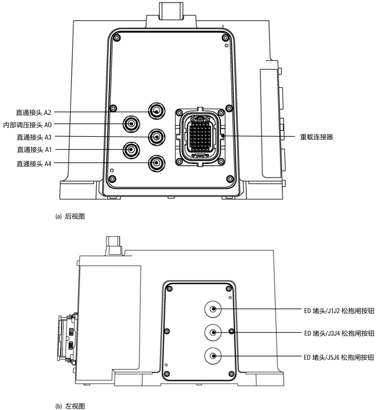
图 4-1 AIR7-920B 操作机本体底座接口
