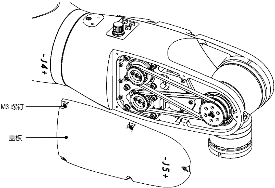
图 9-5 拆卸盖板
