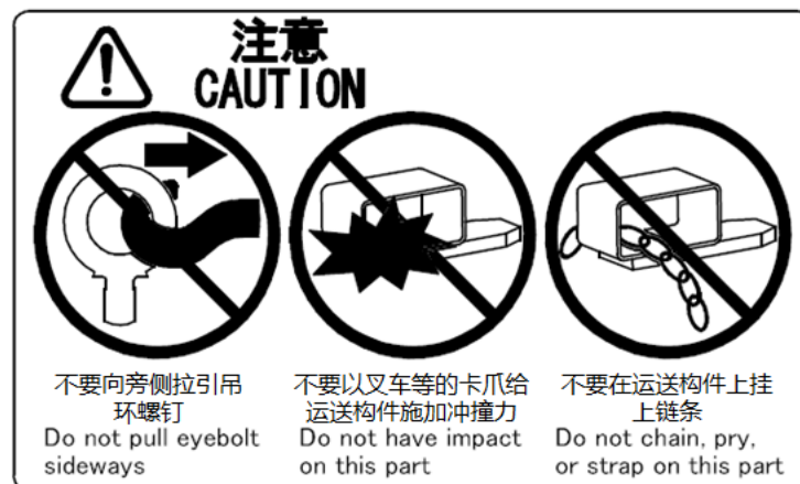
图 3-2 操作机在搬运过程中的注意事项
