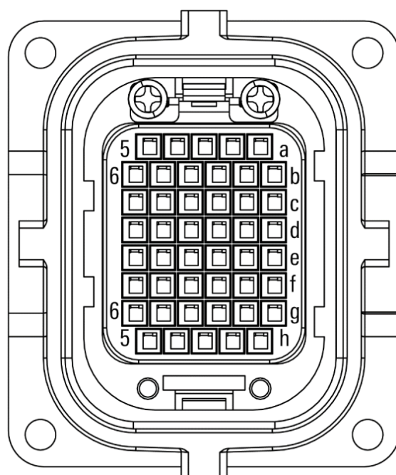
图 4-3 AIR7-920B 型操作机重载接口
