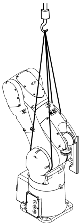
图 3-6 AIR7-920B 吊环搬运示意图
