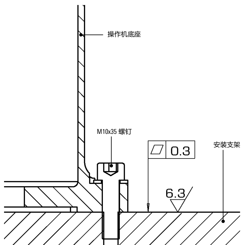
(b) 剖面图
