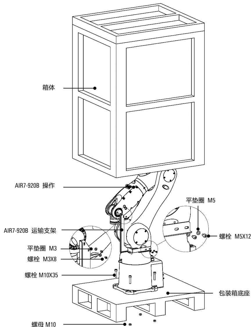
图 3-1 操作机包装示意图
