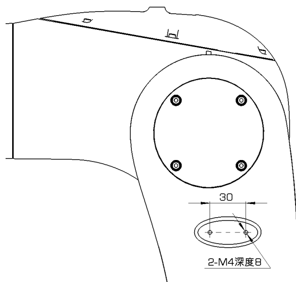
图 6-12 AIR7-920B 大臂接口尺寸图
