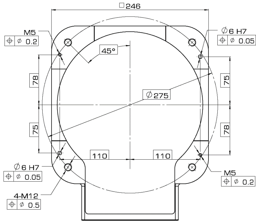
图 3-7 AIR7-920B 型操作机基座接口尺寸
