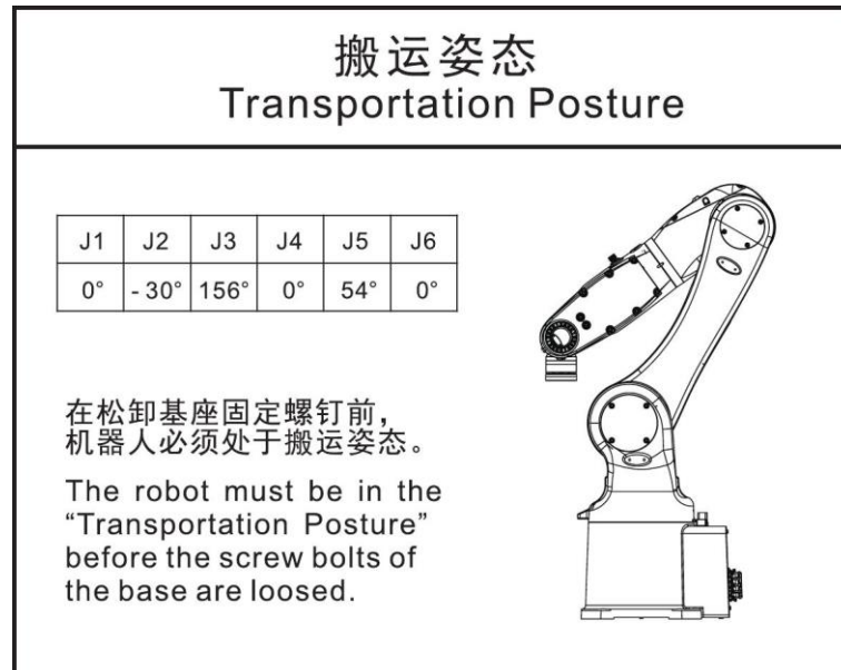
图 2-5 AIR7-920B 操作机搬运姿态标签
