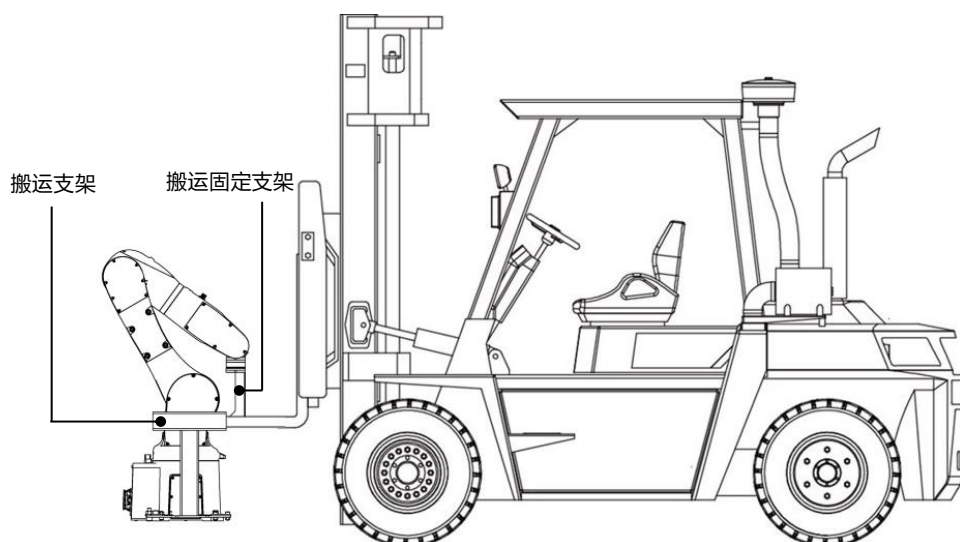
图 3-5 AIR7-920B 叉车搬运示意图
