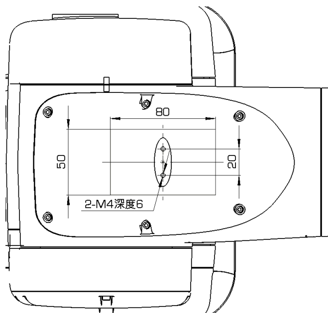
图 6-10 AIR7-920B 型操作机肘部负载接口尺寸示意图
