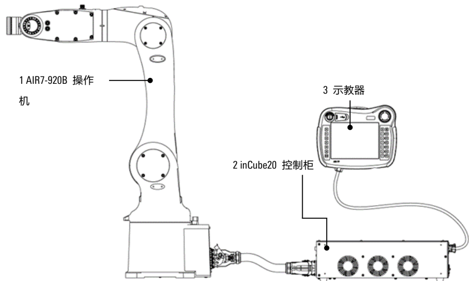
图 2-1 AIR7-920B 工业机器人系统的构成
