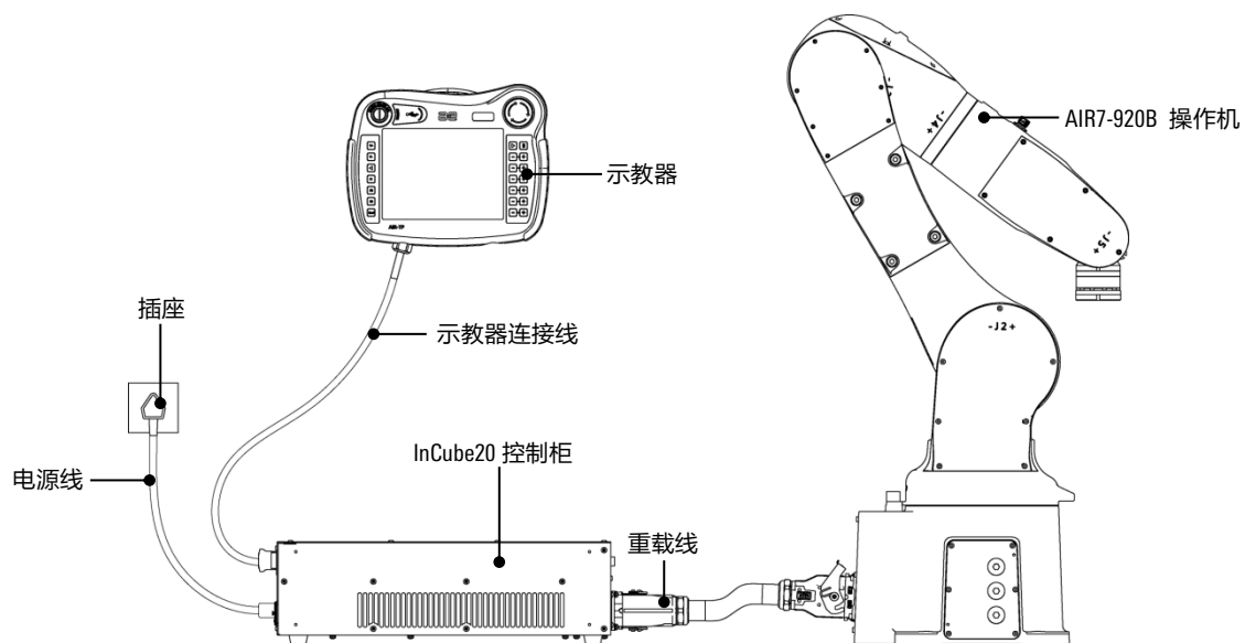
图 5-8 AIR7-920B 工业机器人系统接线概览
