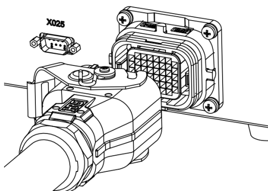
图 5-7 控制柜重载连接器接口
