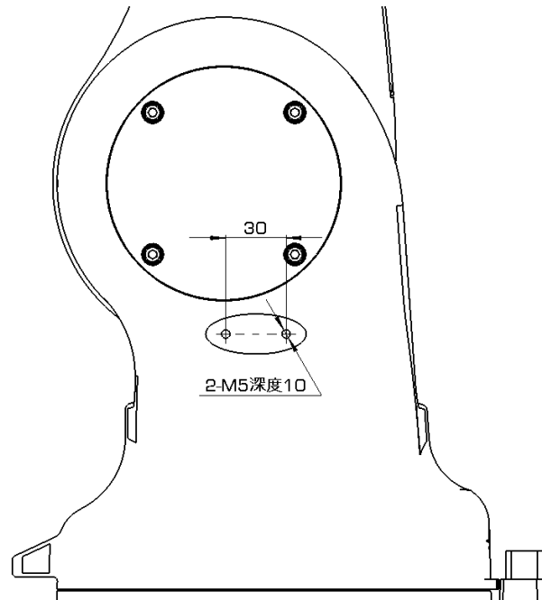
图 6-13 AIR7-920B J1 轴本体接口尺寸图
