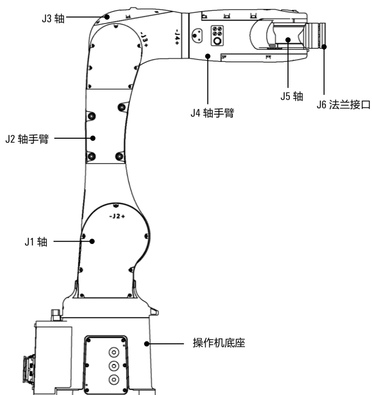
图 2-2 AIR7-920B 型机器人本体及其各个部分
